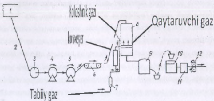
Temir rudalardan po'latlarni do'mnasiz olish usulining texnologik sxemasi
