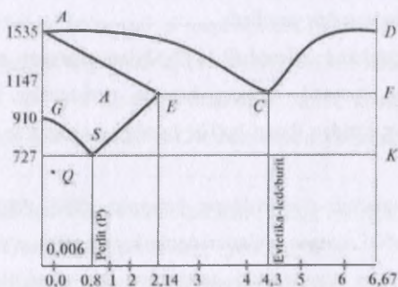
5.8-rasm Temir — uglerod qotishmalarining holat diagrammasi.
