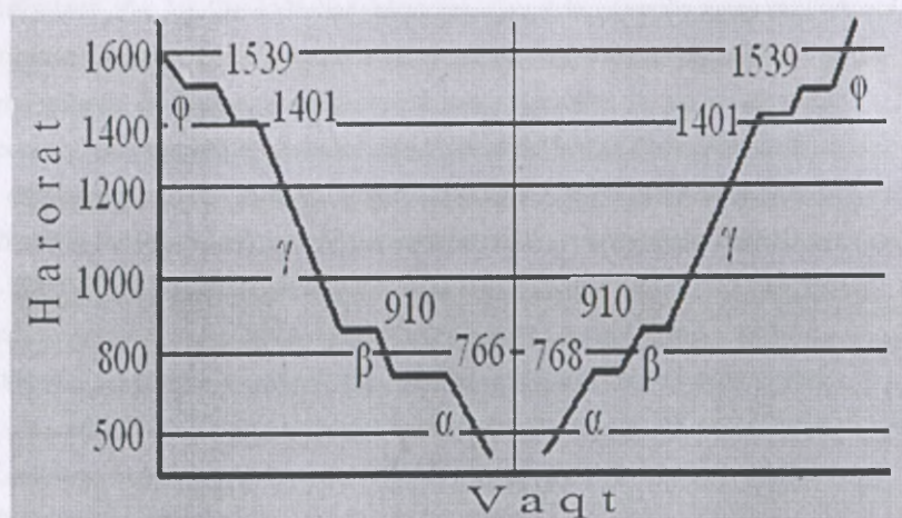
8.1rasm. Temirning sovish va erish grafigi
