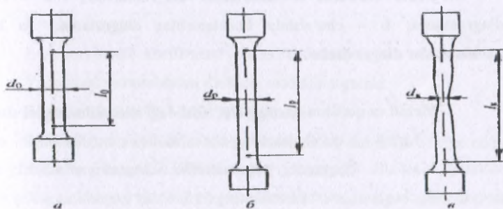
7.2- Rasm. Silindrik namunaning har xil bosqichlaridagi cho'zilish sxemasi:
