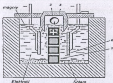
13.5-rasm. Magniy xloridni elektroliz qilish vannasi sektsiyasining sxemasi. 1-anod; 2-katod plastinkasi; 3-to'siq; 4-xlorni chiqarish trubasi.
