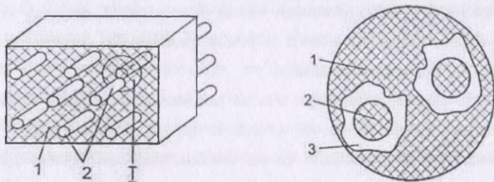
18.1-rasm. Kompozitsion materiallarning tuzilishini tushuntiruvchi chizma: 1 – matritsa (bog'lovchi material); 2 – armatura (mustahkamlovchi) element;
