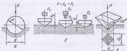
6.10-rasm. Qattqlikni o'lchash: a) Brinel usuli b) Rokvell usuli v) Vickers usuli
