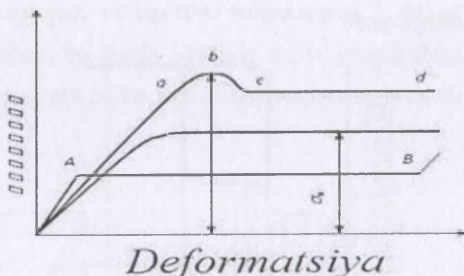
16.3-rasm. Shishasimon (yuqori va pastdagi) hamda kristall strukturali (o'rtadagi) polimerlarning "deformatsiya- kuchlanish" grafigi.
