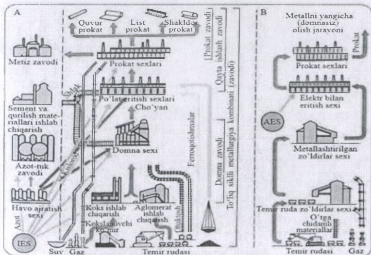
6-rasm. Metallurgiya kombinatidagi sexlar sxemasi
