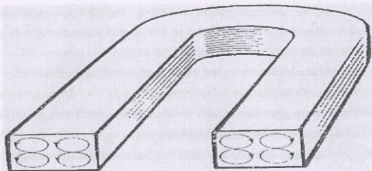
chizma – Elektronlarning xususiy momenti mavjudligini isbotlovchi Shtern va Gerlax tajribalari;
