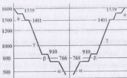
5.7-rasm Temirning sovish va erish grafigi.
