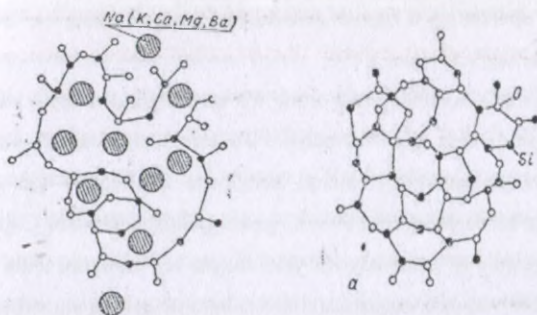
14.2-rasm. Anorganik shishalarning strukturasi:
