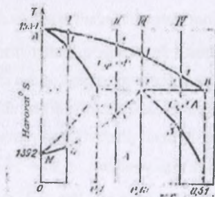
8.6-rasm. Temir-uglerod sistemasining holat diagrammasining umumiy ko'rinishi peritektik qismi
