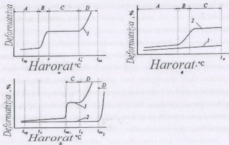
16.7-rasm. Termomexanik grafiklar:
