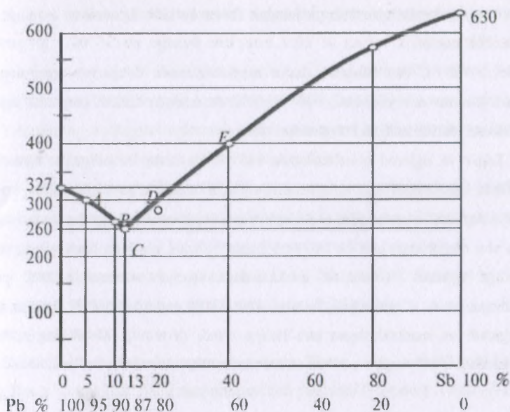
5.6-rasm. Qotishmalarning holat diagrammasi.
