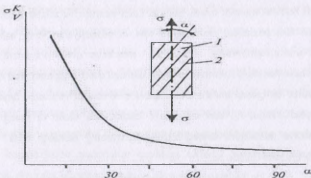
18.3-rasm. Bir tomonga yoʻnalgan toʻliq kompozit mustahkamligining toʻla yoʻnalish burchagiga qarab oʻzgarishi: 1 — matritsa; 2 — toʻla
