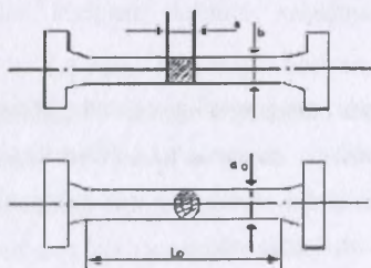
6.7-rasm. Tajriba uchun ishlatiladigan namunalarning sxematik tuzilishi
