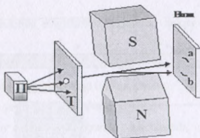
chizma – Elektronlarning xususiy momenti mavjudligini isbotlovchi Shtern va Gerlax tajribalari;
