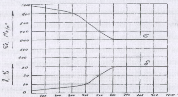
7.5-rasm. Qizdirib bosim bilan ishlash haroratiga ko'ra metall xossalarini o'zgarish sxemasi
