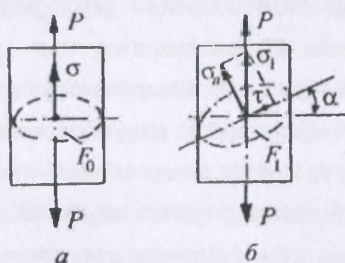
1.3- rasm. Normal va urinma kuchlanishlar sxemasi.
