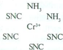
sis-izomer
