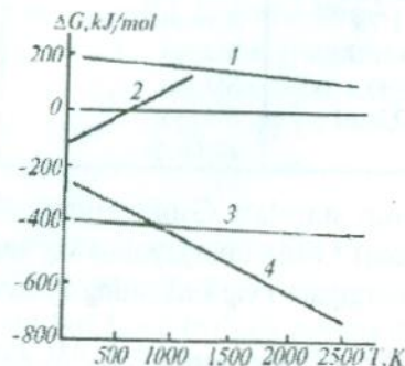
2-rasm. Kimyoviy reaksiyalarning izobar izotermik potensialining haroratga bog'liqligi:
