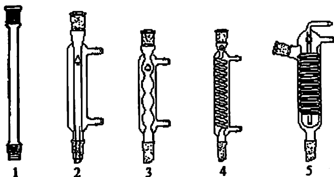
4-rasm: 1 – havo sovutgichi; 2 – Libix sovutgichi; 3 – sharikli sovutgich; 4,5 – spiralli sovutgichlar
