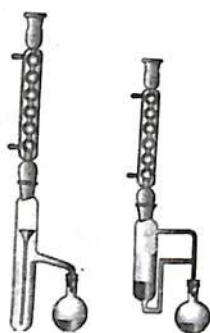
13-rasm. Eritmani to'xtovsiz ekstraksiya qilish asboblari
