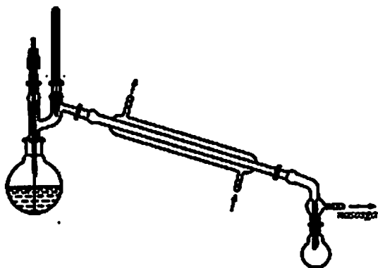
12-rasm. Moddalarni vakuumda haydash asbobi
