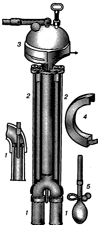
Рис. 2.6. Психрометр Асмана:
