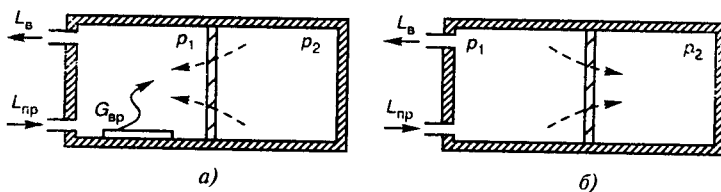
Рис. 2.2. Принципиальная схема вентиляции для выбора соотношения объемов приточного и удаляемого воздуха:
