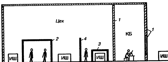
Рис. 7.19. Средства звукоизоляции:
