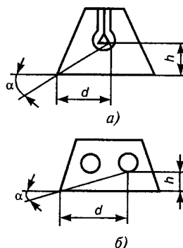
Рис. 2.9. Защитный угол светильника:
