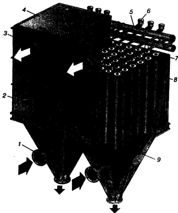
Рис. 7.41. Рукавный фильтр:
