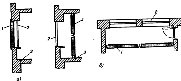
Рис. 7.29. Установка сотовых решенок на окна:
