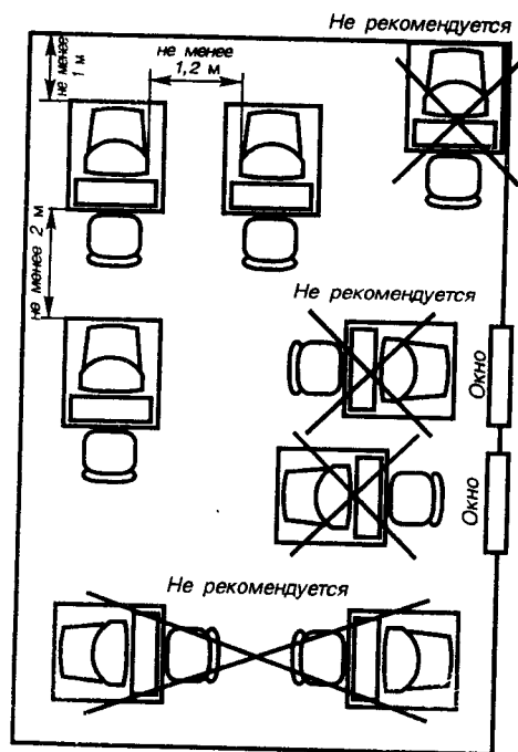
Рис. 7.35. Расположение компьютеров в помещении
