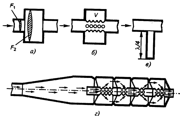
Рис. 7.23. Реактивные глушители:
