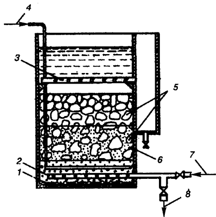
Рис. 7.53. Каркасно-засыпной фильтр:
