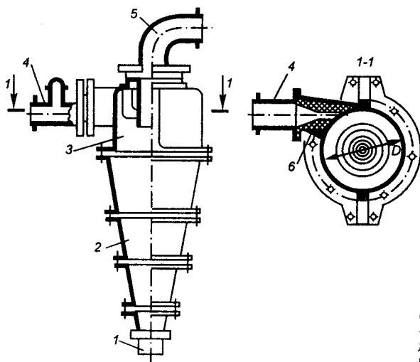
Рис. 7.52. Напорный гидроциклон:
