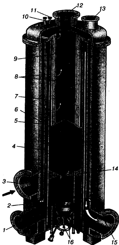
Рис. 7.49. Каталитический реактор:
