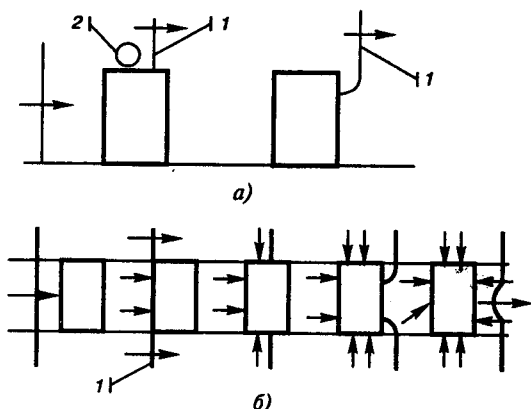
Рис. 9.3. Взаимодействие воздушной ударной волны с плоским препятствием:
