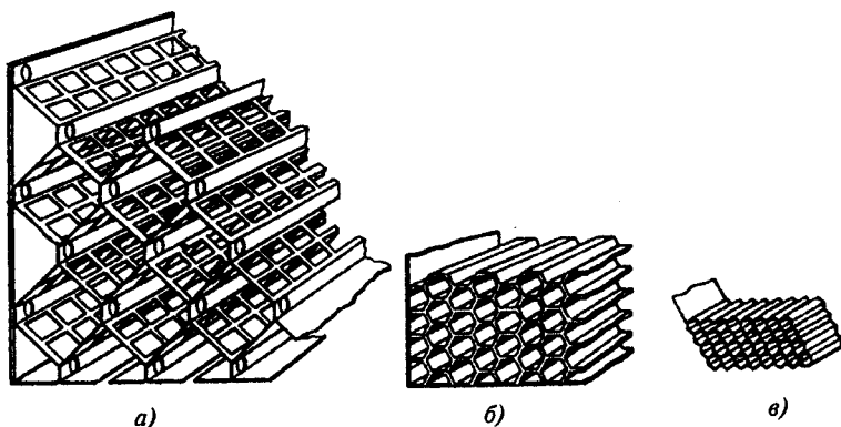
Рис. 7.28. Сотовые решетки, применяемые для экранирования ЭМП в частотных диапазонах:
