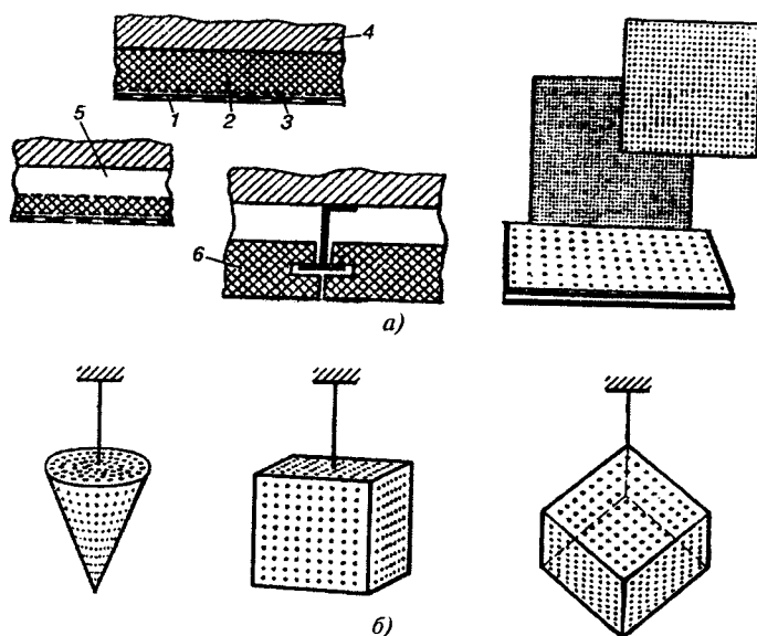
Рис. 7.18. Акустическая обработка помещений:
