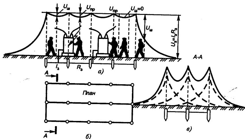
Рис. 7.7. Контурное заземление:
