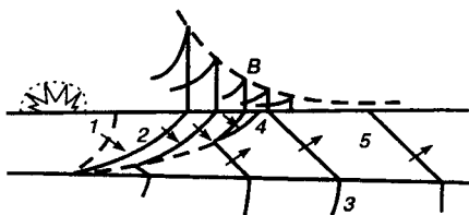
Рис. 9.2. Волновая картина при наземном взрыве
