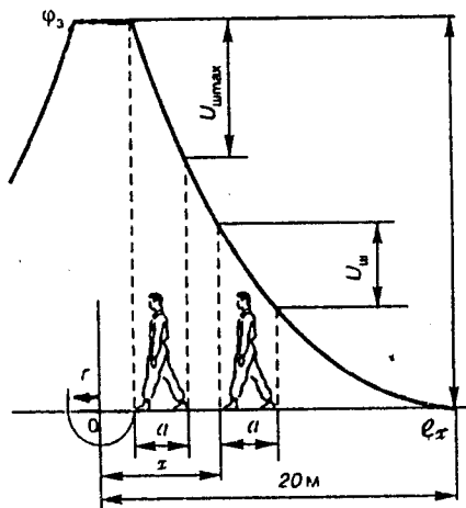
Рис. 7.4. Напряжение шага
