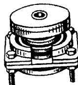
Рис. 7.15. Виброизолирующие опоры:
