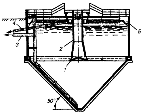
Рис. 7.51. Вертикальный отстойник из сборного железобетона:
