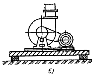
Рис. 7.14. Установка агрегатов на виброгасящем основании: а — на фундаменте и грунте; б — на перекрытии
