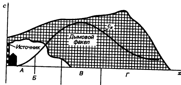
Рис. 5.1. Распределение концентрации вредных веществ в атмосфере у земной поверхности от организованного высокого источника выбросов:
