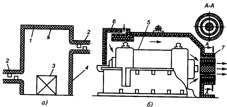
Рис. 7.20. Звукоизолирующий кожух:
