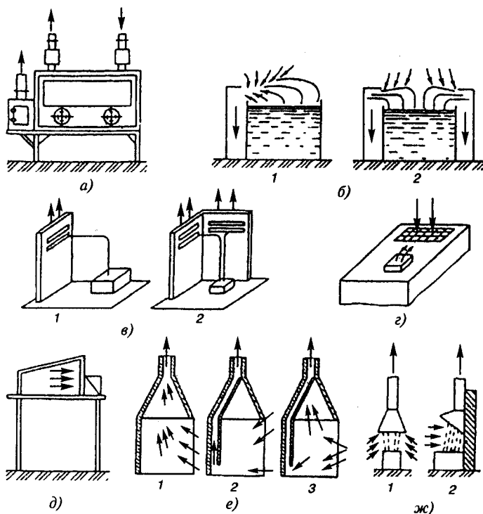
Рис. 2.4. Устройства местной вентиляции:
