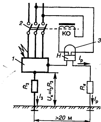
Рис. 7.12. Принципиальная схема устройства УЗО:
