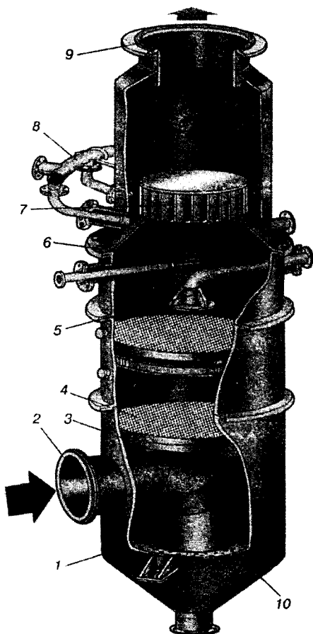
Рис. 7.45. Пенный аппарат:
