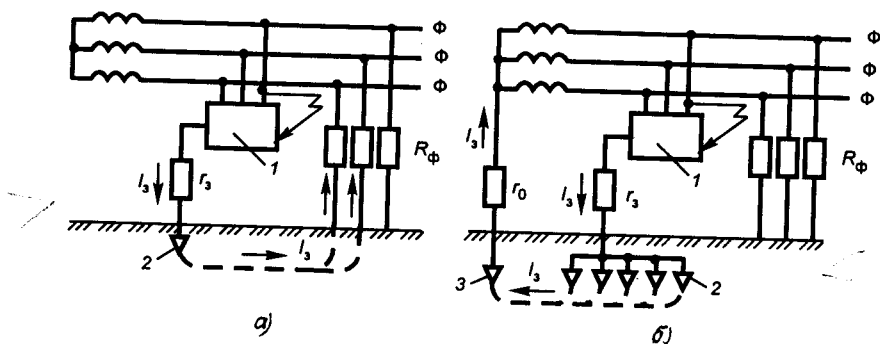
Рис. 7.5. Принципиальные схемы защитного заземления
