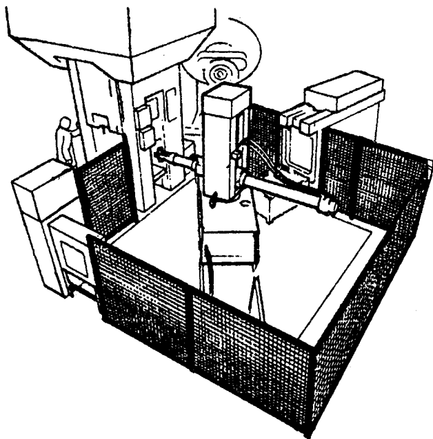
Рис. 7.1. Стационарное сетчатое ограждение промышленного робота
