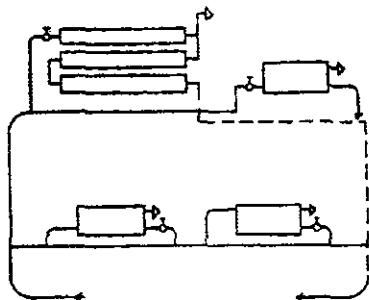
4.4.1-rasm. Pastdan issiqlik uzatuvchi gorizontaal ko'rinishli isitish tarmog'i: a-ikki quvurli; b-bir quvurli.
