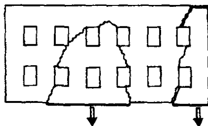
3.7.3-rasm. Binoning o'rta va chekka qismlarining cho'kishi.
