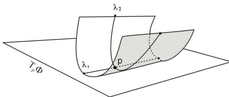
Parabolik nuqta
