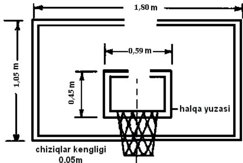
2-rasm. Shit. Uning o'lchovlari.
