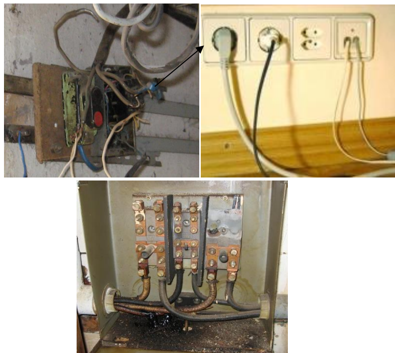
Электр қурилмаларининг улаш (контакт) жойлари мустаҳкам бажарилмаганлиги.
