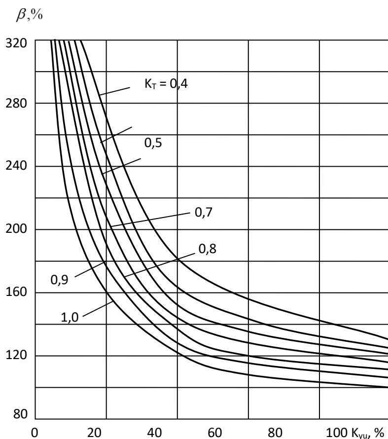
2 – rasm. Ishchi mashinada sarflanayotgan elektr enyergiya solishtirma qiymatining yuklanish koefitsiyentiga bog`liqlik grafigi
