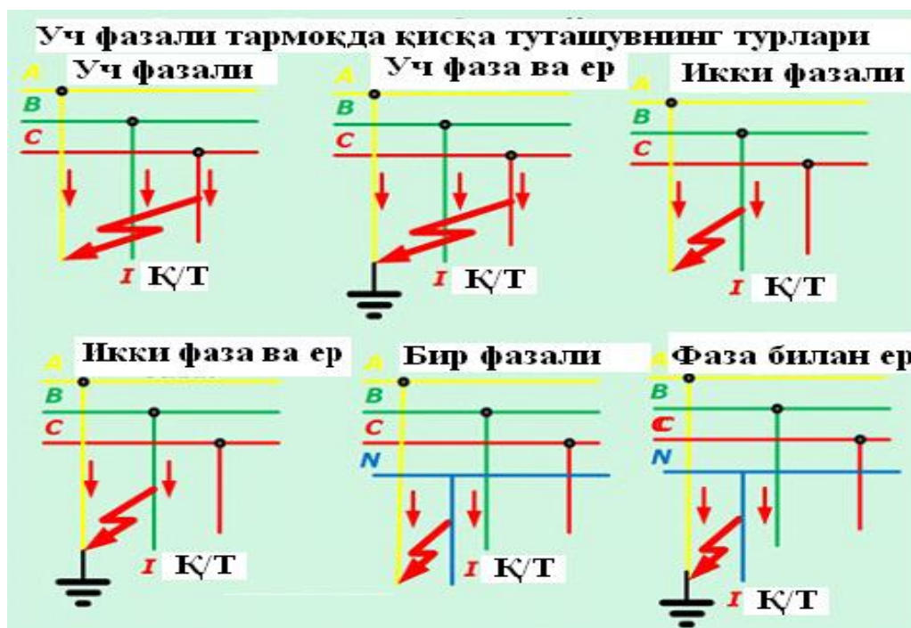
Қисқа туташувнинг турлари.
