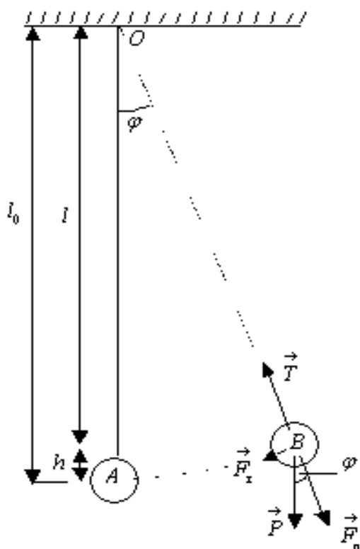
Rasm 1. Eksperimental qurilmaning tasviri
