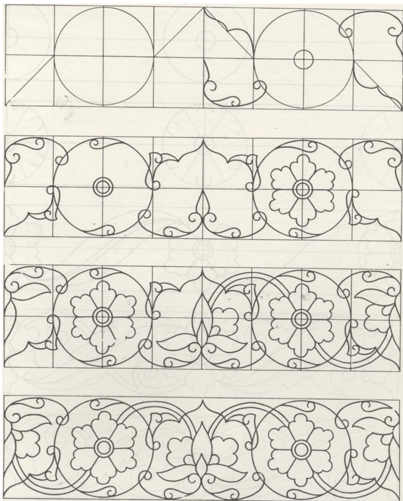
30-rasm. 5-gul. «Aylana shukuftali islamiy» naqsh namunasini chizish bosqichi
