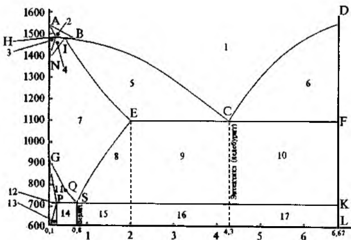
X11.5-расм. Fe — C системанинг >олаг диаграммаси.
