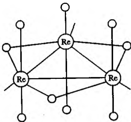
X11.2-расм. [Ке3C!^'] - анионининг фазовий тузилиши.
