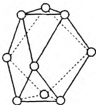
Х1.7-расм. [\text{Bi}_6]^{5+} катиони тригонал призмасининг тузилиши.
