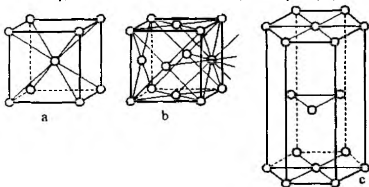
VIII.2-расм. Металллар кристалл панжараларининг асосий турлари.
