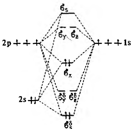
V.4-расм. Аммиак молекуласининг соддалаштирилган молекуляр орбиталар диаграммаси.
