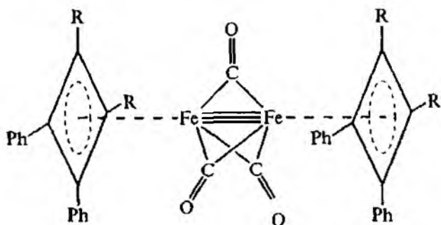
XI.3-расм. 1, 2 ва 3 та боғ воситида боғланган икки ўзакли бирикмалар.
