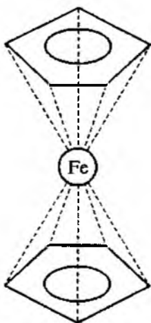
X11.8-расм. Ферроцен молекуласининг тузилиши.
