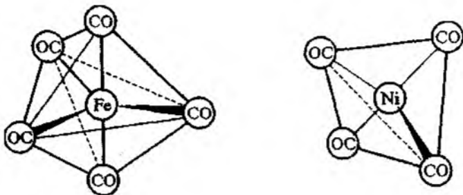
Х11.6-расм. \text{Fe(CO)}_5 ва \text{Ni(CO)}_4 ларнинг тузилиши.
