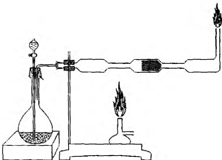
V.5-расм. Жуда оз миқдорда мишьяк бирикмаларини тутган намунани анализ қилиш усуласи.
