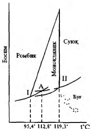
IV.1-расм. Олтингугуртнинг ҳолат диаграммаси.
