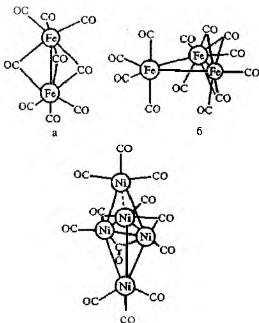
XII.7-расм. \text{Fe}_2(\text{CO})_9 , (а), \text{Fe}_3(\text{CO})_{12} , (б) ва \{m, (\text{CO})_n\} -карбонилларнинг тузилиши.
