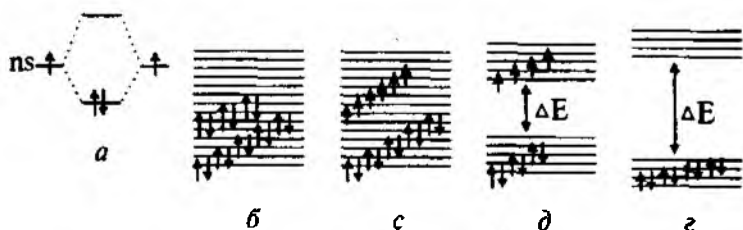
VIII.1-рasm. Metallar, metallmaslar va yarimutkazgichlarda energetik zonalarning joylashish sxemasi. a, b va c — metallarda valent (ostki qismi) va utkazgich zonalari (ustki qismi); d — yarimutkazgichlarda; г — dielektriklarda.
