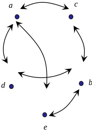
b) Perpendikulyarlik munosobatining grafi
