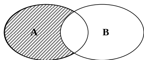
A \setminus B
