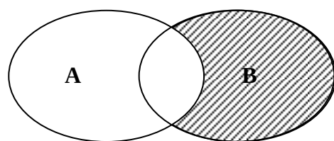
B \setminus A
