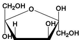
\beta -D-фруктофураноза
