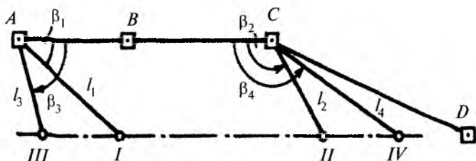
113-rasm. Poligonometriya punktidan yaqinlashuvchi yoʻlak oʻqini rejalar.
