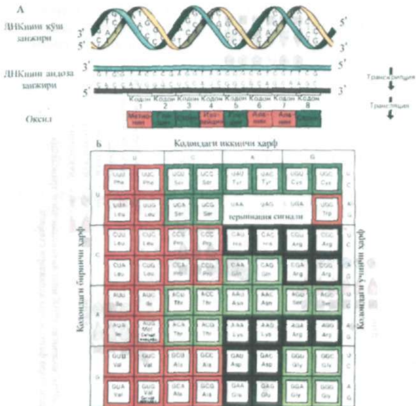
77-расм. ДНК да ифодаланган генетик коднинг маъносини аниқлаб топиш принциплари схемаси.
