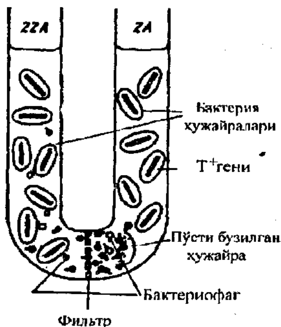
15-расм. Salmonella typhimurium бактериясида трансдукция ҳодисасини кўрсатувчи тажриба схемаси.
