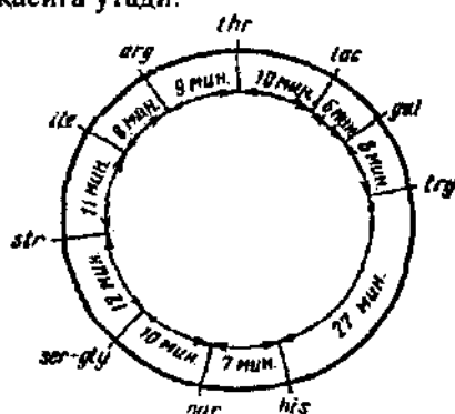
53-расм. Escherichia coli нинг генетик харитаси.
