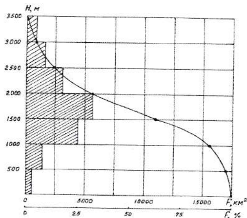
1.7.3-rasm. Daryo havzasining gipsografik egri chizig'i
