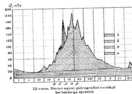
1.9.1-rasm. Daryo oqimi gidrografini vertikal bo'laklarga ajratish.
