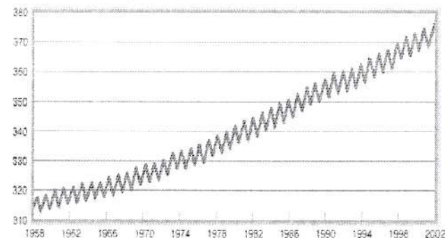
2.2.1-rasm. Killing egri chizig'i – atmosferadagi karbonat angidrid konsentratsiyasi haqida ma'lumotlar (Mauna Loa, Gavay orollari) Manba: Koliforniya universitetining Skripkovskiy okeanografiya instituti
