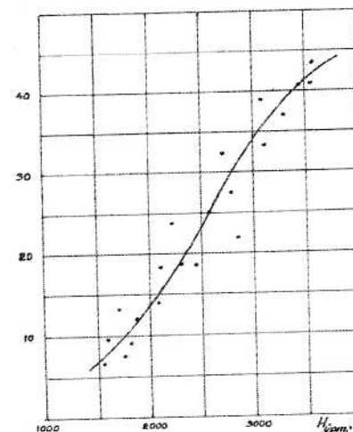
1.10.1-rasm. Oqim moduli ( M )ning havzaning o'rtacha balandligi ( H_{0.1} ) ga bog'liqligini ifodalovchi chizma
