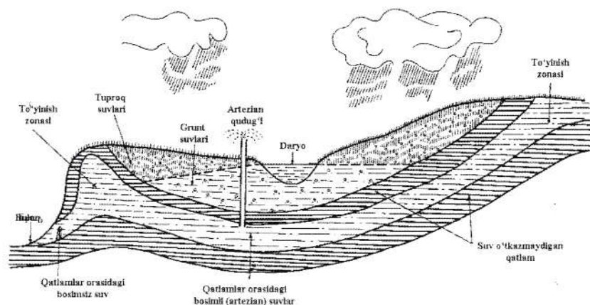
2-rasm. Artezian havza (D.S.Ibrohimov va A.N.Sultonxo'jayevlar bo'yicha)
