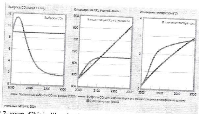
2.2.2–rasm. Chiqindilarning barqarorlashishi va karbonat ангидрид konsentratsiyasining haroratga ta'siri. Manba: MGEIK 2001
