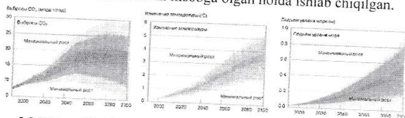
2.2.3-rasm. Chiqindilarning haroratning o'sishi va dengiz sathining ko'tarilishga ta'sirini prognozlash. Manba: MGEIK 2001
