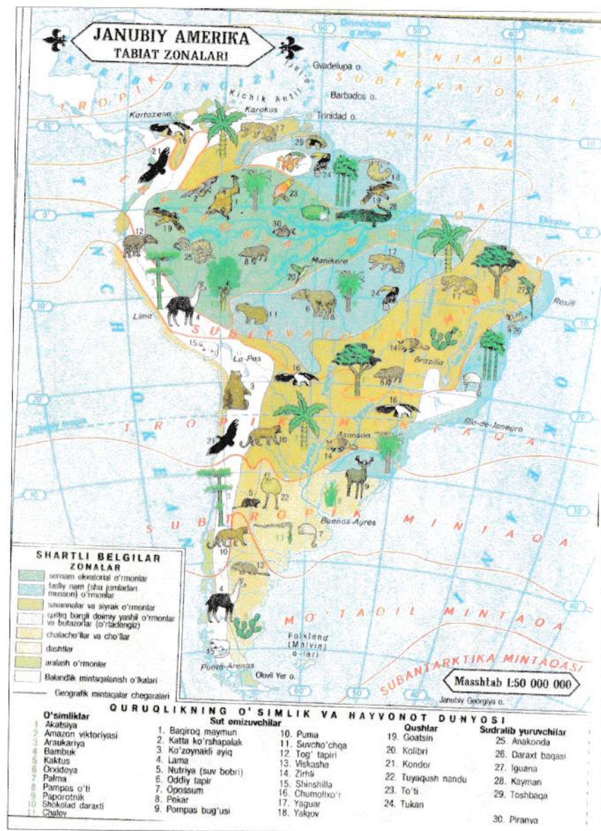
11-rasm. Janubiy Amerika materigi tabiat zonalari kartasi
