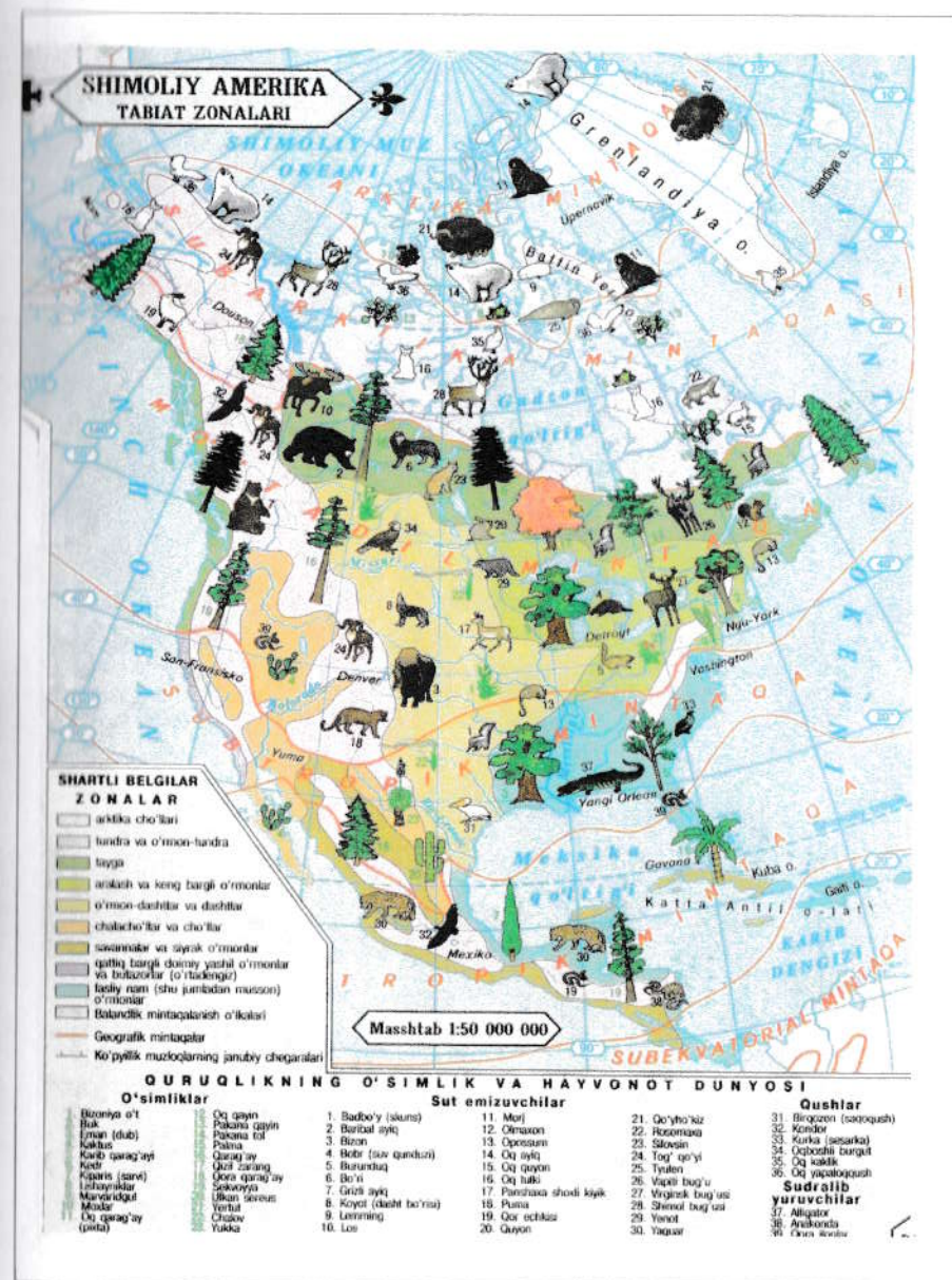
14-rasm. Shimoliy Amerika materigi tabiat zonasi kartasi
