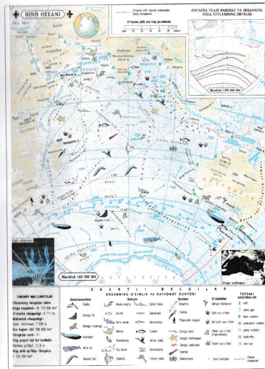
20-rasm. Hind okeani tabiiy kartasi
