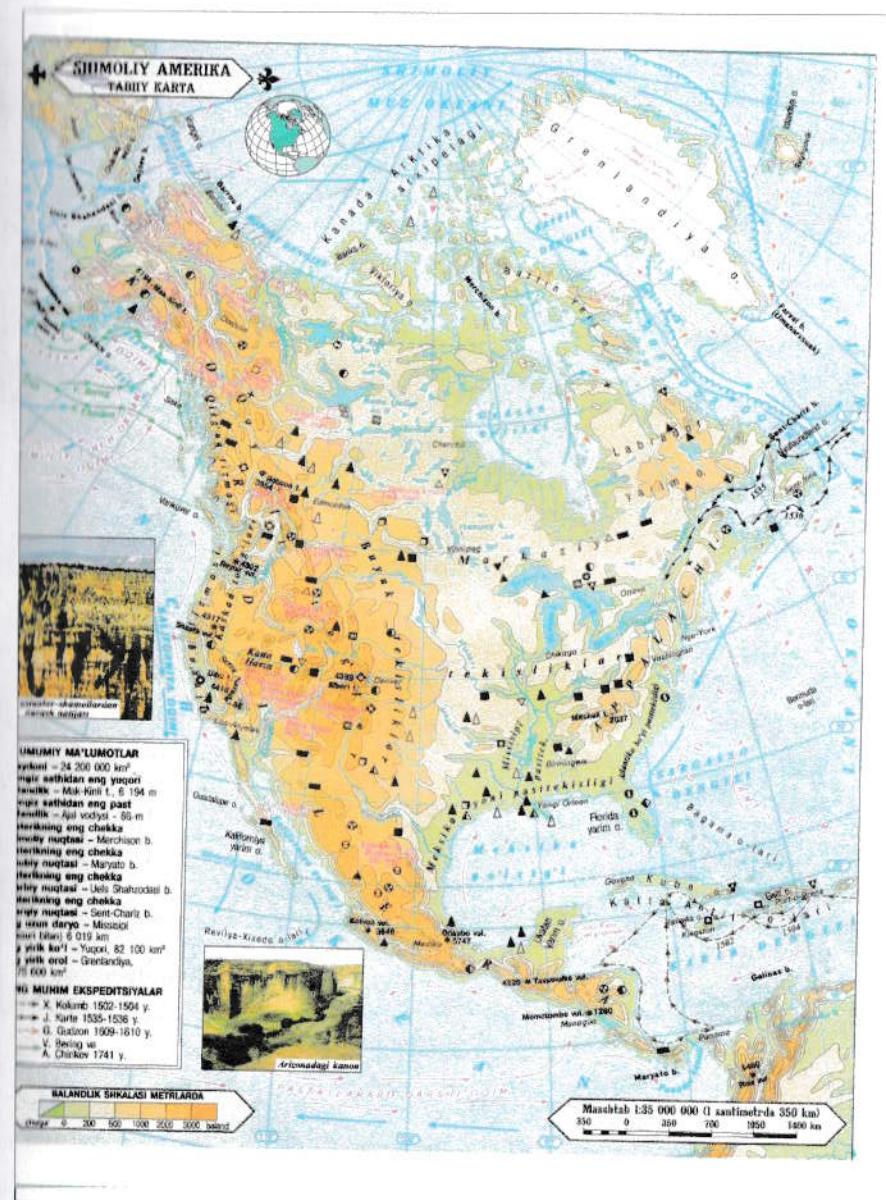
12-rasm. Shimoliy Amerika materigi tabiiy kartasi
