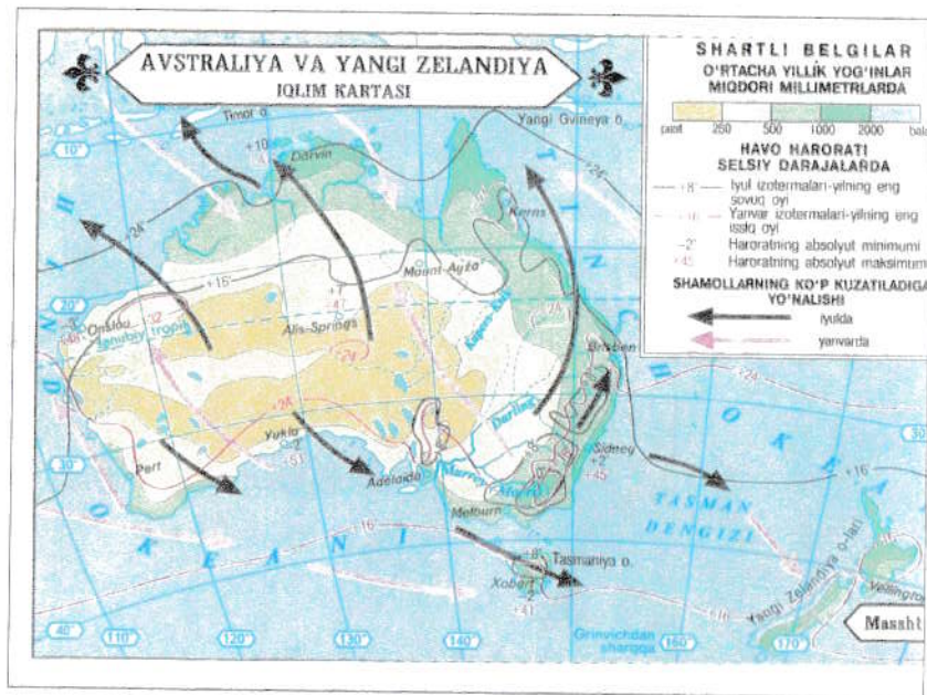
5-rasm. Avstraliya materigi iqlim kartasi
