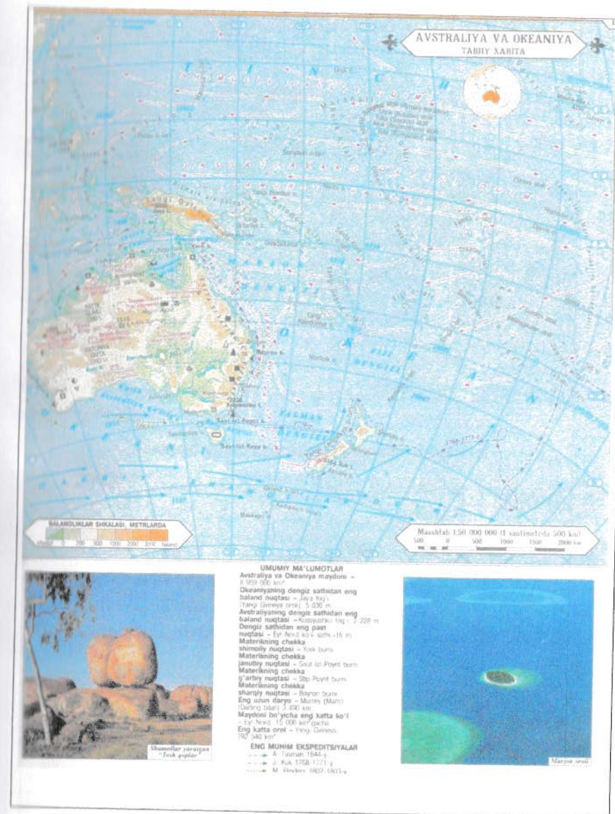
4-rasm. Avstraliya materigi va Okeaniya tabiiy kartasi
