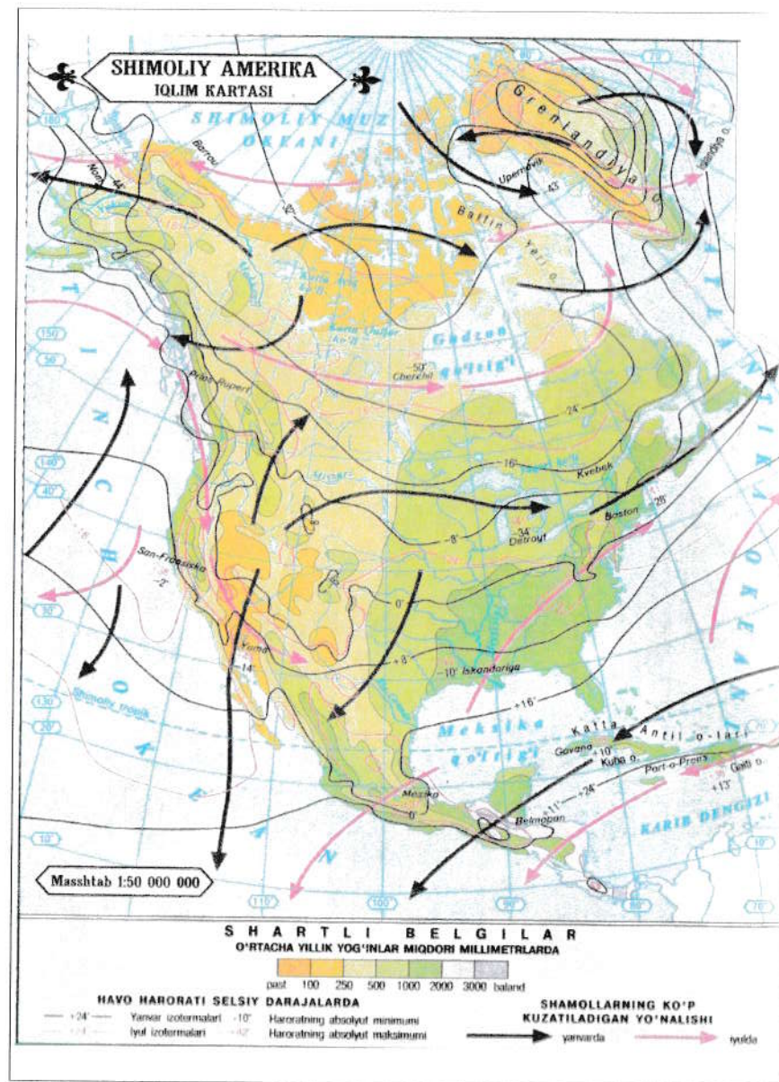
13-rasm. Shimoliy Amerika materigi iqlim kartasi
