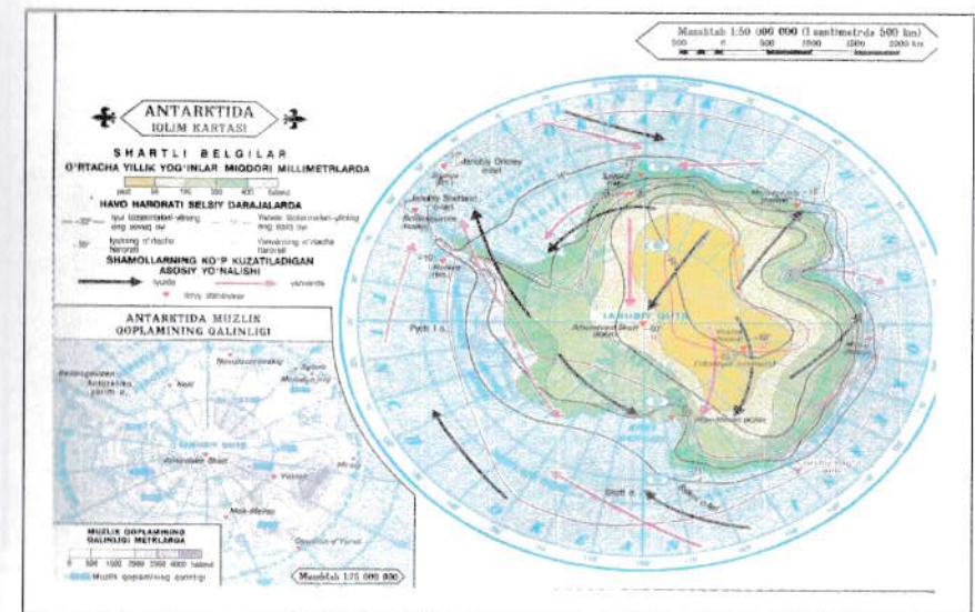
8-rasm. Antarktida materigi iqlim kartasi
