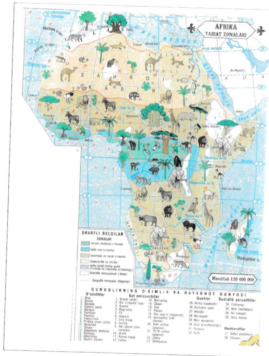
3-rasm. Afrika materigi tabiat zonalari kartasi
