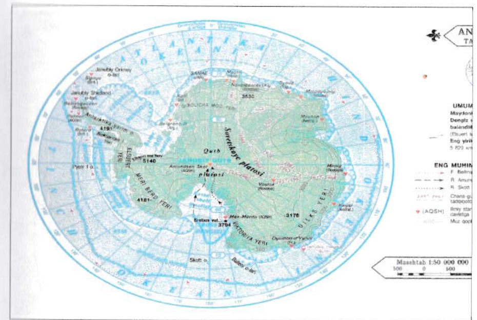
7-rasm. Antarktida materigi tabiiy kartasi
