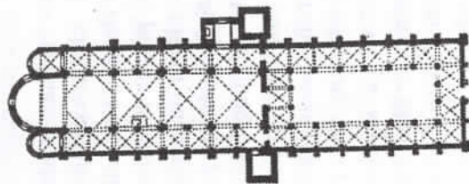
Rasm-63. Milandagi Sant Ambrođio cherkovi tarhi va umumiy ko'rinishi. X-XII asrlar.
