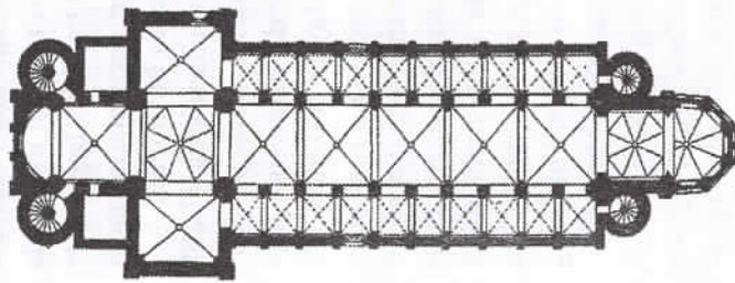
Rasm-96. Vorons sobori tarxi. Qurilishi ishlari 1171-yilda boshlanib, 1234-yilda yakunlangan.
