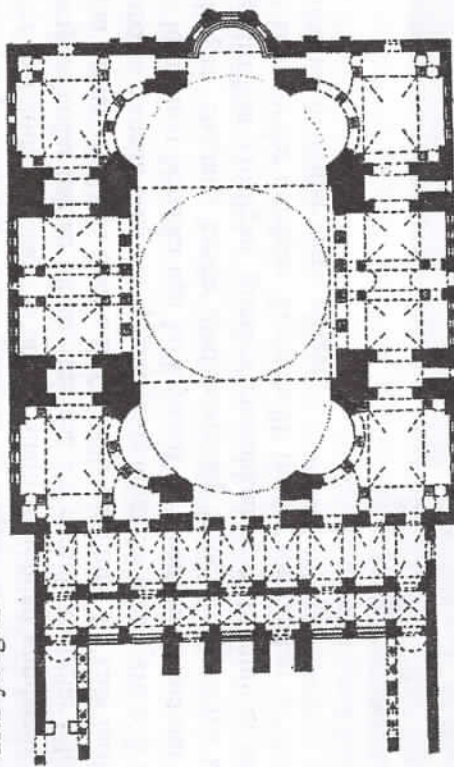
Rasm-7. Konstantinopoldagi Avliyo Sofiya ibodatxonasi tarxi. 532 – 537-yy.
