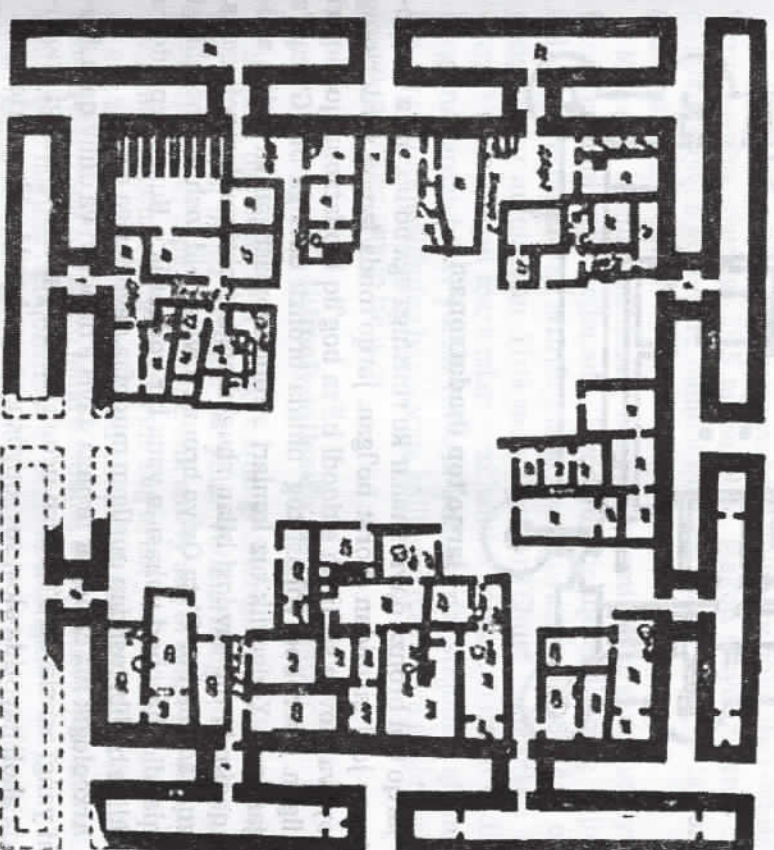
Sopollitepa yodgorligining me'morchilik rejasi
