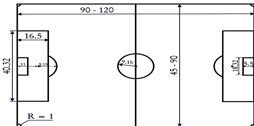
8.1 – rasm. Futbol maydoni
