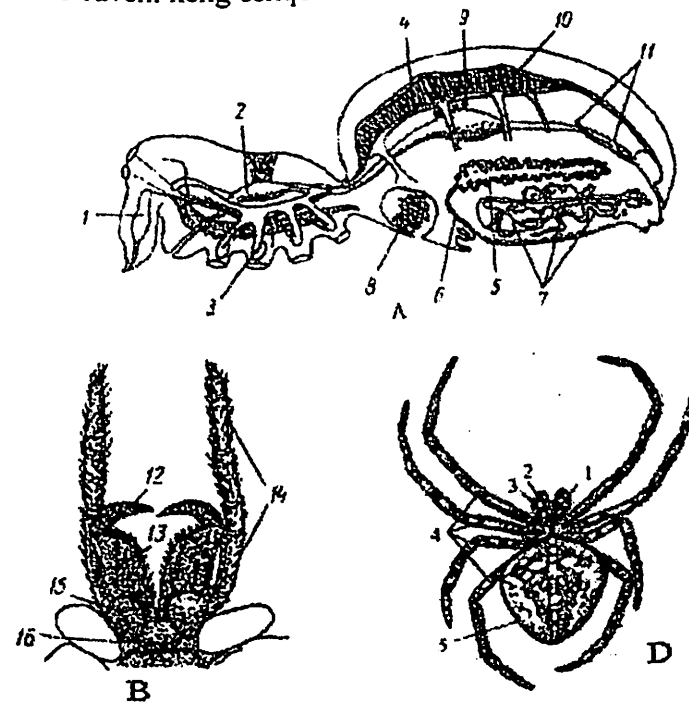
59-rasm. Butli o'rgimchak: A-ichki tuzilishi. B-xelitsera va pedipalparii. D-tashqi tuzilishi: 1-xelitsera asosidagi zahar bezi, 2-so'ruvchi oshqozon, 3-ichakning ko'r o'simalari, 4-yuragi, 5-tuxumdoni, 6-tuxum yo'li, 7-o'rgimchak bezlari, 8-o'pkasi, 9-jigari, 10-yurak teshigi, 11-malpigi naychalari, 12-xelitseraning tirnoqsimon uchki bo'limi, 13-xelitseraning asosiy bo'g'imi, 14-xelitseraning tirnoqsimon uchki bo'limi, 15-pedipalpa asosiy bo'g'imining jag' bo'lagi, 16-pastki labi. D-tashqi pedipalpari, 15-pedipalpa asosiy bo'g'imining jag' bo'lagi, 16-pastki labi. D-tashqi tuzilishi: 1-bosh-kokrak, 2-xelitseralar, 3-pedipalpari, 4-yurish oyoqlari, 5-qorin bo'limi.
