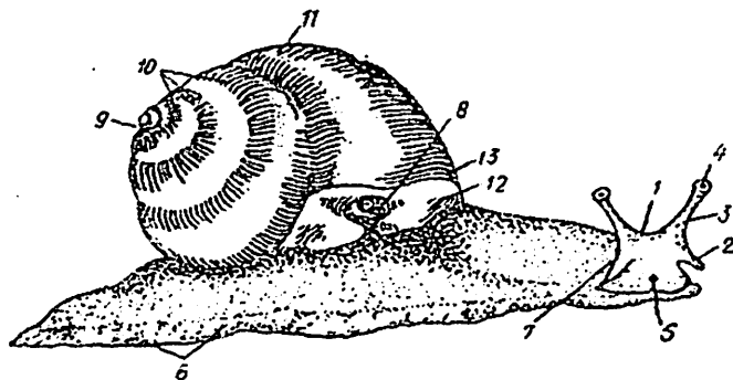
51-rasm. Tok shilliq qurtining tashqi tuzilishi: 1-boshi, 2-lab paypaslagichi, 3-ko'z paypaslagichi, 4-ko'zi, 5-og'iz bo'shlig'i, 6-oyoq, 7-jinsiy teshigi, 8-nafas olish teshigi, 9-13-chig'anoqning tuzilishi (9-cho'qqisi, 10-11-gajaklari, 12-og'izcha, 13-og'izcha qirrası).
