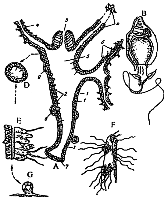
18-rasm. Gidraning ichki tuzilishi: A-gidra gavdasi tuzilishining tik kesimi; 1-ektoderma va uning ostidagi tayanch parda; 2-endoderma; 3-og'iz; 4-paypaslagichlari; 5-gastral bo'shliq; 6-paypaslagichdagi otiluvchi hujayralari; 7-tovon; 8-tuxumi rivojlanayotgan bezlar; 9-urug'don; B-otiluvchi hujayra; D-gidraning ko'ndalang kesimi. E-gidra tanasining kattalashtirilgan bir qismi; F-kattalashtirilgan muskul hujayrasi; G-paypaslagichda joylashgan otiluvchi hujayralar.
