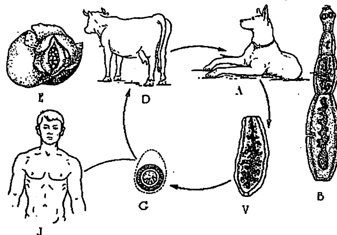
34-rasm. Exinokokk ( Echinococcus granulosus )ning rivojlanish sikli sxemasi: A-asosiy xo'jayini - yirtqich sutemizuvchilar; B-yetilgan exinokokk, V-tashqi muhitga chiqarilgan, yetilgan bo'g'imi, G-tuxumi, D-oraliq xo'jayini - qishloq xo'jalik hayvonlari va odam, E-jigardagi exinokokk pufagi; J-fakultativ oraliq xo'jayin-odam.
