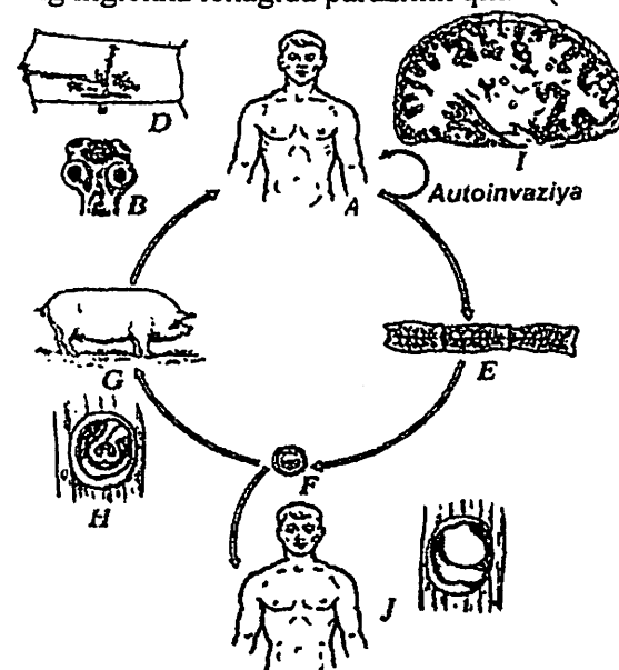
33-rasm. Cho'chqa tasmasimon chuvalchangining hayotiy sikli: A-asosiy xo'jayin-odam, B-bosh qismi, D-germafrodit bo'g'im, E-yetilgan bo'g'imlar guruhi, F-tuxum, G-oraliq xo'jayin, H-go'shtdagi finna, I-odam miyasidagi finnalar, J-odam fakultativ oraliq xo'jayin sifatida.
