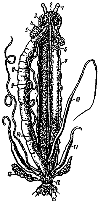
65-rasm. Ko'poyoqlilarning ichki tuzilishi: 1-mo'ylovi, 2-halqumusti gangliysi, 3-zahar bezli jag'oyoqlari, 4-qizilo'ngachi, 5-so'lak bezi, 6-qorin nerv zanjiri, 7-oyog'i, 8-o'rta ichagi, 9-malpigi naychalari, 10-urug'doni, 11-urug' pufagi, 12-urug' yo'li, 13-keyingi bezi.
