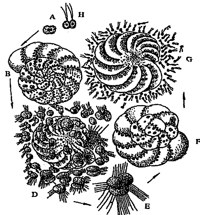
10-rasm. Foraminifera ( Elphidium krispa ) ning nasl almashinib ko'payishi: A-zigota, B-mikrosferik individ, D-mikrosferik individni ko'p marta bo'linishi, E, F-makrosferik individ hosil bo'lishi, G-makrosferik individdan gametalar hosil bo'lishi, H-gametalar kopulyatsiyasi.
