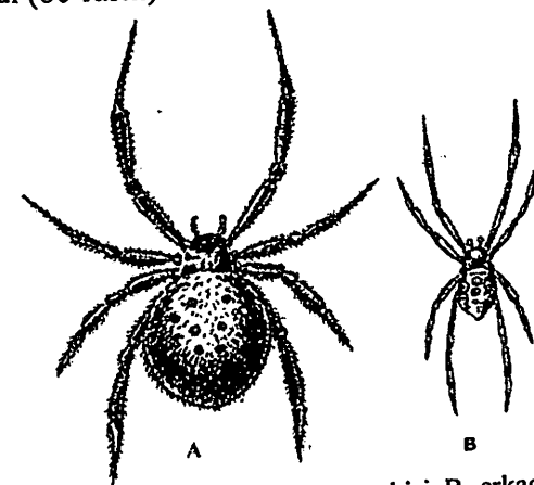
60-rasm. Qoraqurt: A-urg'ochisi, B- erkagi.
