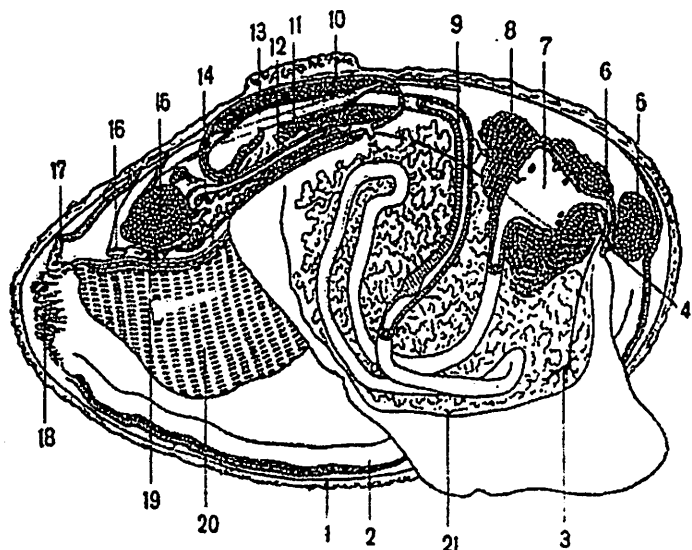
54-rasm. Baqachanoqning ichki tuzilishi: 1-chig'anoq cheti, 2-mantiya cheti, 3-pedal nerv gangliyasi, 4-og'zi, 5-oldingi tutashtirgich muskuli, 6-serebral nerv gangliyasi, 7-oshqozoni (yorib ko'rsatilgan), 8-jigari, 9-ichagi (qisman yorilgan), 10-yurak oldi bo'shlig'i, 11-yurak qorinchasidan o'tgan orqa ichagi, 12-yurak oldi bo'lmasi, 13-yurak qorinchasi, 14-buyragi, 15-orqa tutashtirgich muskuli, 16-anal teshigi, 17-kloaka sifoni, 18-jabra sifoni, 19-visseral nerv gangliyasi, 20-jabrasi, 21-jinsiy bezi.
