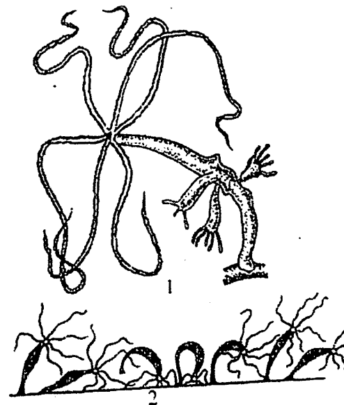
17-rasm. Chuchuk suv gidrasi-Hydra oligactis: 1-kurtaklanayotgan gidra, 2-gidraning har xil usulda harakat qilish sxemasi.
