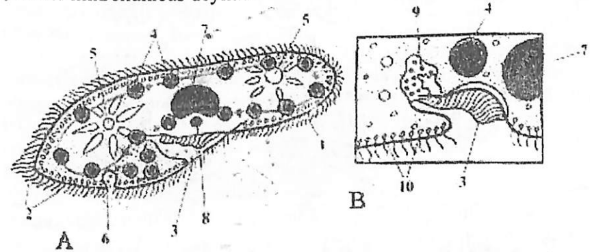
15-rasm. Infuzoriya-tufelka ( Paramecium caudatum ): A-Infuzoriya-tufelkaning tuzilishi; B-Infuzoriya-tufelkaning og'izoldi chuqurchasi: 1-hujayra qobig'i, 2-kiprikli, 3-og'iz teshigi, 4-ovqat hazm qilish vakuolalari, 5-qisqaruvchi vakuolalari, 6-poroshitsa, 7-katta yadrosi (makronukleus); 8-kichik yadrosi (mikronukleus), 9-shakillanyotgan hazm qilish vakuoli, 10-otiluvchi tanachalari (trixotsistlari).
