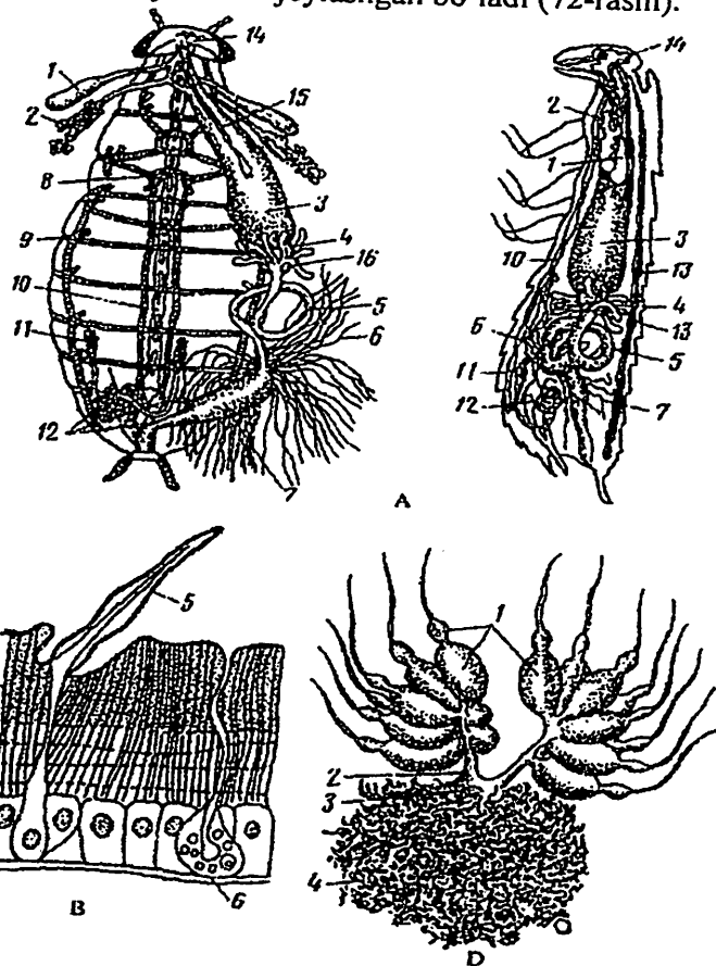
72-rasm. Qora suvarakning ichki tuzilishi. A-ichki tuzilishining orqa va yon tomonidan ko'rinishi: 1-so'lak bezi rezervuari, 2-so'lak bezi, 3-jig'ildon, 4-muskulli oshqozon, 5-o'rta ichagi, 6-malpigi naychalari, 7-orqa ichagi, 8, 9-traxeyalari, 10-qorin nerv zanjiri, 11-urug'don, 12-jinsiy bezlar, 13-yuragi, 14-bosh miyasi, 15-simpatik nerv sistemasi, 16-pilorik (ko'r) o'simtalari; B-kutiikulasining tuzilishi: 1-epikutikula, 2-ekzokutikula, 3-endokutikula, 4-gipoderma, 5-qil, 6-teri bezi; D-urg'ochilik jinsiy organi: 1-tuxumdon naylari, 2-tuxum yo'li, 3-urug' qabul qilgichi, 4-bezlar.
