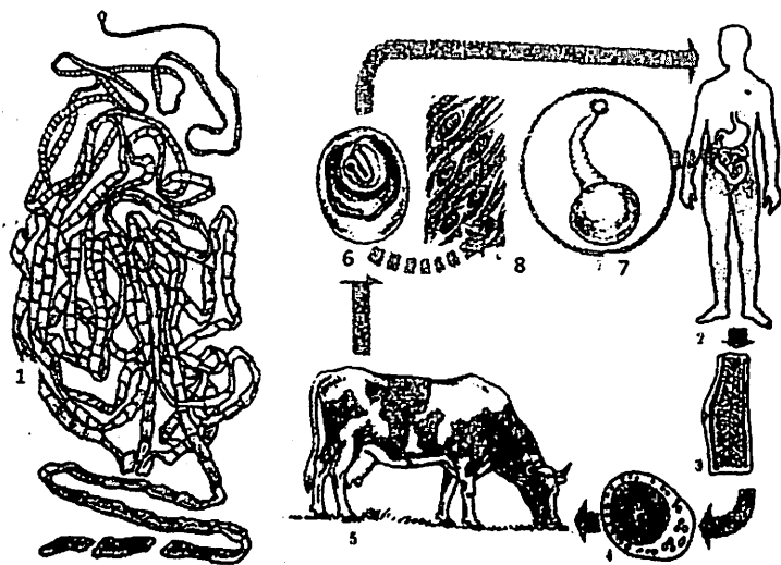
32-rasm. Qoramol tasmasimon chuvalchangi ( Taeniarhynchus saginatus ) ning tashqi tuzilishi va rivojlanish sikli: 1-voyaga yetgan sestoda; 2-asosiy xo'jayini; 3-harakatchan bo'g'ini; 4-onkosferali tuxumi; 5-oraliq xo'jayini; 6-finnasi (sistiserk); 7-asosiy xo'jayini ichagida sestodaning rivojlanishi; 8-sistiserk bilan zararlangan hayvon go'shti.
