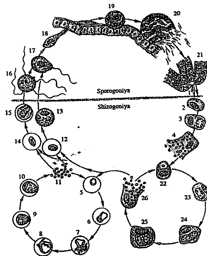
14-rasm. Bezgak parazitining rivojlanish sikli sxemasi: 1-bezgak chivini so'lak bezidan odam qoniga chiqayotgan sporozoitlar; 2,3-sporozoitlarning jigar hujayralarida ko'payishi; 4-shizogo-niya yo'li bilan sporozoitlardan merozoitlarning hosil bo'lishi; 5-11-eritrotsitlarda shizogoniya yo'li bilan merozoitlarning ko'payishi; 12,13-makrogametotsitning yetilishi; 14,15-mikrogametotsitlarning yetilishi; 16,17-makrogameta va mikrogametalar hosil bo'lishi va ularning qo'shilishi; 18-zigota-ookinetalarining chivin ichagi hujayralariga kirishi; 19, 20-sporozoitlar hosil bo'lishi va chivin tana bo'shlig'iga chiqishi; 21-sporozoitlarning chivin so'lak beziga o'tishi; 22-26-parazitning odam hujayralarida rivojlanishi.
