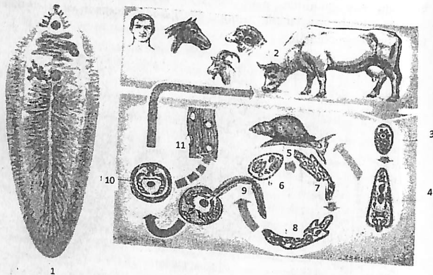
26-rasm. Oddiy jigar qurtining taraqqiyot sikli sxemasi: 1-jinsiy voyaga yetgan shakli (marta), 2-asosiy xo'jayinlari, 3-tuxum, 4-miratsidiy, 5-oraliq xo'jayini-mollyuska, 6-sporosista, 7-yosh rediy, 8-yetilgan rediy, 9-serkariy, 10-adoleskariy, 11-o'tga yopishgan adoleskariylar.
