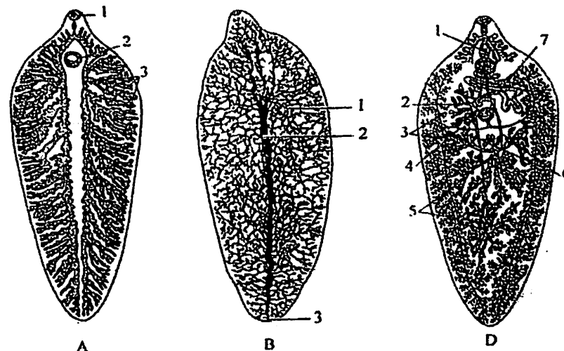
25-rasm. Oddiy jigar qurtining ovqat hazm qilish, ayirish va jinsiy organlari: A-ovqat hazm qilish sistemasi, 1-og'iz so'rg'ichi, 2-qorin so'rg'ichi, 3-shoxlanib ketgan ichagi, B-ayiruv organlari: 1-ayiruv organining naychalari, 2-asosiy ayirish kanali, 3 asosiy ayirish kanali teshikchasi, D-jinsiy sistemasi: 1-qo'shilish organi (sirrus), 2-tuxumdoni, 3-sariqdonlari, 4-sariqdon yo'llari, 5-urug'donlari, 6-urag' yo'llari, 7-bachadoni.
