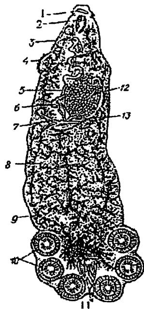
30-rasm. Baqa ko'pso'rg'ichlisi ( Polystoma integerrimum ): 1-og'iz, 2-halqum, 3-jinsiy teshik, 4-qin, 5-urug' yo'li, 6-bachadon, 7-sariqdonning yo'li, 8-sariqdonlar, 9-ichak, 10-yopishish diskasidagi so'rg'ichlari, 11-yopishuv diskasidagi katta ilmoqlari, 12-tuxum yo'li, 13-tuxumdon.
