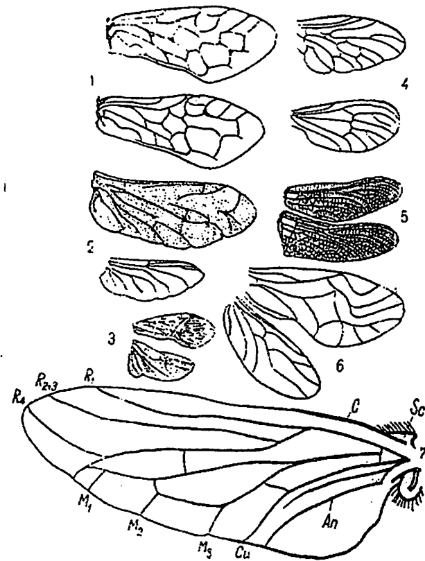
69-rasm. Hasharotlar qanotlarining har xil shakllari va ularning tomirlanish tiplari: 1-parda qanotlarniki; 2-qo'ng'izlarniki; 3-qatiq qanotlarniki; 4-pashshalarniki; 5-ninachilarniki; 6-pichanxo'rlarniki; 7-vizildoq pashshalarniki: C-kostal tomir; Sc-subkostal tomir; M 1 -M 2 -M 3 -medial tomirlar va ularning tarmoqlari; Cu-kubital tomir; A n -anal tomir; R 1 -R 4 -radial tomirlar va ularning shoxchalari.
