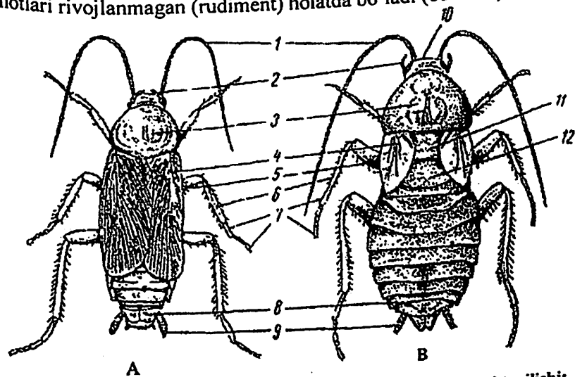
66-rasm. Erkak (A) va urg'ochi (B) qora suvarakning tashqi tuzilishi: 1-mo'ylovlari, 2-jag'paypaslagichlari, 3-oldingi ko'krak bo'g'imi, 4-ustqanoti, 5-soni, 6-boldiri, 7-panjasi, 8-qorinning o'ninchi bo'g'imi, 9-serkilari, 10-boshi, 11-o'rta ko'krak bo'g'imi, 12-orqa ko'krak bo'g'imi.
