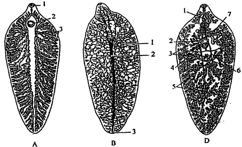
25-rasm. Oddiy jigar qurtining ovqat hazm qilish, ayirish va jinsiy organlari:
