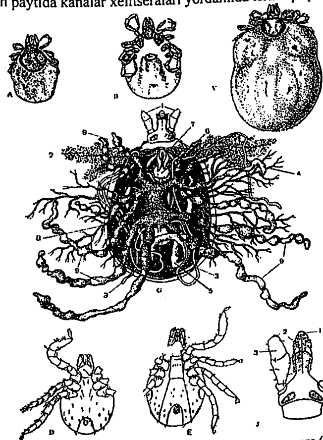
63-rasm. It kanasi ( Ixodes ricinus ): A va B-urg'ochi och kana: orqa (A) va qorin (B) tomonidan ko'rinishi. V-qonga to'ygan kana, G-qon so'rib to'ygan it kanasining ichki tuzilishi: 1-xartumchasi, 2-so'lak bezlari, 3-malpigi tomirlari, 4-traxeyalari, 5-tuxumdoni, 6-miyasi, 7-qizilo'ngachi, 8-o'rta ichagi, 9-o'rta ichakning ko'r o'simtalari, D-lichinkasi qorin tomonidan ko'rinishi, E-nimfasi qorin tomonidan ko'rinishi, J-urg'ochi it kanasining xartumchasi: 1-giposomi, 2-xeliserasining oxirgi bo'g'imi, 3-pedipalpsi.
