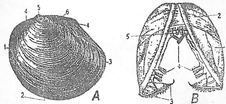
53-rasm. Baqachanoq ( Anadonta sygnea )ning tashqi ko'rinishi va gloxidiy lichinkasining tuzilishi: A-baqachanoq: 1-oldingi qirrasi, 2-qorin qirrasi, 3-orqa qirrasi, 4-yelka qirrasi, 5-chig'anoq cho'qqisi, 6-chig'anoqni quruvchi tashqi paylar; B-baqachanoq lichinkasi-gloxidiy: 1-lichinka chig'anog'i, 2-chig'anoqni yopuvchi muskuli, 3-chig'anoq tishchalari, 4-sezgir tukchalar to'plami, 5-bissus bezlari.
