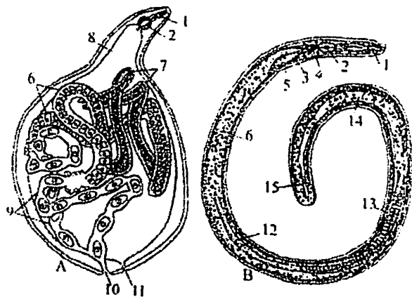
42-rasm. Ildiz bo'rtma nematodasining tuzilishi: A-urg'ochisi; B-erkagi: 1-stileti; 2-halqumi; 3-halqum oldi bezi; 4-nerv halqasi; 5-ayiruv teshikchasi; 6-o'rta ichak; 7-tuxumdoni; 8-tuxum yo'li; 9-bachadoni; 10-jinsiy teshigi 11-anal teshigi; 12-urug'doni; 13-urug' yo'li; 14-urug' to'kuvchi kanali; 15-spikulasi.
