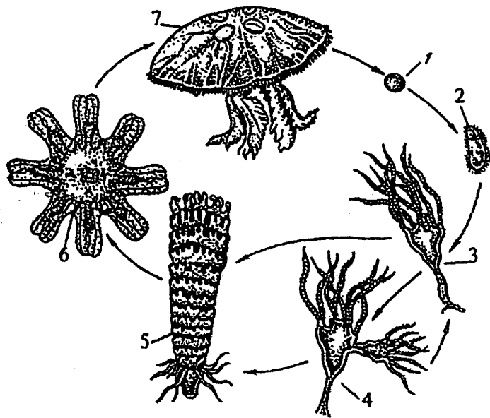
21-rasm. Aureliya meduzasining rivojlanish jarayoni: 1-tuxum; 2-planula lichinkasi; 3-sifistoma; 4-kurtaklanayotgan sifistoma; 5-bo'linish yo'li bilan efiralar hosil bo'lishi; 6-efira; 7-voyaga yetgan meduza.
