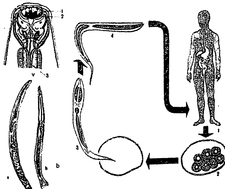
40-rasm. Qiyshiqbosh nematoda ( Ancylostoma duodenale ): a-urg'ochisi, b-erkagi, v-qiyshiqbosh nematodaning og'iz qismi (og'iz kapsulasida kutikulyar tishchalari tasvirlangan): 1-kutikulyar tishlari, 2-og'iz bo'shlig'i, 3-halqumi, g-qiyshiqbosh nematodaning rivojlanish sikli:1-odam, qiyshiqbosh nematodaning xo'jayini, 2-tuxumi, 3-tuxumdan rabbitsimon lichinkaning chiqishi, 4-yuqumli lichinkasi.
