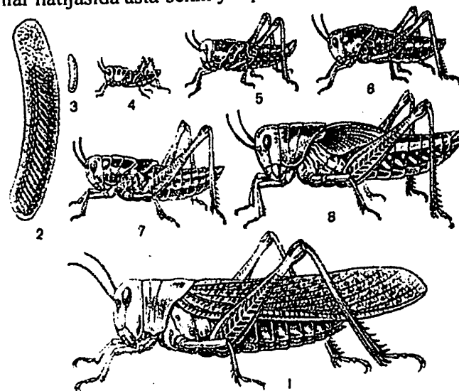
73-rasm. Chala metamorfozli hasharotlar vakili-Osiyo chigirtkasi ( Lacusta migratoria ) ning rivojlanish bosqichlari: 1-voyaga yetgan qanotli chigirtka, 2-tuproqda ko'zacha ichidagi chigirtka tuxumlar, 3-tuxumi, 4,5,6,7,8-beshikta bosqichdagi lichinkalari.
