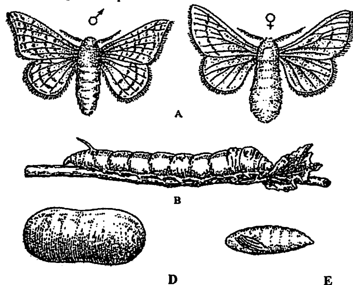
74-rasm. Tut ipak qurtining to'liq metamorfoz orqali rivojlanishi. A-kapalak. B-qurt. D-pilla. E-pilladan chiqarib olingan g'umbak.
