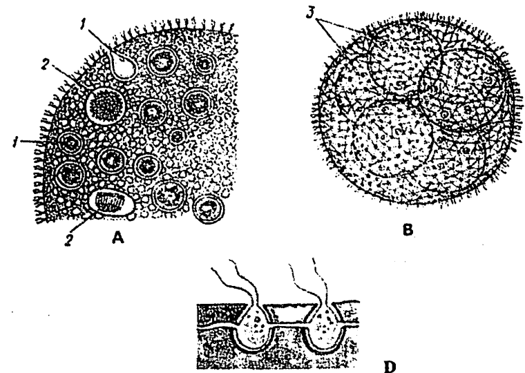
4-rasm. Volvoks ( Volvox globator ): A-Volvox globator koloniyasining jinsiy hujayralari bo'lgan bir qismi. B-Volvox aureus koloniyasining jinsiz ko'payishi: 1-makrogameta, 2-mikrogametalar, 3-ona koloniya ichidagi yosh koloniyalar, D-volvoks koloniyasidagi ikkita hujayrasi.
