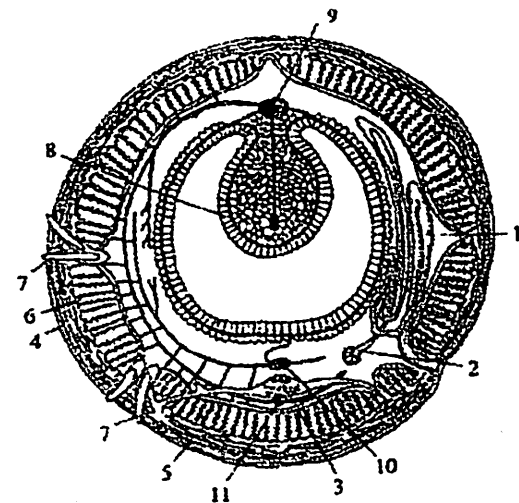
48-rasm. Yomg'ir chuvalchangining ko'ndalang kesimi: 1-metanefridiy, 2-metanefridiy voronkasi, 3-qorin nerv zanjiri gangliysi, 4-teri epiteliysi, 5-ko'ndalang muskullar, 6-bo'ylama muskullar, 7-qillar, 8-ichak tiflozoli, 9, 10-orqa va qorin qon tomirlari, 11-subnevral nervlar.
