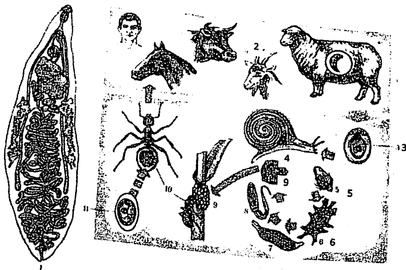
27-rasm. Lansetsimon ikki so'rg'ichlisining tuzilishi va taraqqiyot sikli: 1-voyaga yetgan shakli; 2-asosiy xo'jayinlari; 3-tuxumi; 4-birinchi oraliq xo'jayini va 5-9-lichinkalik taraqqiyoti (5-miratsidiy; 6-7-sporosistalar; 8-serkariy; 9- serkariy tugunchalari); 10-ikkinchi oraliq xo'jayini-chumoli; 11-metaserkariy.
