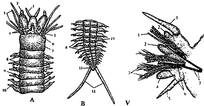
44-rasm. Nereisning tashqi tuzilishi. Nereisning oldingi (A) va keyingi (B) tomoni: 1-paypaslagichlari (antennalari), 2-palpi, 3-og'iz yoni mo'ylovlari, 4-ko'zlari, 5-boshining oldingi bo'g'imi (prostomium), 6-hidlash chuqurchasi, 7-boshining keyingi bo'g'imi (peristomium), 8-parapodiylar, 9-qillari, 10-orqa mo'ylovi, 11-pigidiysi, 12-anal mo'ylovlari, 13-orqa qon tomiri; V-parapodiysi: 1-orqa mo'ylovi, 2-parapodiyning orqa shoxi, 3-qillar tutami, 4,6-parapodiyning qorin shoxlari, 5-parapodiyning qorin mo'ylovi, 6-tayanch qillar.
