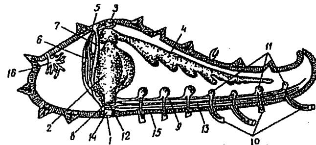
76-rasm. Oddiy amur dengiz yulduzi ( Asterias amurensis ) ning ichki tuzilishi: 1-og'zi, 2-oshqozoni, 3-anal teshigi, 4-ovqat hazm qilish sistemasining bir tarmog'i, 5-ovqat hazm qilish radial tarmoqlarining boshlanish joyi, 6-madrepor tarmog'i, 7-tayanch organi, 8-tosh kanal, 9-radial ambulakral kanal, 10-plastinkasi, 11-ambulakral ampulalari, 12-halqa va radial qon ambulakral oyoqchalari, 13-radial nerv tomiri, 14-halqum, 15-terisida shakllanayotgan skeleti, 16-jinsiy bezlari.
