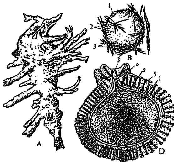
16-rasm. Chuchuk suv bodyaga ( Spongilla lacustris ) si: A-suv osti o'simligidagi bodya-galar; B-gemmula; 1-g'ovaklar teshigi; 2-skelet ignalari; 3-gemmulaning mikroskleritlari; D-gemmula tanasining kesmasi: 1-amfidiskalar; 2-ichki kutikula qobig'i; 3-tashqi muhit bilan bog'lab turuvchi teshikcha; 4-shu teshikchani yopib turadigan to'siq parda; 5-gemmula tanasi ichidagi hujayralar.
