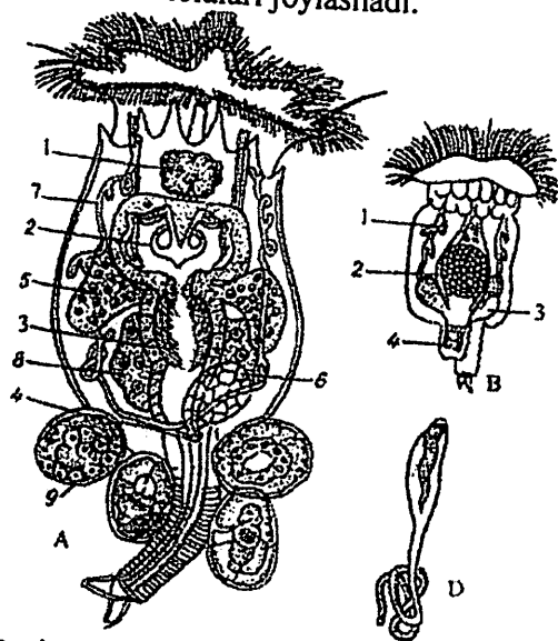
43-rasm. Og'izaylangichlilardan- Brachionus rubens ning tuzishi: A-urg'ochisi: 1-nerv tuguni, 2-mastaks-halqumdagi kavshovchi jag'i, 3-ichak, 4-anal teshigi, 5-so'lak bezi, 6-siydik pufagi, 7-protonefridiy, 8-tuxumdoni, 9-tuxumlari, B-mitti erkagi: 1-protonefridiy, 2-urag'-doni, 3-siydik pufagi, 4-qo'shilish oigani, D-protonefridiy va uning chiqarish naychasi.
