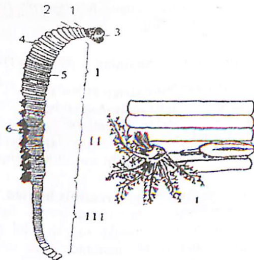
45-rasm. Qum chuvalchangi ( Arenicola marina )ning tuzilishi: I-prostomiumi, 2-perestomiumi, 3-ag'darilgan qismi, 4-parapodiyning orqa shoxchasi, 5-parapodiyning qorin shoxchasi, 6-jabralari, I-tananing parapodiyli qismi, II-tananing parapodiyli va jabrali qismi, III-dum qismi. IV- tananing parapodiyli va jabrali qismining kattalashtirilgan ko'rinishi.
