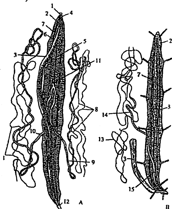
37-rasm. Odam askaridasining ichki tuzilishi: A-urg'ochisi. B-erkagi: 1-lablari; 2-qizilo'n-gachi; 3-ichagi; 4-halqum nerv halqasi; 5-qorin nervi; 6-ayirish sistemasi nayi; 7-fagotsitar hujayralar; 8-tuxumdoni; 9-tuxum yo'li; 10-bachadoni; 11-jinsiy qini; 12-anal teshigi; 13-urug'doni; 14-urug' yo'li; 15-urag' chiqarish nayi.
