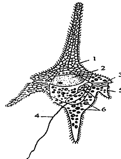
3-rasm. Seratsium ( Ceratium hirudinella ) ning tuzilishi (Averinsev, 1962): 1-qalqon plastinkalaridan biri; 2-yadro; 3-egatcha; 4-xivchin; 5-qalqon o'simalari 6-xromatoforlar
