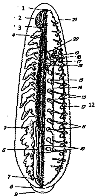
50-rasm. Tibbiyot zulugi ( Hirudo medicinalis ) ning ichki tuzilishi: 1-serebral gangliysi, 2-halqumi, 3-qizilo'ngachi, 4-oshqozoni, 5-oshqozonining orqa o'simtasi, 6-o'rta ichagi, 7-orqa ichagi, 8-anal teshigi, 9-orqa so'rg'ichi, 10-qorin nerv zanjiri gangliysi, 11-metanefridiylari, 12-siydik pufagi, 13-urug' xaltasi, 14-urug' yo'li, 15-metanefridiysining kiprikli voronka-lari, 16-qini, 17-tuxum xaltasi ichida tuxumi bilan, 18-urug'don o'simtasi, 19-penis (urug' to'kish nayi), 20-qo'shimcha bezi, 21-yon lakuni.
