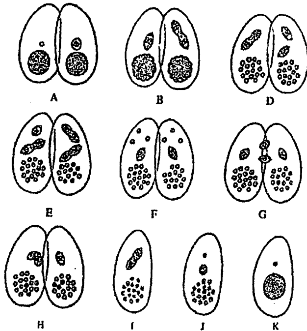
15-rasm. Infuzoriya-tufelka ( Paramaecium caudatum ) da konyugatsiya jarayonining borish sxemasi: A-konyugatsiyaning boshlanishi; B-D-mikronukleusning birinchi bo'linish bosqichi; E-mikronukleusning ikkinch bo'linish bosqichi; F-mikronukleusning uchunchi marta bo'linishi; G-H-migratsiyalanuvchi yadroning statsionar yadro bilan qo'shilib, sinkarion yadro hosil qilishi; I-sinkarion yadroning to'rtinchi marta bo'linishi natijasida sakkizta yadroning hosil bo'lishi; J-K-infuzoriyaning keyingi bo'linishi.
