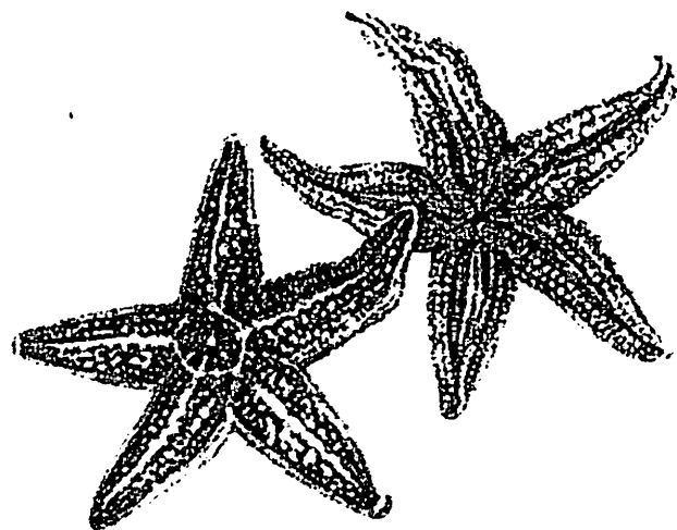
75-rasm. Oddiy amur dengiz yulduzi Asterias amurensis : chapda ustki tomondan va o'ngda qorin tomondan ko'rinishi.
