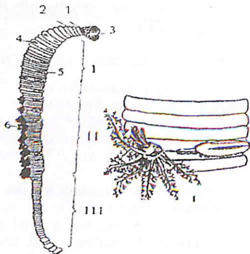
45-rasm. Qum chuvalchangi ( Arenicola marina )ning tuzilishi: 1-prostomiumi, 2-perestomiumi, 3-ag'darilgan qismi, 4-parapodiyning orqa shoxchasi, 5-parapodiyning qorin shoxchasi, 6-jabralari, I-tananing parapodiyli qismi, II-tananing parapodiyli va jabrali qismi, III-dum qismi. IV- tananing parapodiyli va jabrali qismining kattalashtirilgan ko'rinishi.
