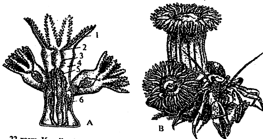
22-rasm. Korall poliqlar. A-korall poliqlar koloniyasi bir qismining tuzilishi: 1-paypaslagichlari, 2-og'iz teshigi, 3-halqumi, 4-ichak bo'shlig'i, 5-mezenterial iplari, 6-tuxum hujayralari; B-zohid qisqichbaqa chig'anog'i ustiga yopishib olgan aktiniya.
