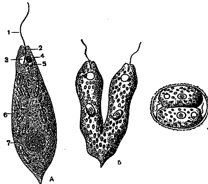
2-rasm. A-Yashil evglena ( Euglena viridis ): 1-xivchini; 2-stigmasi; 3-rezervuari; 4-qisqaruvchi vakuolasi; 5-qisqaruvchi vakuolasi; 6-xromatoforlari; 7-yadrosi. B-evglenani bo'linishi; V-evglenani sistada bo'linishi.
