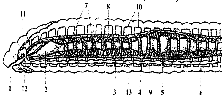
47-rasm. Yomg'ir chuvalchangining ichki tuzilishi: 1-og'zi, 2-halqumi, 3-qorin qon tomiri, 4-jig'ildoni, 5-oshqozoni, 6-ichagi, 7-yuragi, 8-orqa qon tomiri, 9-qorin nerv zanjiri, 10-tana bo'shlig'i, 11-halqum usti nerv tuguni, 12-halqum osti nerv tuguni, 13-qorin nerv tuguni.
