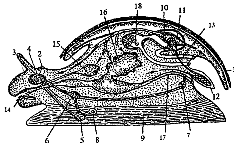
52-rasm. Qorinoq mollyuskalarning ichki tuzilishi sxemasi: 1-chig'anog'i, 2-ko'zi, 3-paypaslagichi, 4-bosh nerv gangliysi, 5-oyoq nerv gangliysi, 6-plevral nerv gangliysi, 7-visseral nerv gangliysi, 8-statotsisti, 9-oyoq, 10-yuragi, 11-yurak oldi xaltasi bo'shlig'i, 12-jabralari, 13-ayirish organlari, 14-qirg'ichi, 15-so'lak bezi, 16-jigari, 17-orqa ichagi, 18-jinsiy bezi.
