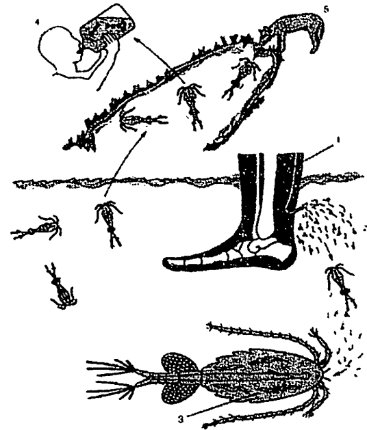
39-rasm. Rishtaning rivojlanish sikli sxemasi: 1-asosiy xo'jayini-odam terisi ostida parazitlik qilayotgan jinsiy yetuk rishta; 2-odam organizmidan suvga tushayotgan rishta lichinkalari; 3-rishta lichinkasi bilan zararlangan siklop; 4,5-rishta lichinkasi bilan zararlangan siklopni suv bilan yutayotgan odam va it.
