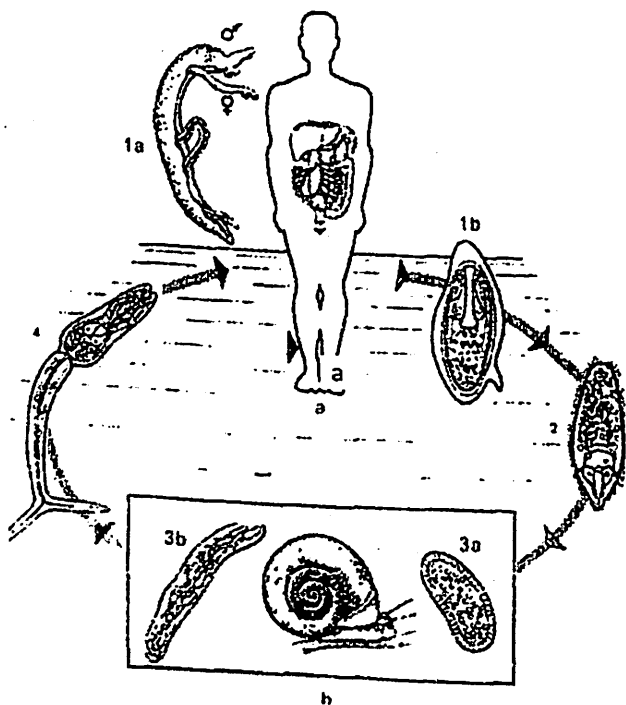
29-rasm. Qon ikki so'rg'ichlilar ( Schistosoma sp. ) ning rivojlanish sikli: a-asosiy xo'jayini: la-urg'ochi va erkak parazitlarning kopulyatsiyasi, 1b-parazitning tuxumi, 2-miratsidiy lichinkasi, b-Qon ikki so'rg'ichlilarning rivojlanish sikli sxemasi: 3-Planorbis urug'iga mansub qorinoyoqli mollyuska, 3a-birinchi yoshdagi sporosista, 3b-ikkinchi yoshdagi sporosista, 4-serkariy.
