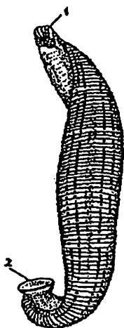
49-rasm. Tibbiyot zulugi ( Hirudo medicinalis ): 1-oldingi so'rg'ichi, 2-keyingi so'rg'ichi.
