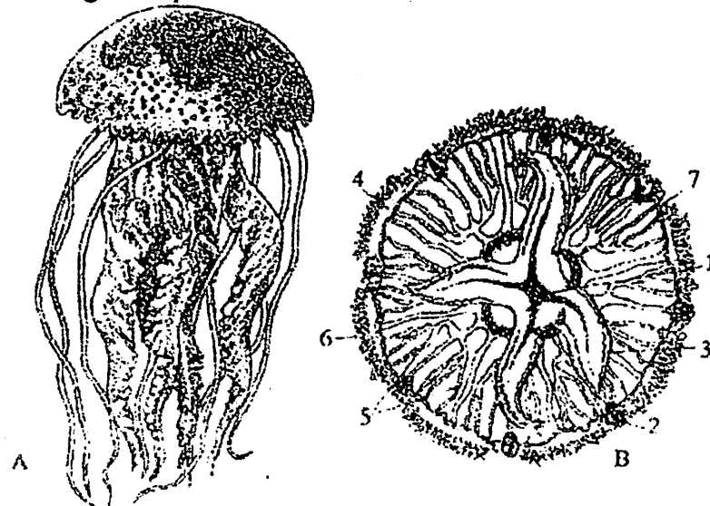
20-rasm. Ssifoid meduzalar: A-Ildizog'iz meduza, B-Aureliya ( Aurelia aurita ): 1-og'iz, 2-ropaliya, 3-og'iz bo'laklari, 4-halqa nay, 5-radial naylar, 6-paypaslagichlar, 7-jinsiy bezlar.
