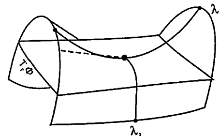
Giperbolik nuqta
