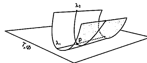
Parabolik nuqta
