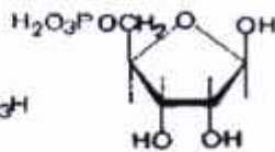
riboza-5-fosfat
