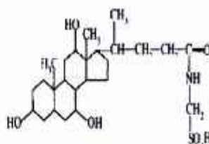
Tsarexolat kislotasi
