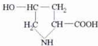
Oksiprolin
