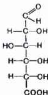
D-glyukouron kislota
