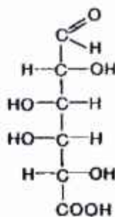
D-galaktouron kislota
