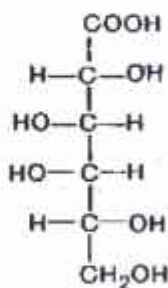
D-galakton kislota
