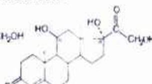
Gidrokortizon(kortizol)
