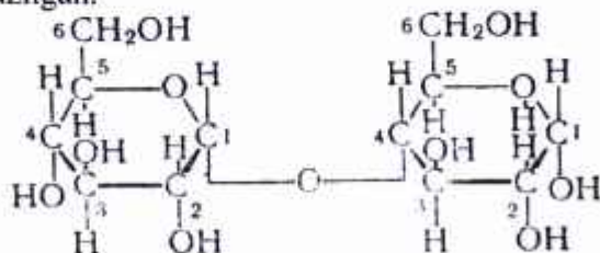
maltoza
