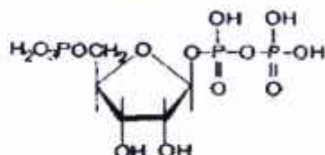
5-fosforibozil-1-pirofosfat
