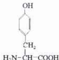
Tirozin
