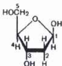
2-dezoksi-D-ribofuranosa
