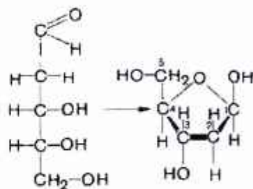
D-2- dezoksiriboza
