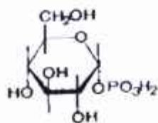
glyukoza-1-fosfat
