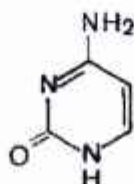
Sitozin
