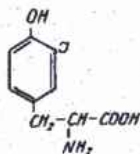
3'-monoyodtirozin (MIT)
