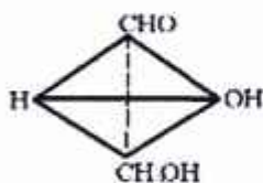
D-glitseraldegid
