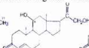
Kortikosteron
