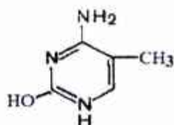
5- metil-sitozin
