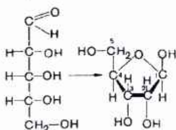
D- riboza
