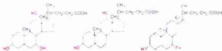
Xenodezoksixolot kislotasi
