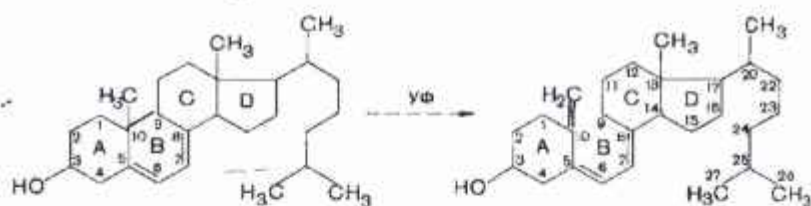
7-Degidroholesterin
