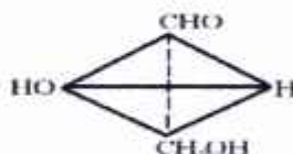
L-glitseraldegid
