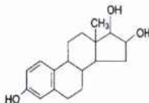
Esterol
