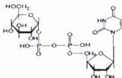
Uridindifosfatglyukoza (UDF-glyukoza)
