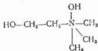
xolin
