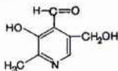
Piridoksal
