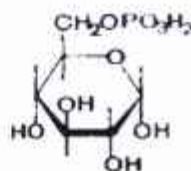
glyukoza-6-fosfat
