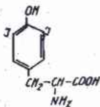
3,5- diyodtirozin (DIT)
