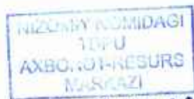
Alanin
