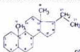
Pregnan
