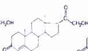
Dezoksikortikosteron
