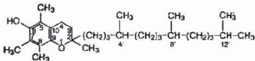
\alpha - tokoferol
