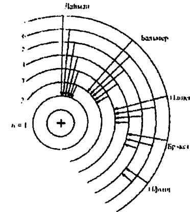
37-rasm. N. Bor bo'yicha vodorod atomining spektral seriyalari
