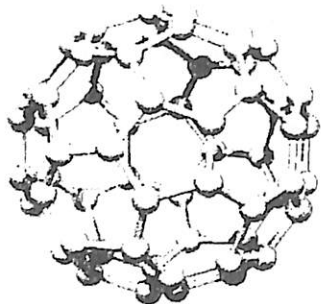
43-rasm. Fulleren molekulası
