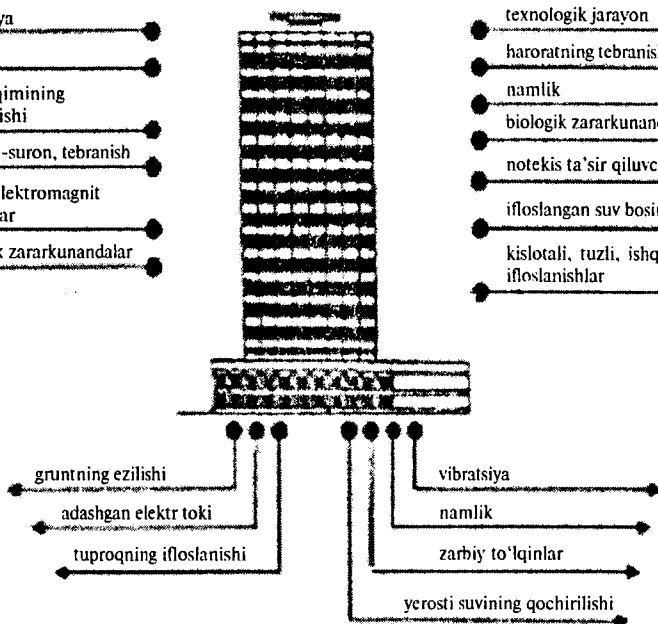
2.5- rasm. Fuqaro va sanoat binolarining atrof-muhitga ko'rsatadigan ta'sirlari.
