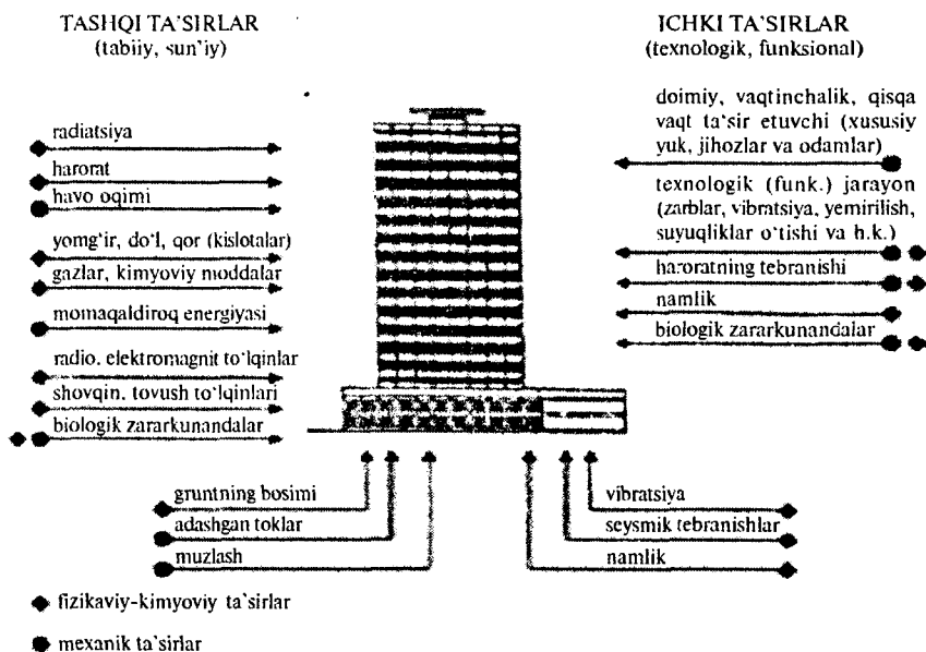
2.4- rasm. Binoga taʼsir qiluvchi (tashqi va ichki) taʼsirlar.
