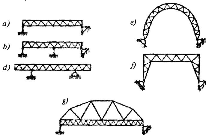
9.2- rasm. Metall ferma turlari:
