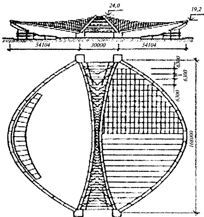
6.4- rasm. Krilatskiydagi (Rossiya) velopoyga o'yingohi yopmasi.
