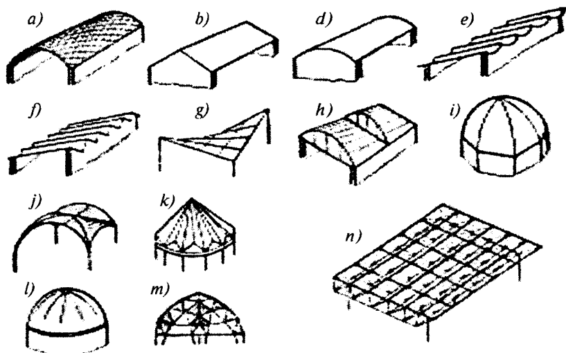
10.2- rasm. Zamonaviy fazoviy yog'och konstruksiyalarining asosiy ko'rinishlari:
