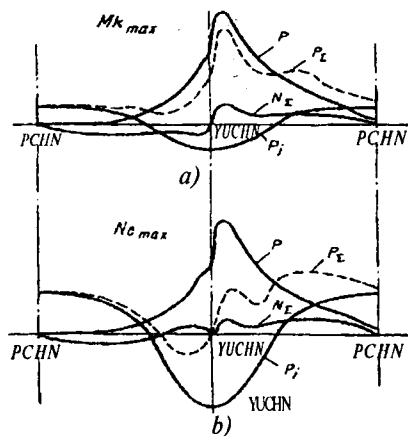
1.14-rasm. Eng yuqori burovchi moment (a) va eng yuqori quvvat-dagi (b) rejimlarda porshenga ta'sir qiluvchi kuchlar.
