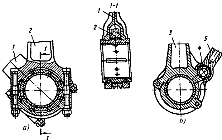
6.2-rasm. Bo'g'inlangan shatunlar konstruksiyasi: a – markaziy bo'g'inlanish, b – tirkama shatunli. 1 – ayri shatun; 2 – ichki shatun; 3 – asosiy shatun; 4 – tirkama shatunning asosiy shatun bilan bo'g'inlash barmog'i; 5 – tirkama shatun.
