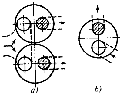
9.2-rasm. Bir silindrga ikki klapani ikki qator joylashtirish (a, b).
