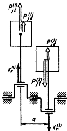
2.2-rasm. Ko'p silindrlı dvigatellarning muvozanatlanmaganligini keltirib chiqaradigan kuch omillarining tahliliga.
