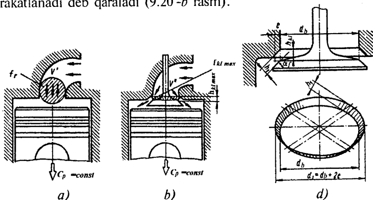
9.20-rasm. Gaz oqimining o'rtacha shartli tezliklarini aniqlashga:
