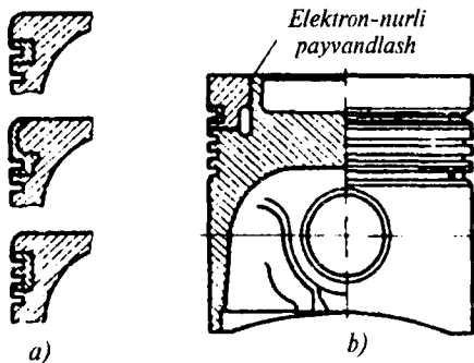
5.10-rasm. Porshen halqalarining yeyilishga qarshi kirgizmalari:
