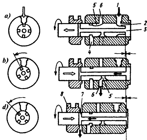
5.19-rasm. Bir plunjnerli taqsimlash nasos seksiyasining ishlash sxemasi.
