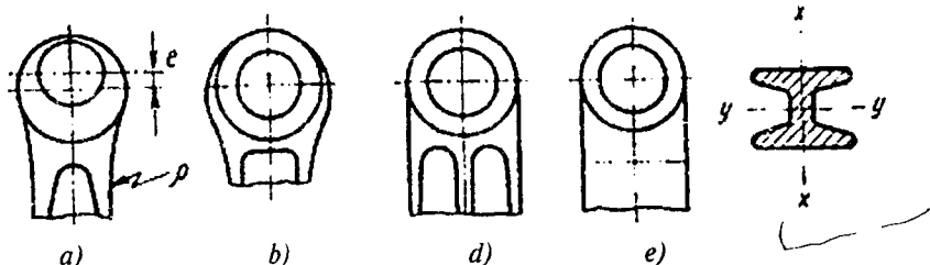
6.4-rasm. Porshen kallagini mustahkamlashga konstruktiv misollar:
