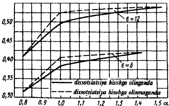
2.20-rasm. Hisoblangan siklning FIK ni havoning ortiqlik koeffitsiyentiga bog'liqlik grafigi.
