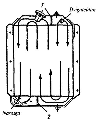
11.10-rasm. Uch yo'lli radiatorlarda sovitish suyuqligining harakatlanish sxemasi: 1 va 2—radiatorning mos holda yuqori va quyi baklaridagi to'siqlari.
