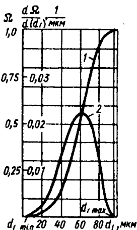
3.29-rasm. To'zitishning yig'indi egri chizig'i va chastotalar egri chizig'i.
