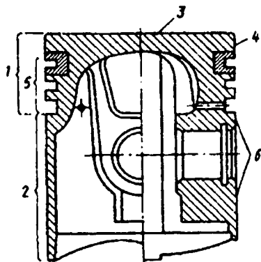
5.1-rasm. Porshenning asosiy elementlari.
