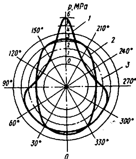
5.17-rasm. Aylana boʻyicha silindr koʻzgusiga halqa radial bosimining epyurasi: 1 – noksimon; 2 – tuxumsimon; 3 – oʻrtacha radial bosim.
