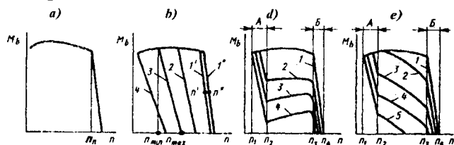
5.39-rasm. Turli rostlagichlar bilan jihozlangan dvigatellarning tezlik tavsiflari: a — chegaraviy eng yuqori aylanishlar chastotasini cheklovchi rostlagich; b — barcha rejimli rostlagich; d — ikki rejimli rostlagich; e — tezlik tavsifi yassiroq kechadigan barcha rejimli rostlagich.
