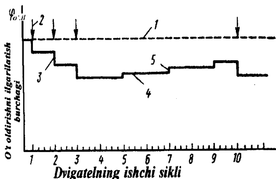
7.26-rasm. To'rt silindrli dvigatelning silindrlaridan biridagi detonatsiyani yo'qotish konturining ishlash
