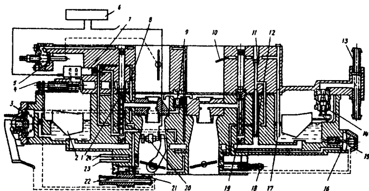
5.9-rasm. VAZ-2108 karbyuratorining konstruktiv sxemasi.
