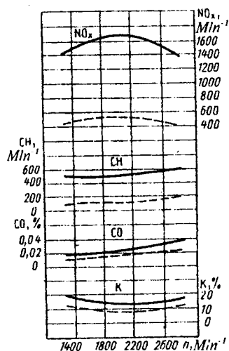
6.11-rasm. Dvigatellar IG ning tutab chiqishi va zaharililigi:
