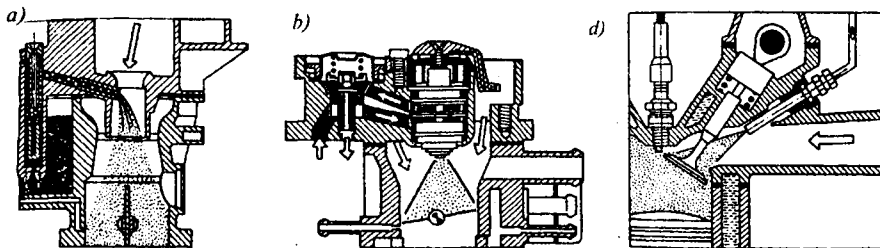
3.17-rasm. Karbyuratsiyalashda (a), markaziy (b) va taqsimlanish bilan (d) purkashda yonilg'i uzatish.
