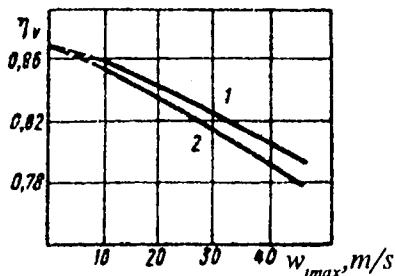
3.37-rasm. To'ldirish koeffitsiyenti va zaryadning harakat tezligini tangensial tashkil etuvchisini eng yuqori qiymati orasidagi o'zaro
