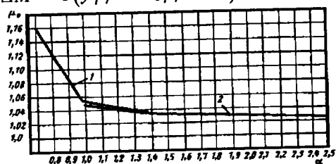
2.2-rasm. Molekular o'zgarish kimyoviy koeffitsiyentining havoni ortiqlik koeffitsiyenti \alpha ga bog'liqligi:
