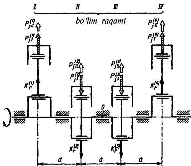
2.13-rasm. To'rt silindrli dvigatelda tirsakli val va inersiya kuchlarining ta'sir qilish sxemasi.
