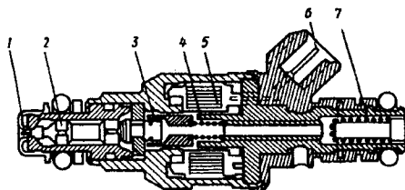
5.11-rasm. Elektromagnit forsunka.
