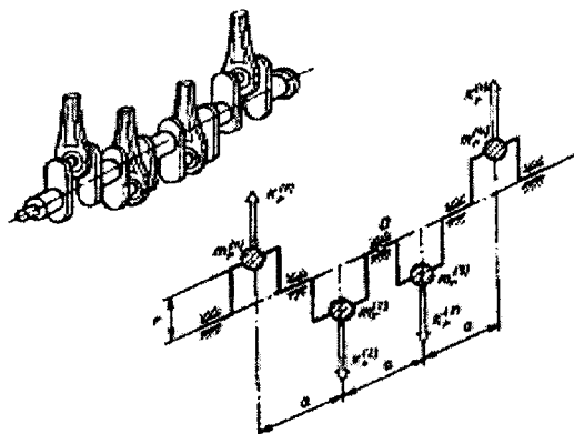
2.6-rasm. To'rt taktli to'rt silindrli bir qatorli dvigatelning o'zi muvozanatlanadigan tirsakli vali.
