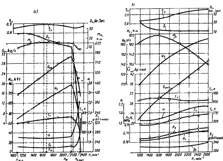
7.14-rasm. Tashqi tezlik tavsiflari:
