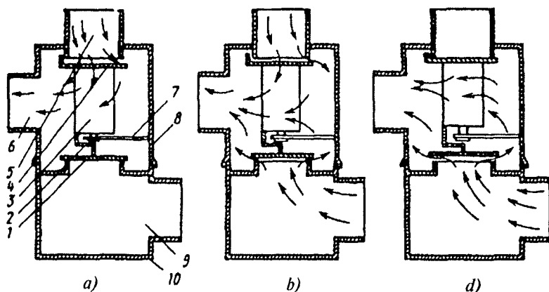
11.3-rasm. Termostatning ishlash sxemasi:
