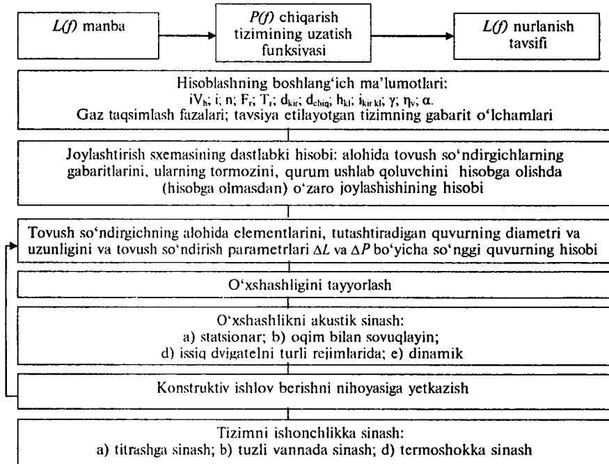
13.5-rasm. Ishlatilgan gazlar chiqarish tizimi va shovqin soʻndirgich hisobining prinsipial sxemasi.
