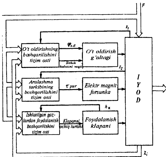
7.25-rasm. IYOD kompleks boshqarish tizimi ishlashining blok-sxemasini:
