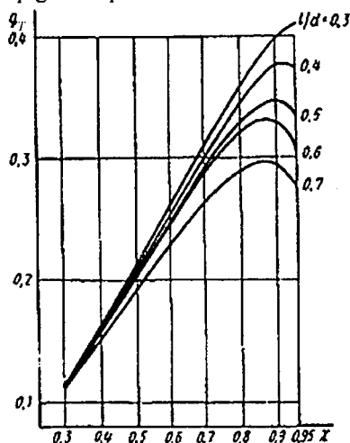
10.4-rasm. Yuklangan qismi orqali sarflash koeffitsiyentining eksentrisitetga bog'liqlik grafiqi.
