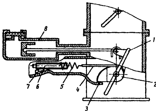
5.6-rasm. Eng yuqori aylanishlar chastotasining pnevmatik cheklagich sxemasi.
