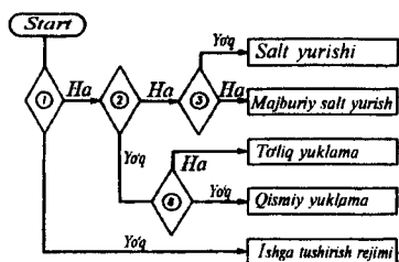
7.28-rasm. Dvigatel ish rejimini indifikasiyalash algoritmining sxemasi:
