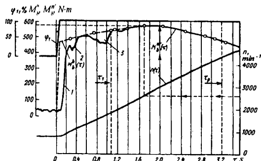
7.21-rasm. Karbyuratorning birlamchi kamerasi DTQ ni tez ochish bilan amalga oshirilishida karbyuratorli dvigatelning tezlashish jarayoni.
