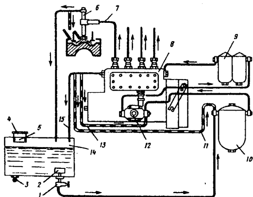
5.14-rasm. Ajratilgan turdagi yonilg'i tizimining sxemasi (uzluksiz chiziq 15 va uzilgan chiziq 11 va 13 lar bilan yuqori bosimli nasosdan ortiqcha yonilg'ini olib ketish sxemalari keltirilgan):
