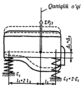
2.24-rasm. Osmaning bikrlilik o'qi x ni joylashtirish sxemasi.
