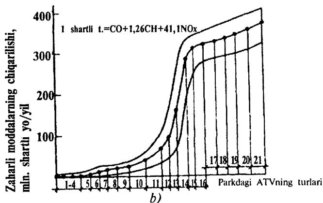
16.1-rasm. Sobiq SSSR da avtotransport vositasi parkining tarkibi (70-yillar boshlarida) (a) va avtomobil transporti orqali atmosferaga me'yorlanadigan zararli moddalarining chiqarib tashlanishi (b).
