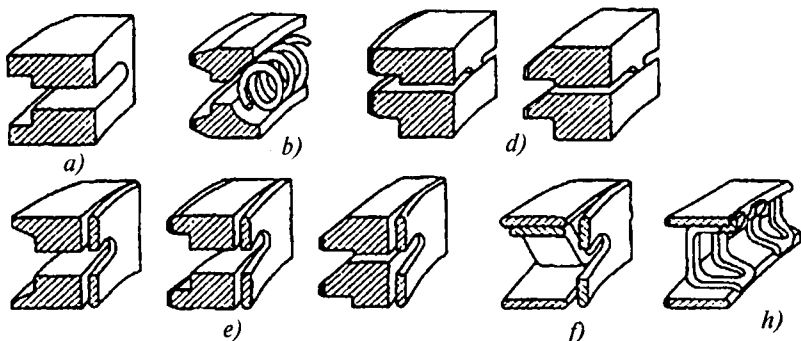
5.16-rasm. Moy sidiruvchi halqalarning asosiy konstruktiv yechimlari: a – kengaytirgichsiz qutisimon turdagi; b – oʻralgan prujina kengaytirgichli qutisimon turdagi; d – ikki qirgʻichli halqa; e – radial kengaytirgichli qutisimon turdagi; f – radial va oʻq boʻyicha kengaytirgichli; h – tangensial kengaytirgichli.
