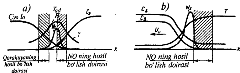
3.16-rasm. Diffuzion alanga ko'lamini (a) va bir jinsli aralashmada tarqaladigan alanga ko'lamini (b) tuzilishi.
