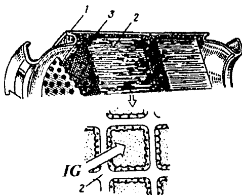
13.6-rasm. Katalitik neytrallagichning tuzilishi.
