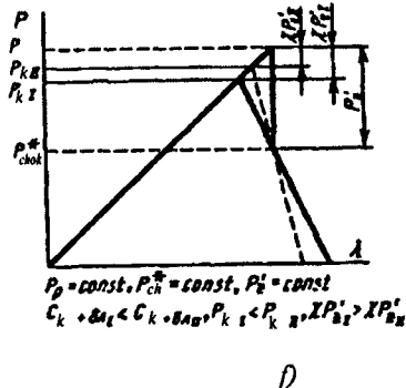
4.9-rasm. Dvigatel kuch sxemalari elementlarining ishonchligini baholashga: a – hisoblash sxemasi; b – tortishda kuch sxemasining deformatsiyasi; d – kuch diagrammasi-deformatsiya; e, f – kuch sxemasi detallari bikrligi nisbatlarining variantlari.
