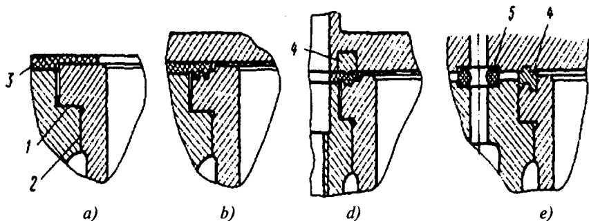
4.6-rasm. Gaz sizadigan choklarni zichlash:
