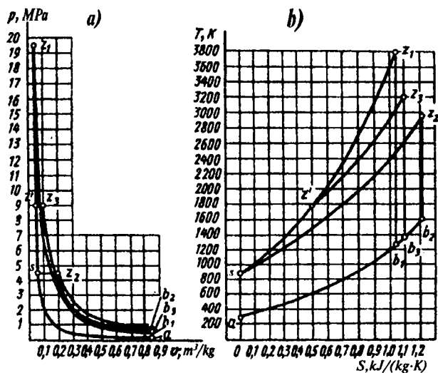
2.9-rasm. Otto, Dizel va Sabate-Trinkler sikllarini q_1 , \varepsilon = \text{idem} bo'lganda p - V (a) va T - s (b) koordinatalarda taqqoslash grafiqi.
