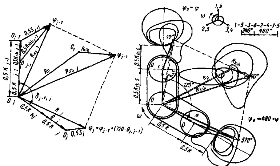
1.11-rasm. O'zak bo'yinga yuklamaning qutb diagrammasini qurish (olti silindrli to'rt taktli dvigatelning oltinchi o'zak bo'yni).
