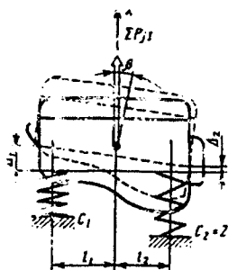
2.23-rasm. Ulangan tebranishlarning paydo bo'lish sxemasi.
