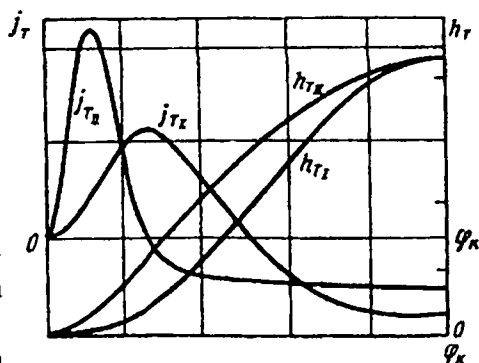
9.25-rasm. Polinom darajasi ko'rsatkichlari to'plami turlicha bo'lgan «polidayn» usuli bo'yicha profilangan kulachok turtkichining ko'tarilish h_T va tezlanish j_T grafigi:
