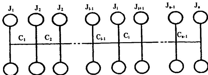
8.3-rasm. Umumlashgan koordinatasi n bo'lgan ekvivalent buralma tizim.
