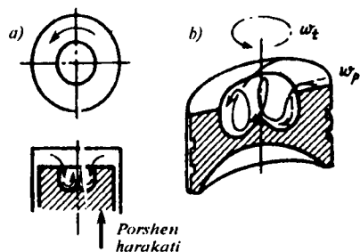
3.36-rasm. Zaryadning yonish kamerasiga oqib o'tishi va harakati sxemasi:
