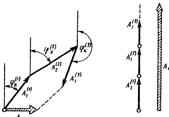
a) 8.8-rasm. Amplitudalarning vektorli diagrammalari (a,b).
