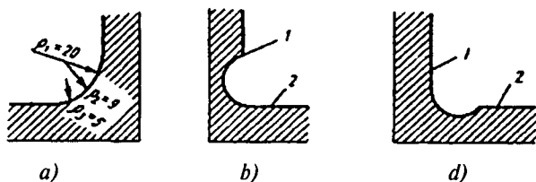
7.6-rasm. Galtellarning shakllari:
