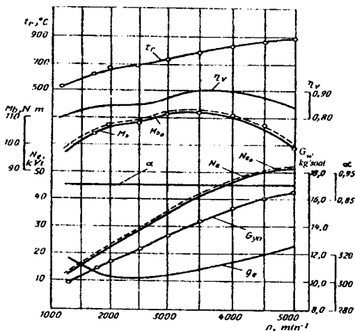
7.11-rasm. Yengil avtomobil karbyuratorli dvigatelining tashqi tezlik tavsifi: iV_h = 1,5l .
