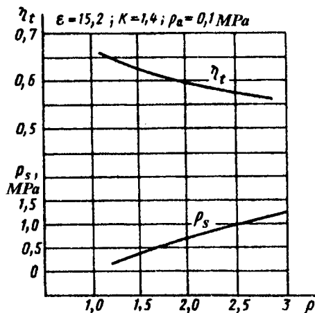
2.7-rasm. Dizelning termodinamik sikli ko'rsatkichlarini dastlabki kengayish darajasiga bog'liqlik chiziqli tasviri.
