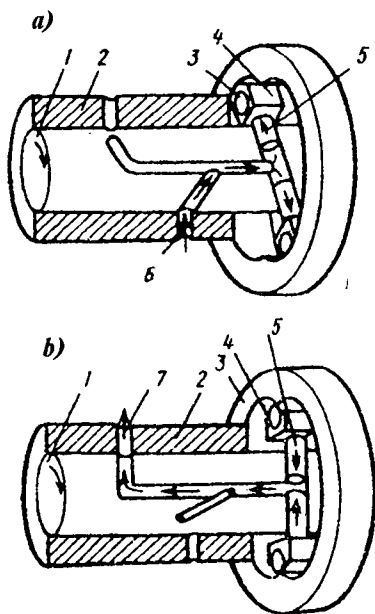
5.20-rasm. Rotorli taqsimlash nasosi.
