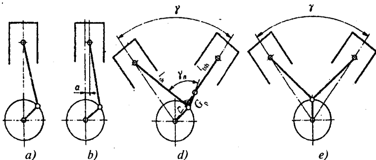
1.1-rasm. KSHM kinematik sxemalari:
