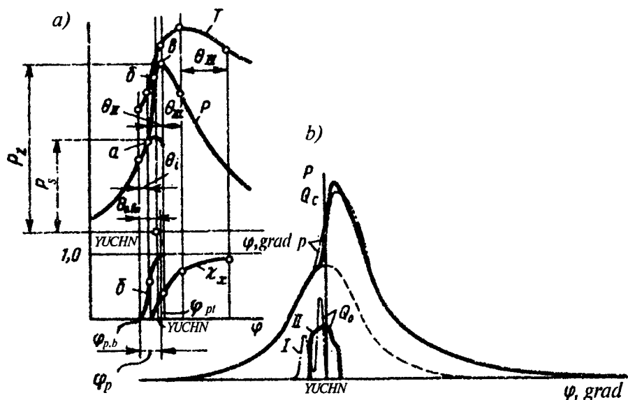
3.41-rasm. Indikator diagrammasi va issiqlikni kiritish d
