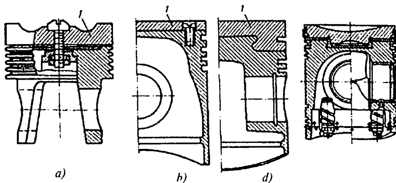
5.12-rasm. Tarkibli porshenlarning birikish variantlari: a – markaziy bolt bilan; b – periferiysi bo'yicha vintlar bilan; d – maxsus bobishkalar bilan.
