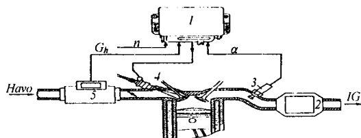
6.10-rasm. Kislorod datchigi ishorasi (signali) bo'yicha yonilg'i uzatishni boshqarish ( \alpha = 1,0 ): 1 — boshqarishning elektron bloki; 2 — uchta tashkil etuvchili katalitik neytrallagich; 3 \lambda — zond; 4 — elektr magnit forsunka; 5 — havo sarfini o'lchagich.
