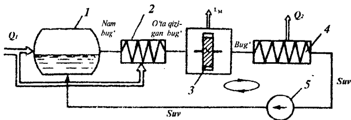
1.1-rasm. Bug' dvigatelining sxemasi:
