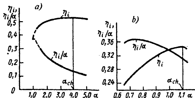
4.1-rasm. Dizel (a) va uchqundan o't oldiriladigan dvigatel (b) uchun \eta_i va \eta_i / \alpha larning havoning ortiqlik koeffitsiyentiga bog'liqligi.
