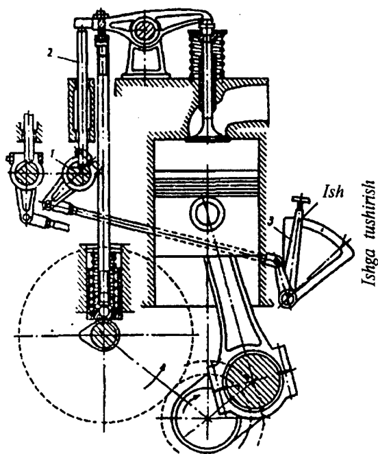
14.7-rasm. Dekompressor mexanizmlı gaz taqsimlash mexanizmining sxemasi.
