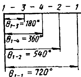
1.13-rasm. To'rt taktli dvigatelning yig'indi burovchi momentining shakllanish sxemasi: a – ayrim krivoshiplargata'sir qiluvchi momentlar sxemasi; b – yig'indi burovchi momentni qurish sxemasi.
