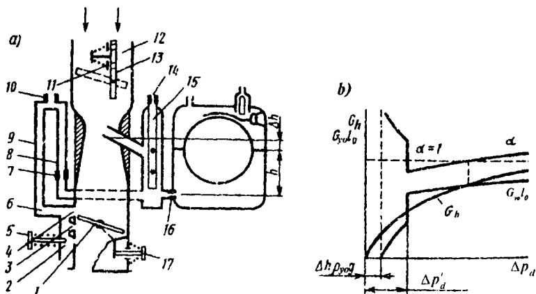
5.4-rasm. Jiklyorda siyraklanish pasayadigan karbyuratorning sxemasi (a) va bosh tizimi tavsifi (b).
