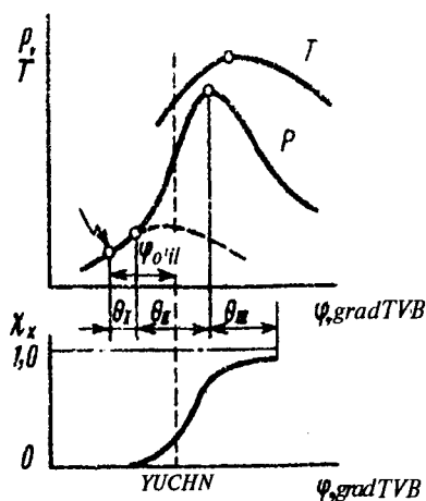
3.19-rasm. Uchqundan o't oldiriladigan dvigatelnining indikator diagrammasi ( \varphi_{o'II} — o't oldirishni ilgarilash burchagi, \theta_I , \theta_{II} , \theta_{III} — yonish jarayoni fazalari). \chi_x — issiqlik ajralib chiqish koeffitsiyenti.
