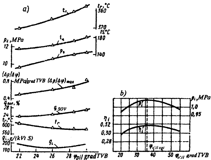
4.2-rasm. Ilgarilatish burchagi bo'yicha tavsiflar: a — purkash (dizel); b — o't oldirish (benzinli dvigatel).
