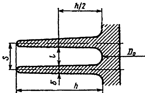
11.19-rasm. Trapetsiyasimon sovitish qovurg'asi.
