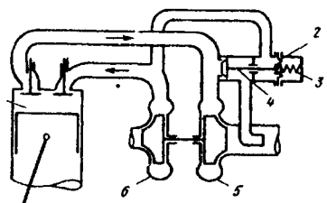
5.33-rasm. Gazni o'tkazib yuborish sxemasi: 1 — silindr; 2 — membrana; 3 — prujina; 4 — o'tkazib yuboruvchi klapan; 5 — turbina; 6 — kompressor.
