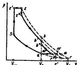
2.24-rasm. p—V koordinatalarda issiqlik aralash usulda beriladigan sikl.
