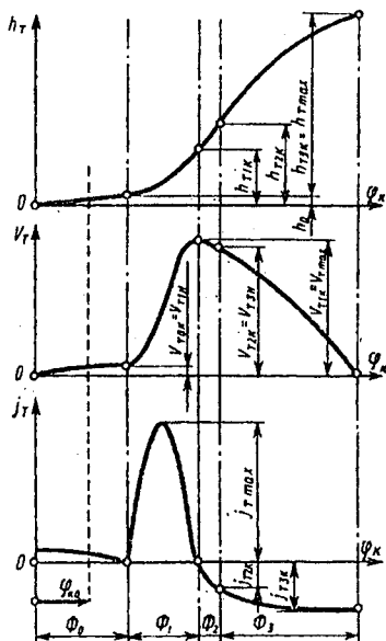
9.24-rasm. Kurs usuli bo'yicha profillangan kulachok ko'tarilishi h_T , tezligi v_T va tezlanishi j_T ning grafifi.
