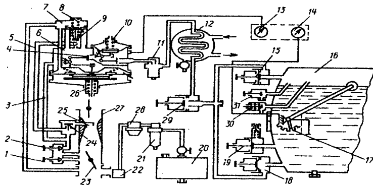
5.12-rasm. Suyuqlantirilgan gaz bilan ta'minlash tizimi sxemasi:
