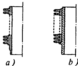
4.8-rasm. Havo bilan sovitiladigan IYOD ning silindrlari: a — monometalli; b — bimetalli.
