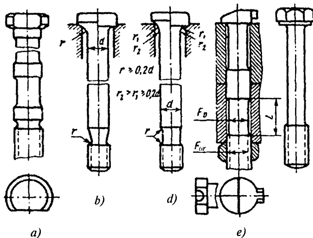
6.6-rasm. Vertikal kesimli kallagi nosimmetrik shaklli (a), tayanch sathi kamaytirilgan kallakli (b) bolt kallagining va uning shatundagi o'rnashadigan joyiga kontaktli sferik sathli (d), o'rnatuvchi elementli (e) bo'lgan shatun boltlarining konstruksiyalari.
