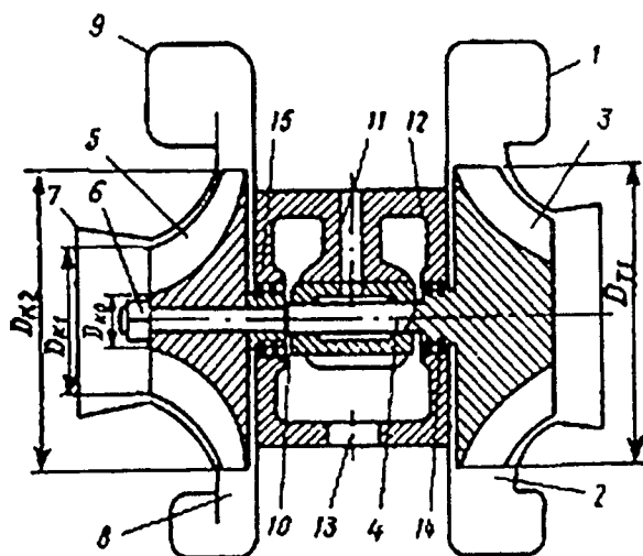
12.4-rasm. Turbokompressorning sxemasi.
