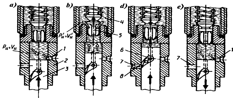
5.15-rasm. Yuqori bosimli nasos seksiyasining ishlash sxemasi (a...e).
