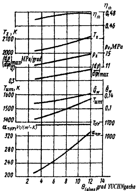
2.15-rasm. Hisoblangan sikl ko'rsatkichlarini alanganlanishni ilgariyatish burchagiga bog'liqlik chiziqli tasviri.
