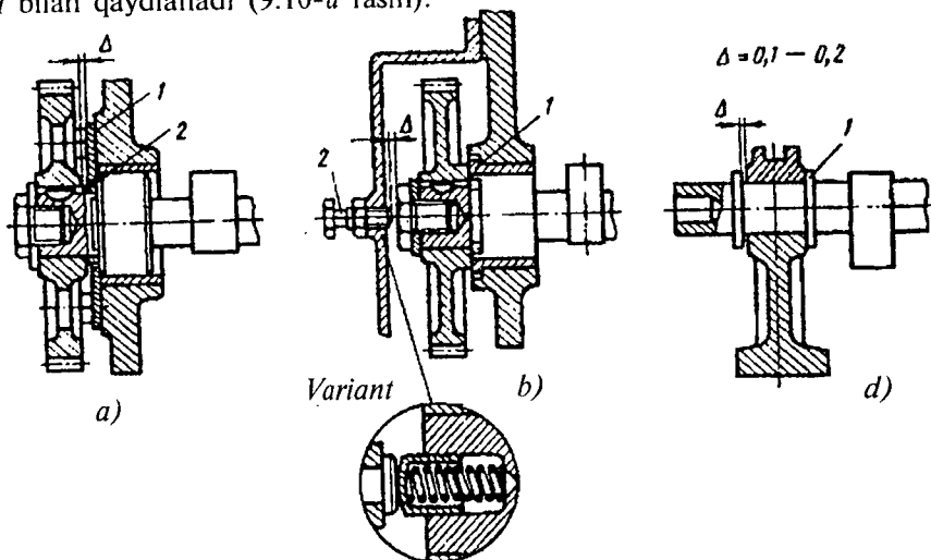
9.10-rasm. Taqsimlash valining o'q chizig'i bo'ylab siljishini qaydlash: a – bronza tirak flanes bilan; b – podshipnikning aylana chiqig'i va rostlash bolti bilan; d – aylana chiqiqlar bilan.
