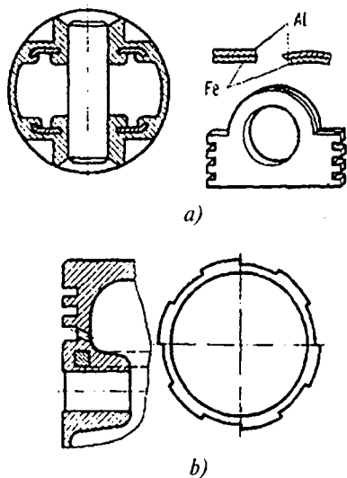
5.9-rasm. Porshenlarning termorostlagichli kirgizmalari:
