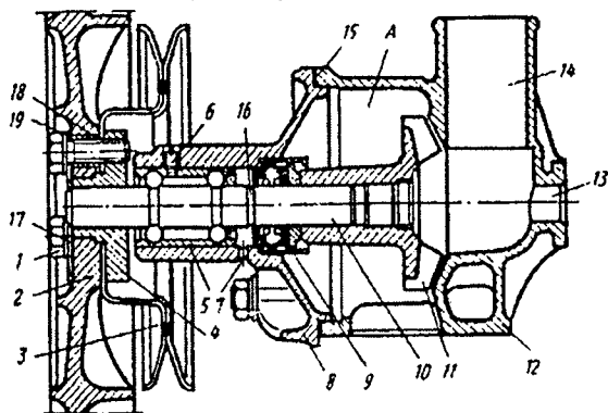
11.12-rasm. Dvigatelning suyuqlik nasosi:
