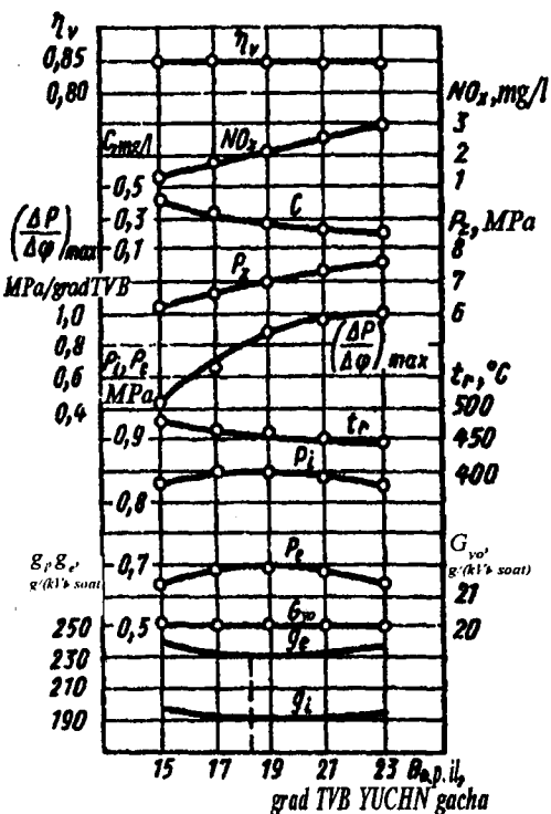
7.7.-rasm. Dizelning yonilg'i purkashni ilgarilatish burchagi bo'yicha roslash tavsifi.
