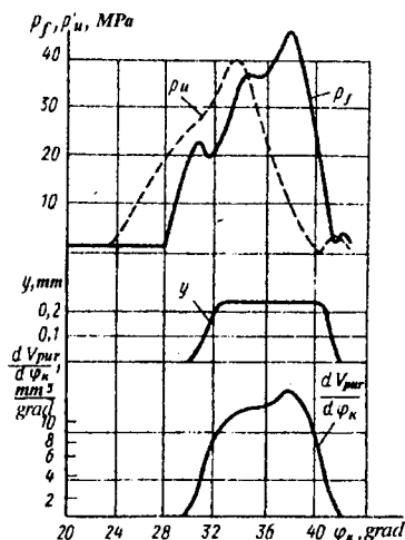
5.28-rasm. Yonilg'i tizimining gidrodinamik hisobi natijalari.
