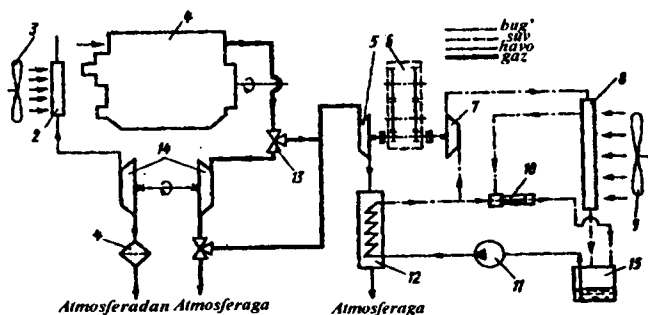
2.21-rasm. Kompaundli kuch qurilmasining prinsipial sxemasi:
