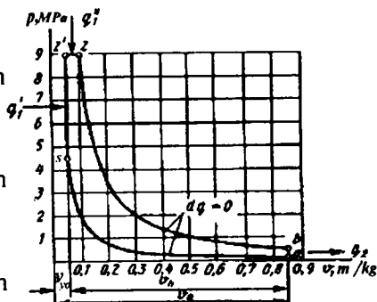
2.3-rasm. Issiqlik aralash usulda beriladigan sikl (Sabate-Trinkler sikli).
