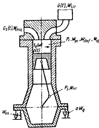
6.17-rasm. Dvigatel konstruksiyasini ideallashtirish va akustik nurlanishning paydo bo'lishi.
