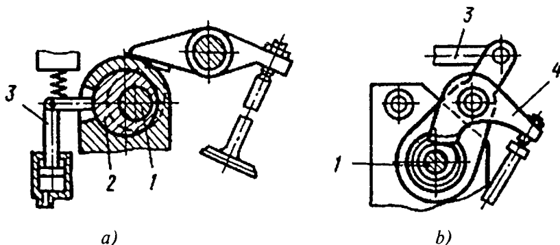
9.9-rasm. Rostlanadigan fazali gaz taqsimlash mexanizmlari.
