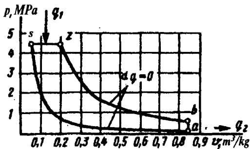
2.5-rasm. Issiqlik o'zgarish bosimda beriladigan sikl (Dizel sikli).
