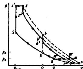
2.27-rasm. Ishchi jismni dastlabki siqish bilan p—V koordinatalardagi sikli.
