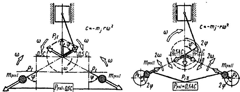
2.12-rasm. Qaytma-ilgarilanma harakatlanuvchi massalar inersiya kuchlarini muvozanatlash mexanizmining sxemasi: a - P_{II} birinchi tartibli; b - P_{III} ikkinchi tartibli.
