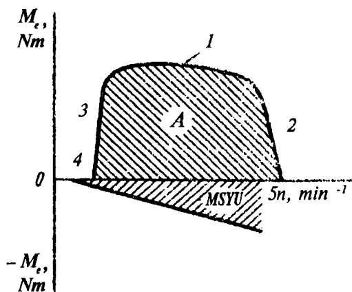
1.11-rasm. Avtomobil dvigateli ishlashining yuklama va tezlik rejimlari maydoni.
