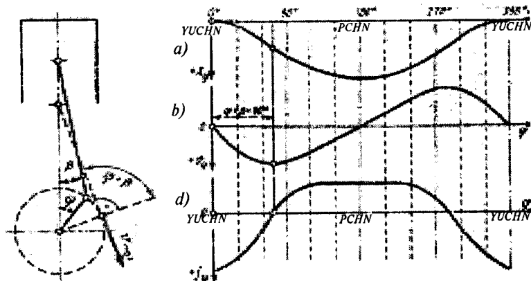
1.3-rasm. Porshenning kinematik parametrlari:
