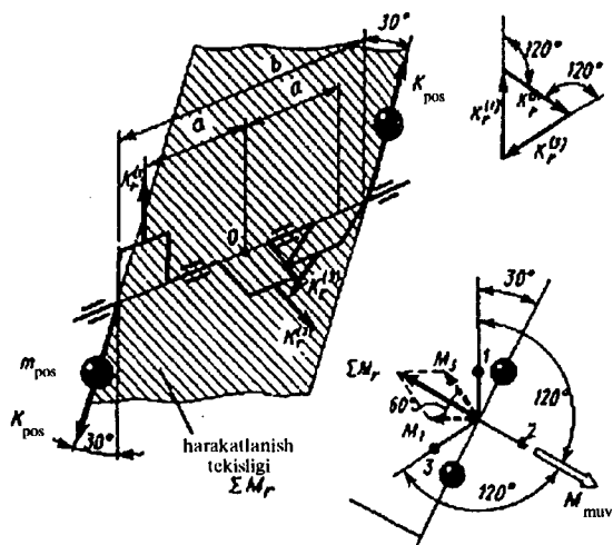
2.8-rasm. \delta = 120^\circ burchak ostida bo'lgan uch krivoshipli fazoviy tirsakli valni muvozanatlash.
