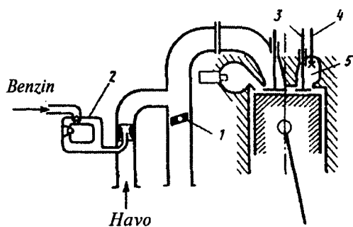
14.6-rasm. Dizelni benzinda ishga tushirish tuzilmasining sxemasi.
