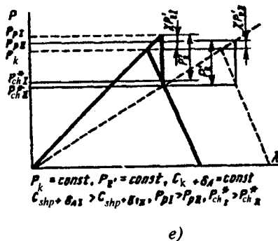
4.9-rasm. Dvigatel kuch sxemalari elementlarining ishonchligini baholashga: a – hisoblash sxemasi; b – tortishda kuch sxemasining deformatsiyasi; d – kuch diagrammasi-deformatsiya; e, f – kuch sxemasi detallari bikrligi nisbatlarining variantlari.
