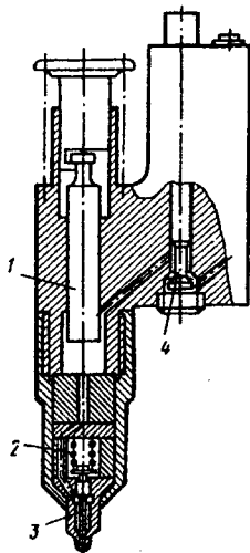
5.24-rasm. Mexanik yuritmal va dozlashni hamda purkashni ilgarilatish burchagini elektron boshqaradigan nasos-forsunka:
