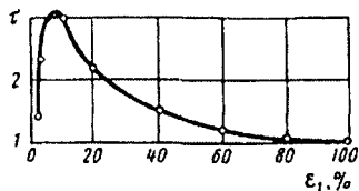
12.2-rasm. Ikki bosqichli havo tozalagich ishlashining nisbiy vaqti \tau ning birinchi bosqichni o'tkazib yuborish ko'effitsiyenti \varepsilon_1 ga bog'liqligi.
