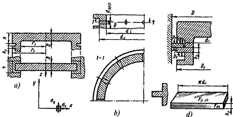
5.19-rasm. Porshen elementlarini hisoblash modeli:
