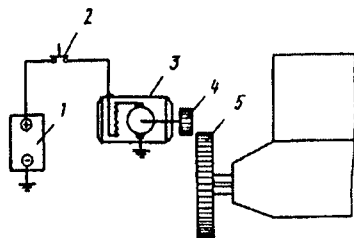
14.1-rasm. Dvigatelni elektr startyor bilan ishga tushirish sxemasi.
