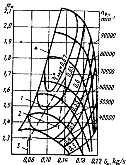
12.5-rasm. Kompresorning tavsifi.
