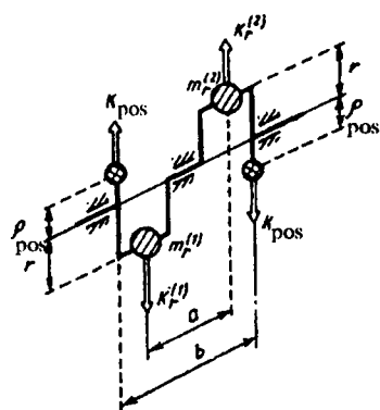
2.4-rasm. \delta=180^\circ bo'lgan bir qatorli ikki silindrlı dvigatelning tirsakli valini muvozanatlash.
