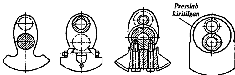
7.7-rasm. Tirsakli valning jag‘i va posangilarining shakli.
