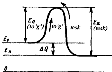
3.10-rasm. To'g'ri va teskari reaksiyalarning aktivatsiya energiyasi E_a va issiqlik samarasi \Delta Q .
