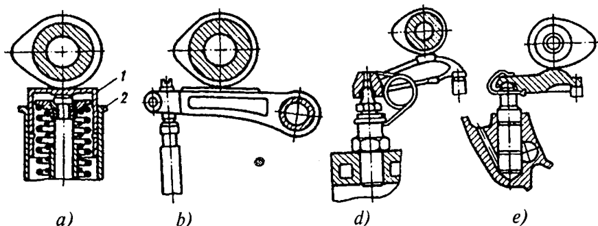
9.17-rasm. Taqsimlash vali yuqorida joylashganda klapanlarning yuritmasi ( a, b, d, e ).
