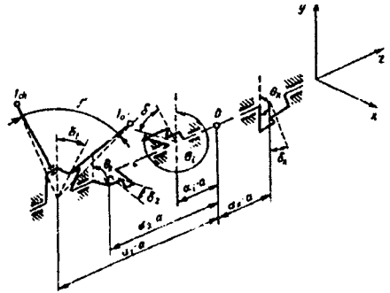
2.16-rasm. Yagona algoritm bo'yicha dvigatelning muvozanatlanmaganligini hisoblash sxemasi.
