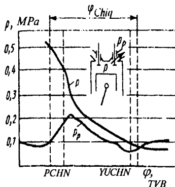
3.2-rasm. To'rt taktli dvigatelning chiqarish jarayoni- da p va p_p larning o'zgarishi: \varphi_{chiq} — chiqarish fazasi.
