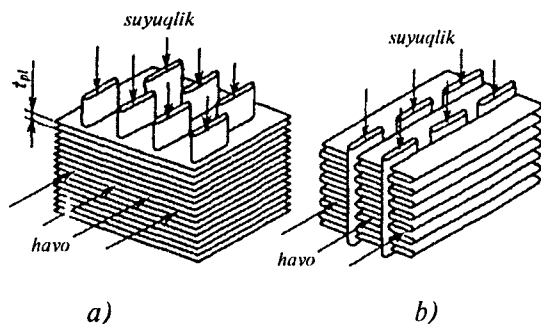
11.4-rasm. Radiator sovitish panjarasining o'zagi: a—naycha-plastinali; b—naycha-tasmali.
