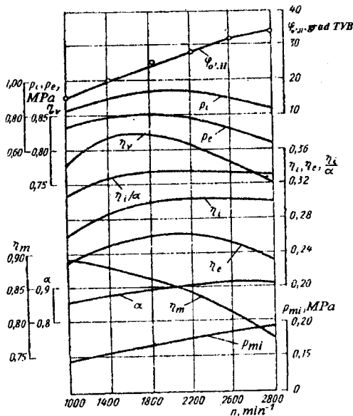
7.12-rasm. Yuk avtomobili karbyuratorli dvigateling tashqi tezlik tavsifi bo'yicha ishchi jarayoni asosiy ko'rsatkichlarining o'zgarishi: iV_h = 6,0 l.
