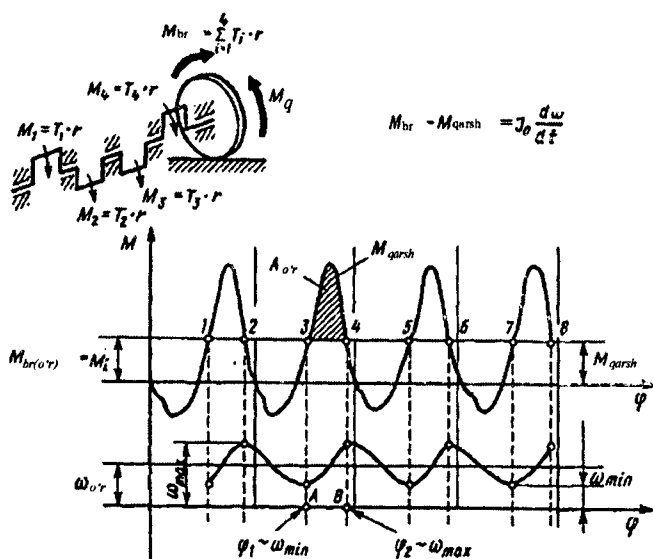
2.18-rasm. Barqaror ishlash rejimida to'rt silindrli dvigatel validagi momentlarning balansi.
