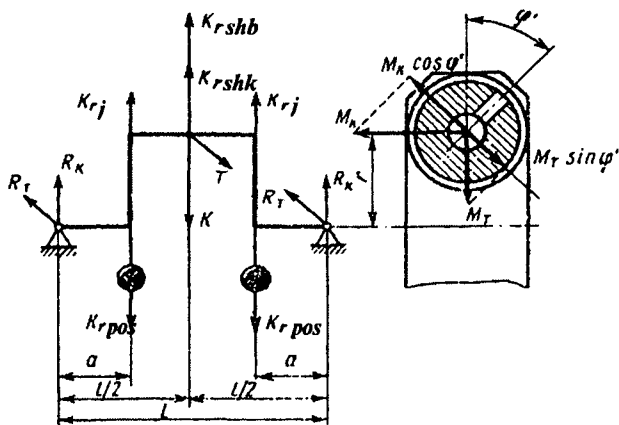
7.9-rasm. Krivoshipning hisoblash sxemasi.
