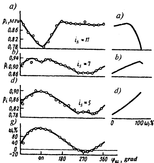
4.3-rasm. Yonilg'i uzatish va aylanishlar chastotasi o'zgarmas bo'lganda siqish jarayoni oxiridagi zaryad harakatining o'rtacha burchak tezligining o'rtacha indikator bosimga ta'siri: a, b, d — i_s 11, 7 va 5 larga teng bo'lganda ekranli klapaning burilish burchagiga mos holda p_i ni bog'liqligi; g — ekranli klapani burilish burchagiga foizda ifodalangan zaryad harakati burchak tezligini bog'liqligi; a', b', d' — i_s 11, 7 va 5 larga teng bo'lganda mos holda foizda ifodalangan zaryad harakatini burchak tezligiga p_i ni bog'liqligi.
