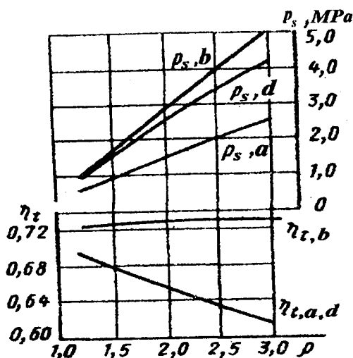
2.13-rasm. Termodinamik sikllar ko'rsatkichlarini dastlabki kengayish darajasiga bog'liqlik chiziqli tasviri: a sikl — porshenli dvigatel; b sikl — turbina oldidagi gazlar bosimi o'zgaruvchan bo'lgan kombinirlangan dvigatel; d sikl — turbina oldidagi gazlar bosimi o'zgarmas bo'lgan p_z , T_z = idem bo'lgan sharoitdagi kombinirlangan dvigatel. Havo bosimsiz beriladigan dvigatelni siqish darajasi \varepsilon kombinirlangan dvigatellarda \varepsilon_0 ga teng.
