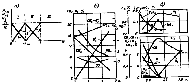
2.1-rasm. Yonish mahsulotlaridagi tashkil etuvchilar miqdorining \alpha ga bog'liqligi.
