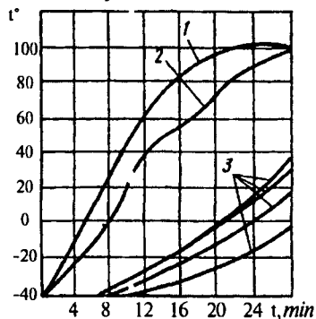
14.9-rasm. ZIL-375 dvigateli elementlari haroratining isitish vaqtiga bog'liqligi.
