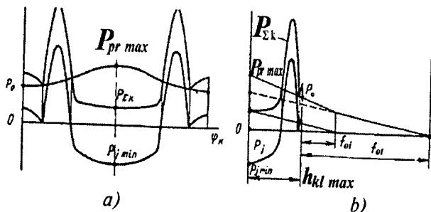
9.29-rasm. GTM da kuchlar o'zgarishining bog'liqligi: a - taqsimlash vali kulachogining burilish burchagiga nisbatan; b - klapan yo'lga nisbatan.
