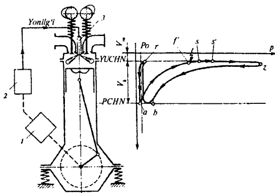
1.5-rasm. Dizelning sxemasi va indikator diagrammasi: 1 — reduktor; 2 — yuqori bosimli yonilg'i nasosi (YUBYON); 3 — forsunka.
