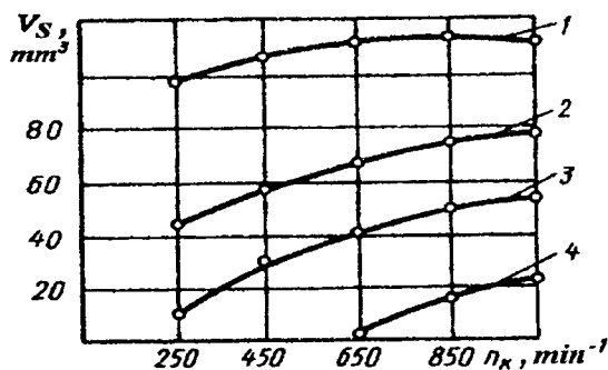
5.25-rasm. Reykaning turli to'rt holatida yonilg'i uzatishning tezlik tavsifi:
