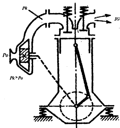
1.9-rasm. Yuritmalı kompressor orqali dvigatelga qo'shimcha havo kiritish sxemasi.
