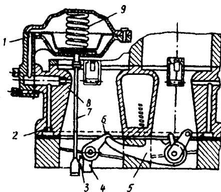
5.8-rasm. Ikkilamchi kamera drossel to'smaqopqog'ining pnevmatik yuritmasi.
