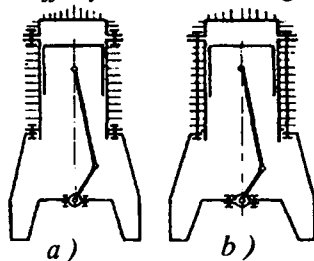
4.7-rasm. Havo bilan sovitiladigan IYOD ning kuch sxemalari: a — yuk ko'taruvchi silindrlri; b — yuk ko'taruvchi kuch shpilkali.
