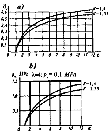
2.6-rasm. Ottoning termodinamik sikli ko'rsatkichlarini siqish darajasiga bog'liqlik chiziqli tasviri: a - \eta_i ; b - p_s .
