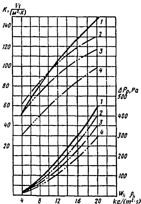
11.8-rasm. Havoning massali tezligiga bog'liq holda issiqlik uzatish koeffitsiyenti K va radiatorlarning aerodinamik qarshiligi P_r :
