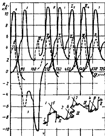
1.16-rasm. ZIL-130 dvigatelining tirsakli validagi o'zak podshipnigiga ta'sir qiluvchi kuchlar (drossel qopqog'i 100% ochiq holda, n=1000 \text{ min}^{-1} ).
