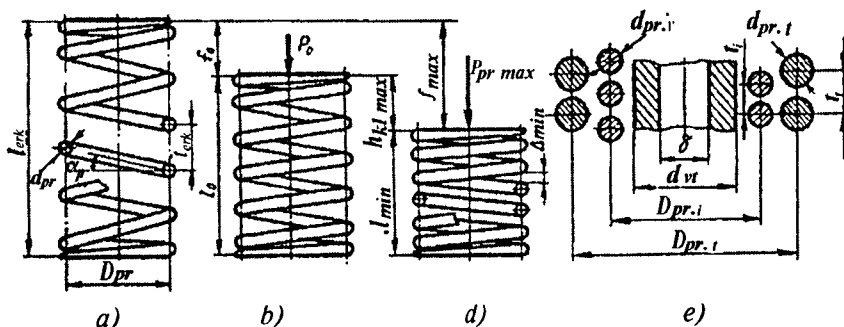
9.30-rasm. Klapan prujinalarining turli holatlarida uning geometrik parametrlari:
