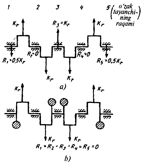
2.7-rasm. Bir qatorlı to'rt silindrlı dvigatelnıng o'zak tayanchlaridagi yuklama:
