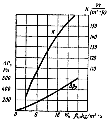
11.11-rasm. Sovitish havosi tezligining radiatorning K va \Delta p_p kattaliklariga ta'siri.
