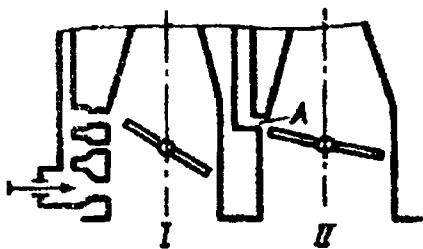
5.7-rasm. Drossel toʻsmaqopqoqlari ketma-ket ochiladigan ikki kamerali karbyuratorning prinsipial sxemasi: I va II — birlamchi va ikkilamchi kameralar.
