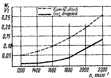
6.23-rasm. KamAZ dvigatellarining akustik quvvati.
