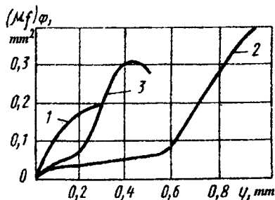
5.23-rasm. To'zitikchilarning gidravlik tavsiflari: 1 — ko'p oqimli; 2, 3 — shtiftli.
