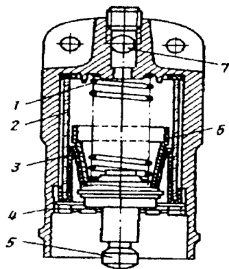
12.3-rasm. «Baxara» firmasining yo'l qo'yilgan (ruxsat etilgan) gidravlik qarshilikli indikator:
