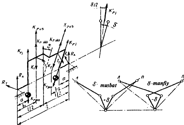
7.11-rasm. Siljilgan shatun boʻyinli krivoshipning hisobi uchun sxema.
