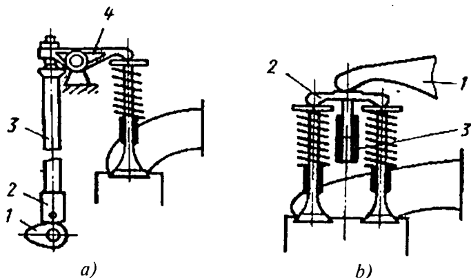
9.5-rasm. Taqsimlash valining quyi (a) va yoki o'rtada (b) joylashishi.
