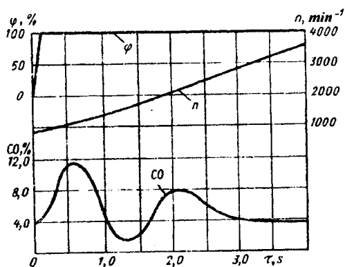
7.22- rasm. DTQ tez ochilishi keltirib chiqargan karbyuratorli dvigatelning tezlashish jarayonida IG dagi CO miqdorining o'zgarishi.
