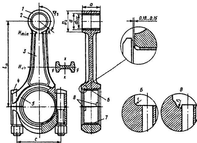
6.1-rasm. Yakka shatun konstruksiyasi:
