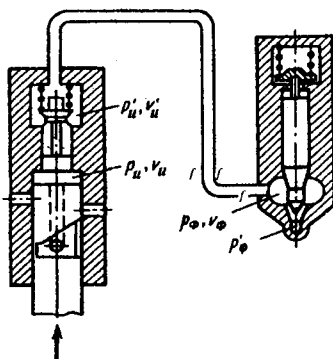
5.27-rasm. Yonilg'i tizimining hisoblash sxemasi.
