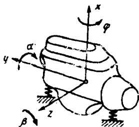
2.20-rasm. Amortizatsiya-langan dvigatel sxemasi.
