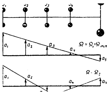
8.9-rasm. Besh massali tizim tebranishlarining birinchi va ikkinchi shakllari.
