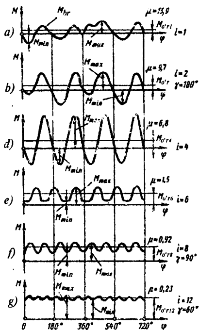
2.17-rasm. Silindrlar soni turlicha bo'lgan (a–g) to'rt taktli karbyuratorli dvigatellarning yig'indi buruvchi momentlari.
