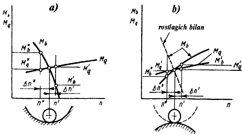
5.35-rasm. Yuklama ostida dvigatel ish rejimlarining barqarorligi: a — barqaror; b — beqaror (rostlagichsiz).
