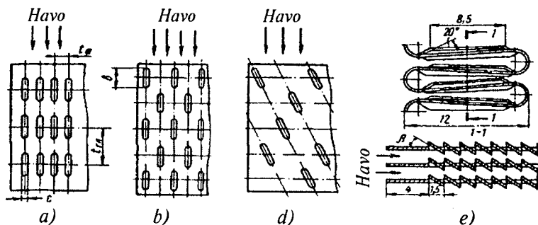
11.6-rasm. Naycha-plastinali radiatorlarning sovitish panjaralari elementlari:
