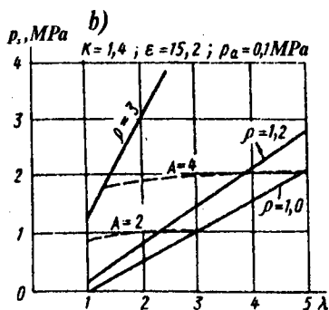
2.8-rasm. Sabate-Trinklar termodinamik sikli ko'rsatkichlarini bosimning ortish darajasiga bog'liqlik chiziqli tasviri:
