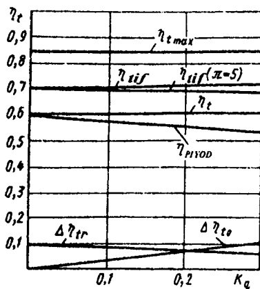
2.30-rasm. Termik FIK ni «issiqlik yo'qolish» koeffitsiyentiga bog'liqligi.
