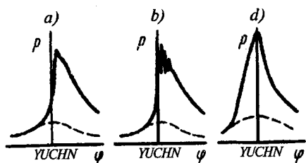
3.21-rasm. Uchqundan o't oldiriladigan dvigatel yonish jarayonini buzilishidagi indikator diagramma: a — kuchsiz detonatsiya; b — kuchli detonatsiya; d — barvaqt alangalanish.
