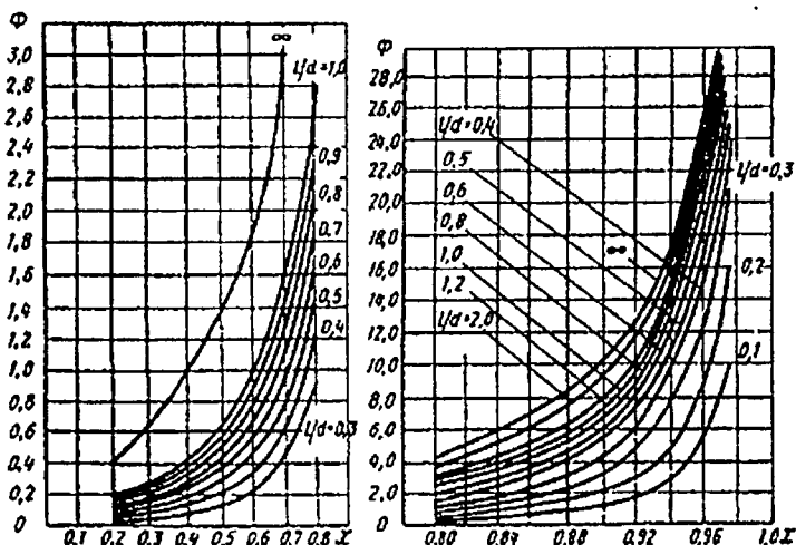
10.2-rasm. Yuklanganlik koeffitsiyentiga nisbiy eksentrisitetning bog'liqligi grafiqi.
