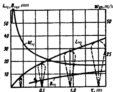
3.31-rasm. Vaqtga bog'liq holda oqimning geometrik ko'rsatkichlarini va uning oldingi ko'lamidagi tezligini o'zgarishi.
