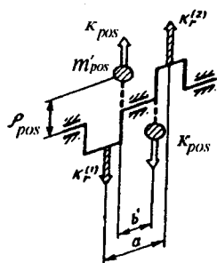
2.5-rasm. Bir qatorli ikki silindrli dvigatel valini muvozanatlash sxemasining varianti.
