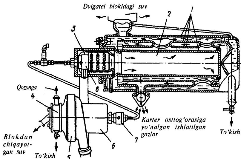
14.8-rasm. Ishga tushirishdan oldin dvigatelni suyuqlikli isitkichi.
