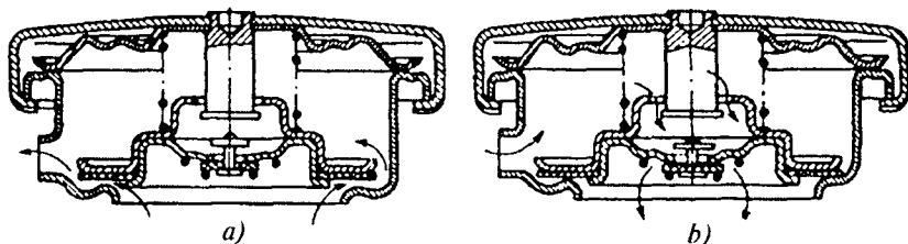
11.2-rasm. Klapan ochiq bo'lgan paytida kengayish baki kengaytirgich, kondensator, sovitish g'ilofidagi suyuqlik sathini stabilagichi va deaerator (sovitish suyuqligidan havo, gazlar va bug'ni ajratgich) vazifasini bajaradi. Bakning umumiy hajmi sovitish tizimining sig'imini 10...25% ga ega bo'lganida bug'-havo bo'shlig'ining hajmi, odatda, 5...7% ni tashkil etadi. Sovitish tizimining solishtirma hajmi yengil avtomobillar uchun 0,18...0,24 l/kVt ni, yuk avtomobillari uchun esa 0,25...0,34 l/kVt ni tashkil etadi.
