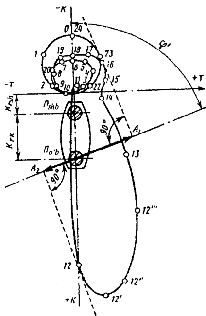
7.10-rasm. Shatun bo'yining egilishdagi hisob sxemasi.
