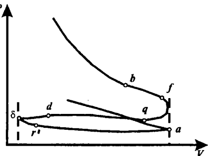
13.1-rasm. Ishlatilgan gazlarni chiqarib tashlashda shovqin hosil bo'lishining xarakterli uchastkalari bilan chizilgan indikator diagramma.
