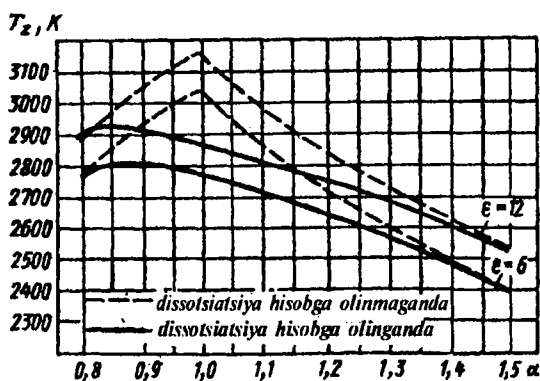
2.19-rasm. Siklning eng yuqori haroratini havoning ortiqlik koeffitsiyentiga bog'liqlik grafi.
