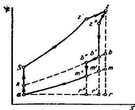
2.26-rasm. Ishchi jismni dastlabki siqish bilan T—S koordina- talardagi sikli.
