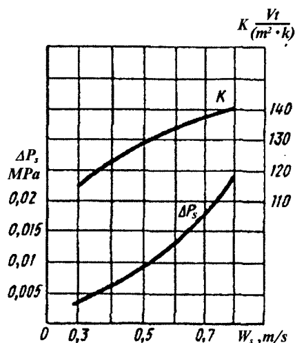
11.9-rasm. Sovitish suyuqligi tezligi radiatorning K va \Delta P_s lar qiymatlariga ta'siri.
