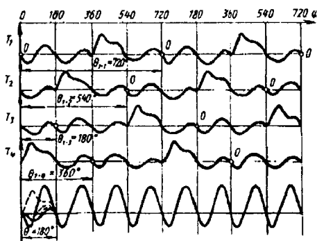
1.13-rasm. To'rt taktli dvigatelning yig'indi burovchi momentining shakllanish sxemasi: a – ayrim krivoshiplargata'sir qiluvchi momentlar sxemasi; b – yig'indi burovchi momentni qurish sxemasi.
