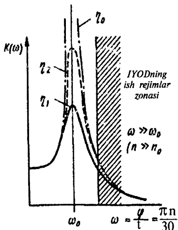
2.22-rasm. Erkinlik darajasi birga teng bo'lgan tizimning uzatish funksiyasining chastotali bog'liqligi ( \eta_1 > \eta_2 ).
