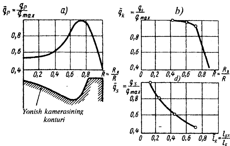
4.8-rasm. Dizel detallari bo'yicha issiqlik yuklamasining taqsimlanishi: a — porshen; b — silindr kallagi; d — silindr gilzasi; R_x — silindr o'qidan o'lchash doirasigacha bo'lgan oraliq R = D/2 ; l_{gx} — gilzaning yuqori qirrasidan o'lchash doirasigacha bo'lgan oraliq; l_g — gilza uzunligi.
