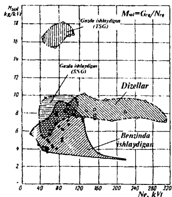
6.2-rasm. PIYOD solishtirma massasining quvvatga bog'liqligi.
