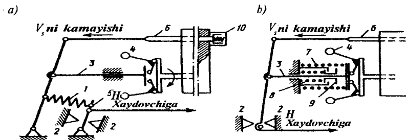
5.40-rasm. Rostlagichlarning sxemasi: a — barcha rejimli; b — ikki rejimli.
