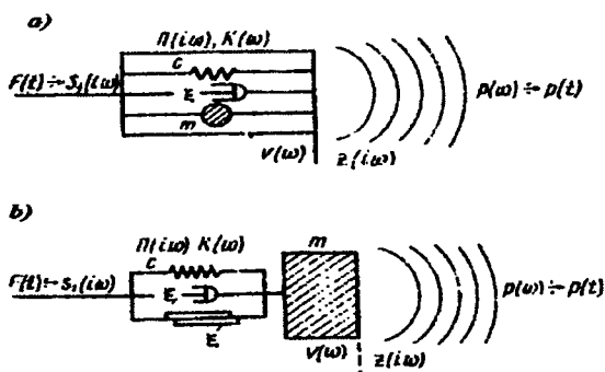
6.18-rasm. Dvigatel shovqini hosil bo'lishining oddiy sxemasi.
