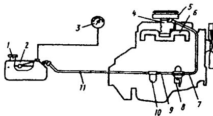
5.1-rasm. Karbyuratorli dvigatelning ta'minlash tizimi sxemasi.
