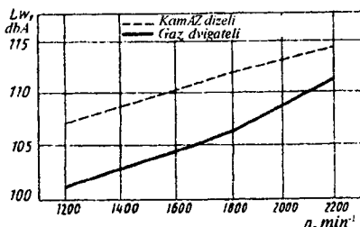
6.22-rasm. KamAZ dvigateli tovush quvvatining umumiy darajasi.
