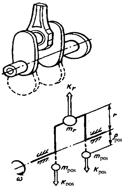
2.3-rasm. Bir silindrlı dvigatel valini muvozanatlash.
