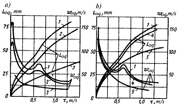
3.33-rasm. YAMZ-236 dizelining yonilg'i tizimini turli rejimlarda ishlashida oqimni oldingi ko'lamini tezligi w_{oq} ni va uzunligi L_{oq} ni o'zgarishi ( p_{pr} = 1,5 \text{ MPa} ):
