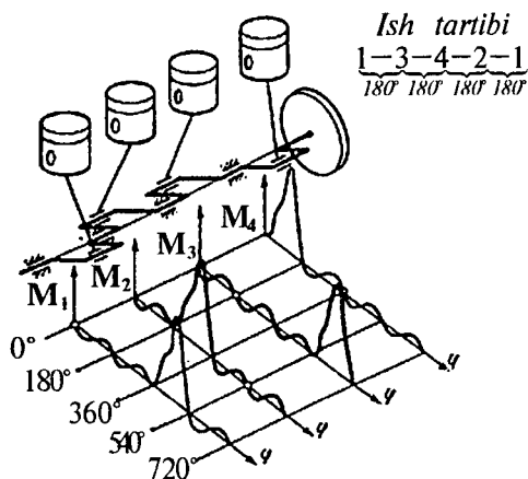
8.1-rasm. Tirsakli valning o'zgaruvchan momentlar bilan yuklanish sxemasi.
