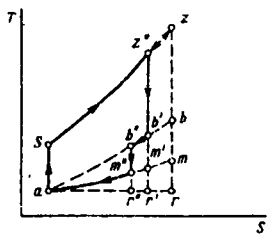
2.22-rasm. T—S koordinatalarda issiqlik o‘zgarmas hajmda beriladigan sikl.
