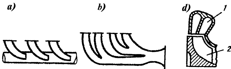
5.31-rasm. Impulslar o'zgartiruvchisi joylashtirilgan tizim: a, b — chiqarish kollektorida; d — turbina korpusida: 1 — turbina korpusi, 2 — ishchi g'ildirak.
