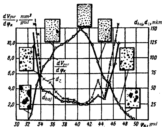
3.32-rasm. Purkash jarayonida yonilg'ining hajmiy uzatilishini va tomchilarning o'rtacha diametrining o'zgarishi.
