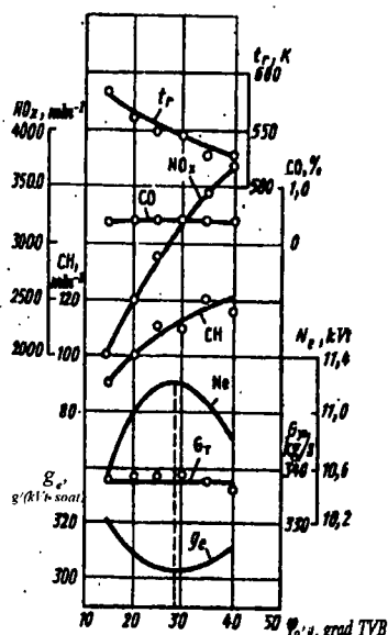
7.5.-rasm. O't oldirishning ilgariyatish burchagi bo'yicha rostlash tavsifi:
