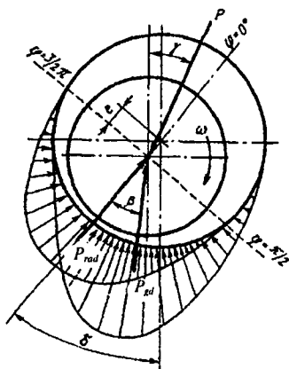
10.8-rasm. Sapfa markazi trayektoriyasini hisoblashga.
