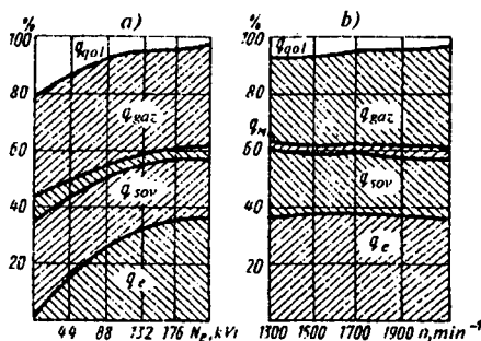
4.9-rasm. Gaz turbinali bosim ostida kiritishda avtotraktor dizelinig issiqlik balansi:
