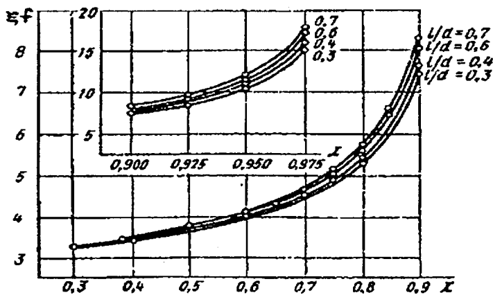
10.3-rasm. Aylanishga shipning qarshilik koeffitsiyentining eksentrisitetga bog'liqlik grafiqi.
