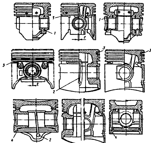
5.3-rasm. Uchqundan o't oldiriladigan dvigatellarning porshenlari:
