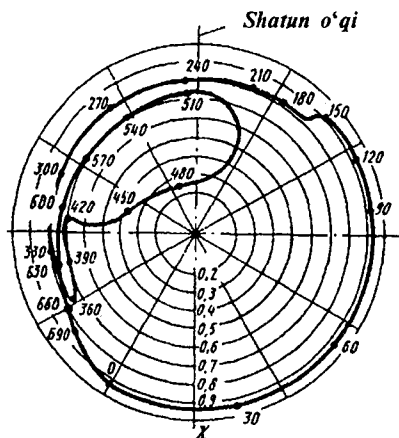
10.9-rasm. Shatun bo'yni markazining trayektoriyasi.
