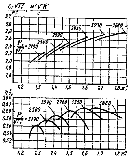
12.6-rasm. Turbinaning tavsifi.
