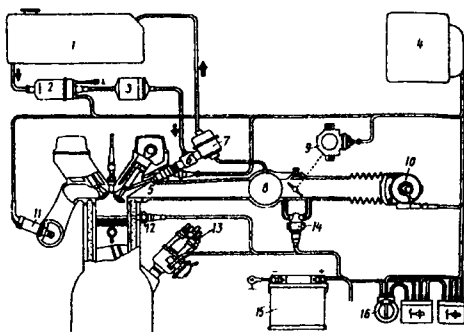
5.10-rasm. Benzinni purkab taqsimlash tizimining sxemasi.
