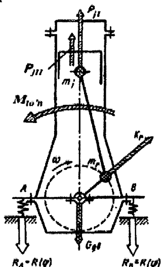
2.1-rasm. Bir silindrlı dvigatelning muvozanatlanmaganligini keltirib chiqaradigan kuch omillari.
