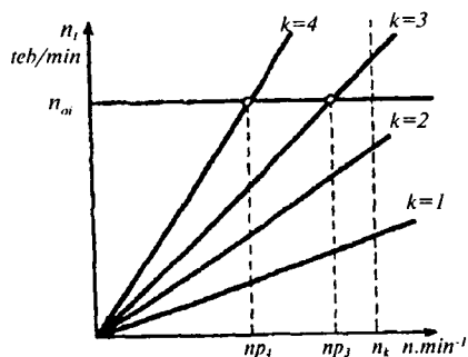
8.10-rasm. Dvigatel ishlashining rezonansli rejimlarini chastotaviy diagramma bo'yicha aniqlash.
