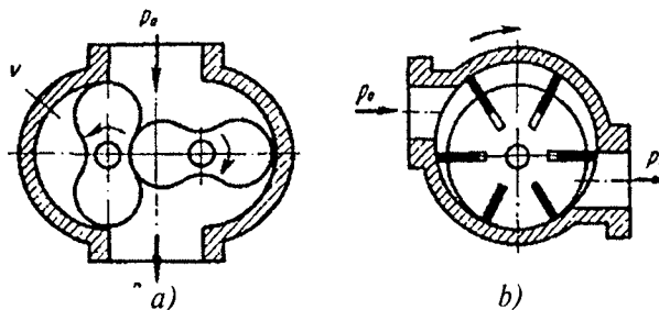
12.7-rasm. Hajmiy yuritmal kompressorlar: a – rotor-shesternali; b – rotor-plastinali.
