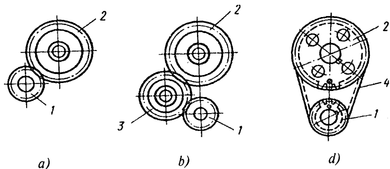
9.7-rasm. Quyidagilar yordamida quyi taqsimlash valiga yuritma:
