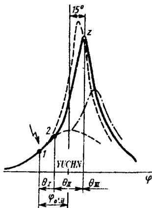
7.6-rasm. O't oldirishning eng maqbulida, ilgariroq bo'lishida va kechikishidagi indikator diagrammalar.
