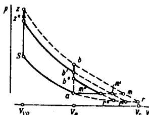
2.23-rasm. p—V koordinatalarda issiqlik o‘zgarmas hajmda beriladigan sikl.
