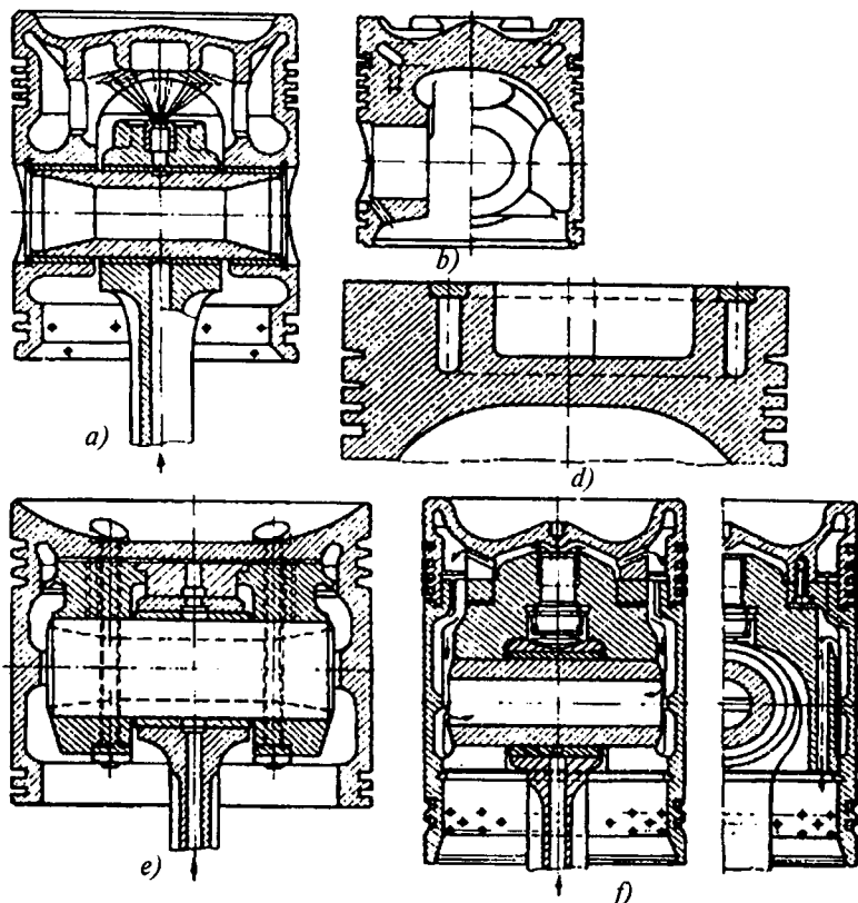
5.11-rasm. Majburiy sovitiladigan porshenlar:
