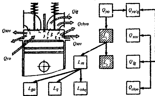
1.7-rasm. IYOD ning energetik balansi.
