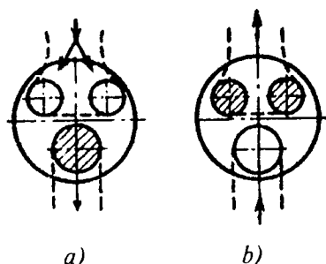
9.3-rasm. Bir silindrga uchta klapani joylashtirish varianti (a, b).
