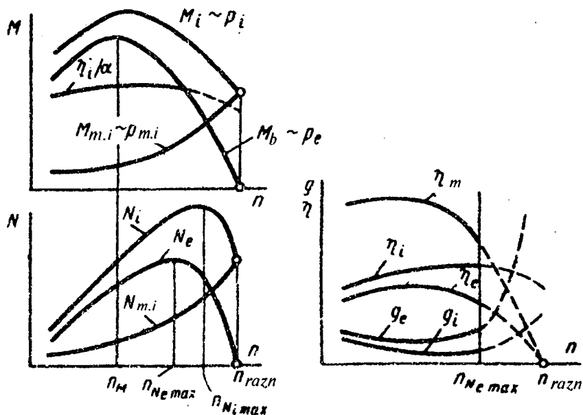
4.7-rasm. Dvigatelning indikator, samarali ko'rsatkichlarini va mexanik isrof bo'lishlarni xususiyatlaydigan parametrlarining aylanishlar chastotasiga bog'liqligi.
