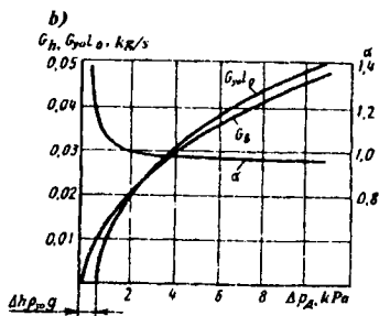
5.2-rasm. Oddiy karbyuratorning sxemasi (a) va tavsifi (b).
