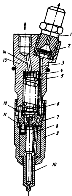
5.21-rasm. Prujina bilan berkitiladigan bekik forsunkaning konstruksiyasi:
