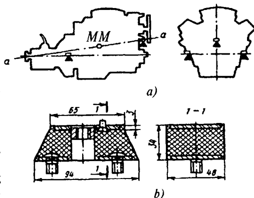
2.25-rasm. Avtomobil dvigateli osmasining sxemasi (a) va elastik elementi konstruksiyasining varianti (b).
