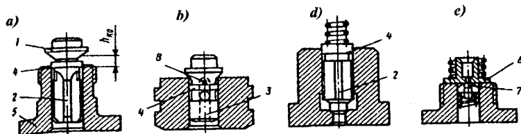
5.17-rasm. Haydovchi klapanlarning konstruksiyalari:
