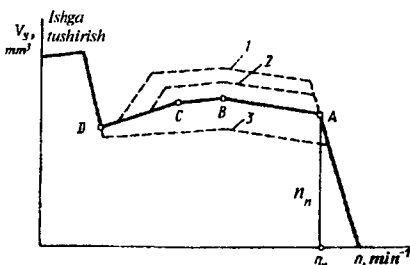
5.26-rasm. Yonilg'i uzatishning tashqi tezlik tavsifini tuzatish.
