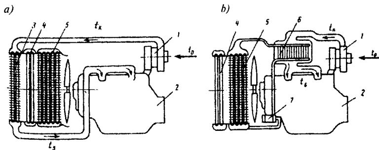
5.32-rasm. Havoni sovitish tizimlari:
