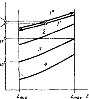
5.44 rasm. Barcha rejimli rostlagichning statik tavsifi.
