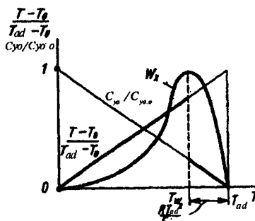
3.11-rasm. Cheklangan miqdordagi aralashmaning yonish tugashida yonilg'ining nisbiy konsentratsiyasi, kimyoviy reaksiyaning nisbiy harorati va tezligini o'zgarishi.
