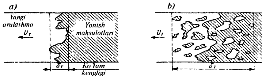
3.12-rasm. Alanga tarqalishining pulsatsiyali tezligini me'yoriy tezlikka nisbati kam (a) va ko'p (b) bo'lgandagi turbulent alanga ko'lamining sxemasi.
