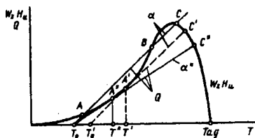
3.15-rasm. Kimyoviy reaksiyada issiqlik ajralib chiqish va turli haroratda issiqlik olish tezligini taqqoslash (alangananishni tahliliga).
