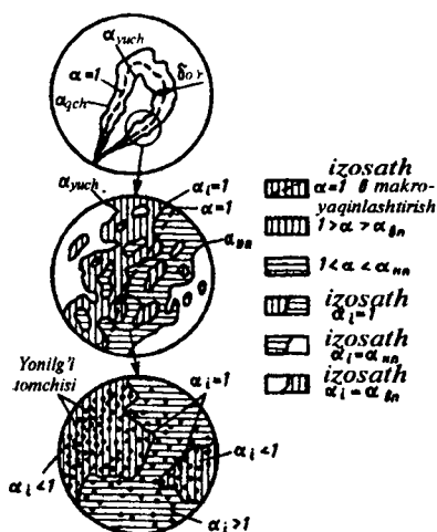
3.14-rasm. Yonilg'i oqimini turli darajada tahlil qilinishida uni tuzilishi ( \alpha_{yuch} va \alpha_{gch} yonishni yuqori va quyi konsentration chegarasiga mos keladigan havoning ortiqlik koeffitsiyenti).
