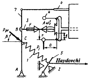
5.42-rasm. Bevosita ta'sir etuvchi barcha rejimli mexanikaviy rostlagich sxemasi:
