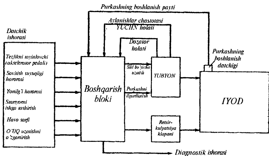
7.27.-rasm. Dizelni mikroprotessorli boshqarish majmuasi tizimining blok-sxemasi.
