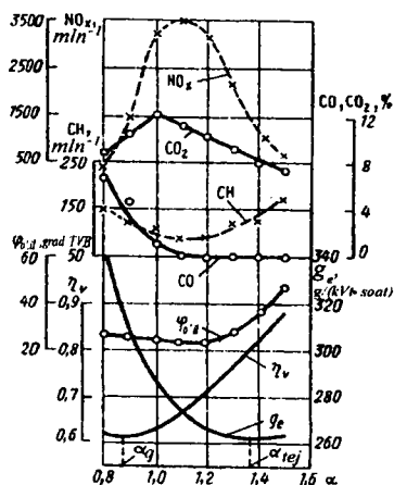
7.2-rasm. Quvvatning doimiyligida aralashma tarkibi bo'yicha rostlash tavsifi:
