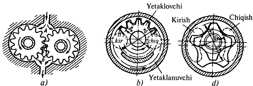
10.10-rasm. Tashqi – a va ichki (evolventli – b , episikloidali – d ) ilashmali moy nasoslari.
