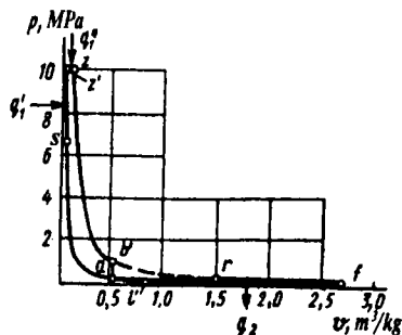
2.12-rasm. Kombinirlangan dvigatellarning sikllari: az'zb'f'l' — turbina oldidagi bosim o'zgaruvchan bo'lganda; az'zb'arf'l' — turbina oldidagi bosim o'zgarmas bo'lganda.
