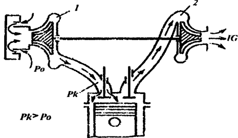
1.10-rasm. Gazturbina orqali qo'shimcha havo kiritish sxemasi.
