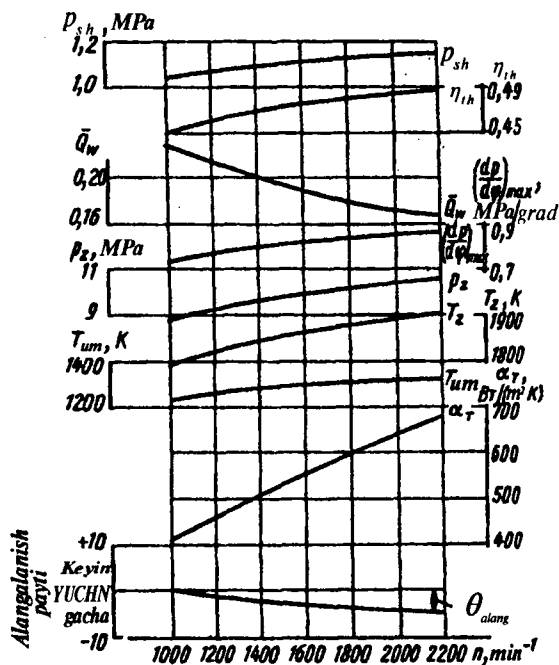
2.17-rasm. Hisoblangan siklning ko'rsatkichlarini aylanishlar chastotasiga bog'liqlik grafiqi.
