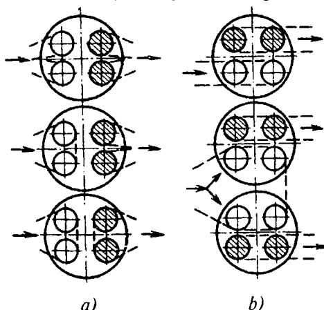
9.4-rasm. Bir silindrdagi to'rt klapaning joylashish variantlari (a, b).
