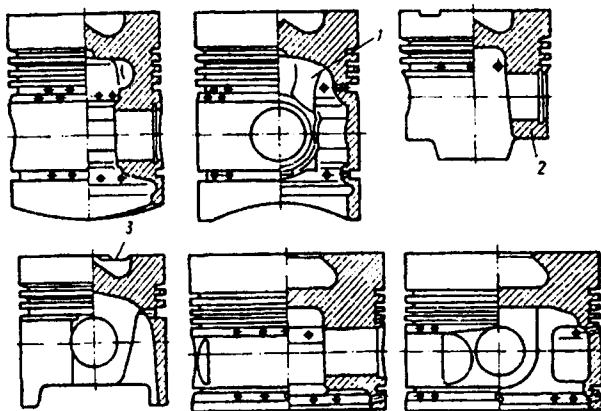
5.2-rasm. Dizellar porshenlarining konstruksiyasi:
