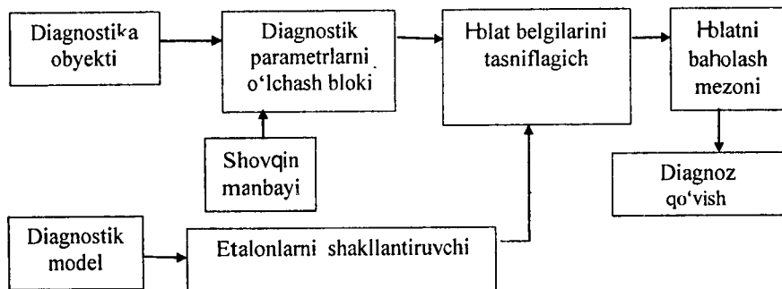
15.1-rasm. Dvigatellarni diagnostikalash tizimlarining tarkibiy sxemasi.
