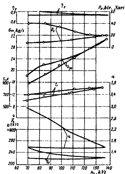
7.15-rasm. Bosimsiz kiritiladigan dizelning rostlagich tavsifi.
