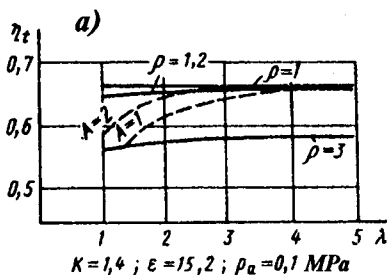
2.8-rasm. Sabate-Trinklar termodinamik sikli ko'rsatkichlarini bosimning ortish darajasiga bog'liqlik chiziqli tasviri:
