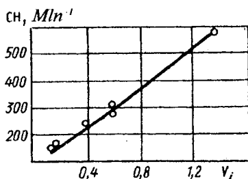
6.12-rasm. Yonish kamerasi porshenda joylashgan dizellarning IG dagi CH miqdoriga to'zitkichning igna osti hajmining ta'siri.
