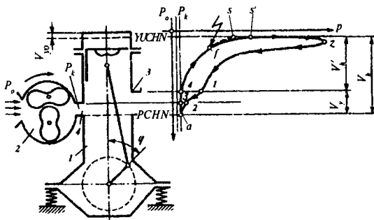
1.6-rasm. Ikki taktli dvigatelning sxemasi va indikator diagrammasi.
