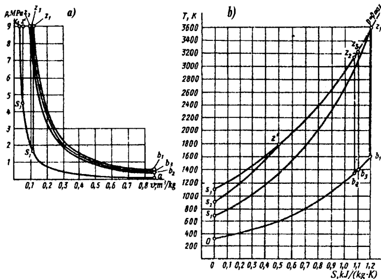
2.10-rasm. Otto, Dizel va Sabate-Trinkler sikllarini q , p = \text{idem} bo'lganda p - V (a) va T - s (b) koordinatalarda taqqoslash grafiqi.
