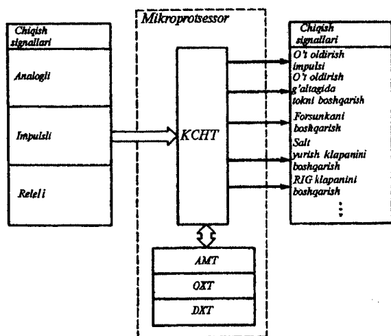
7.24-rasm. Uchqundan o't oldiriladigan dvigatelni mikroprotsessorli boshqarish majmuasi bloking tarkibi.
