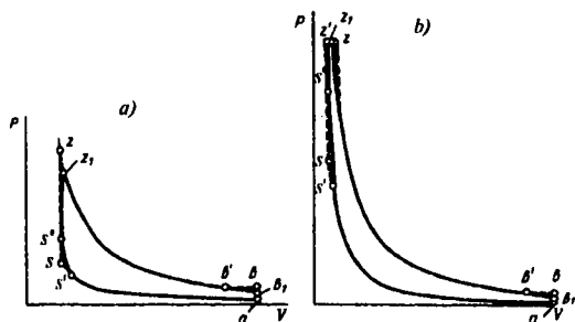
3.43-rasm. Uchqundan o't oldiriladigan dvigatel (a) va dizelning (b) siqish-kengayish diagrammasi.
