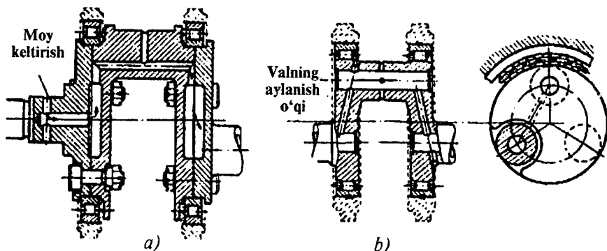
7.3-rasm. Yumalash podshipniklariga tarkibiy (a) va monolit (b) tirsakli valni o'rnatish.
