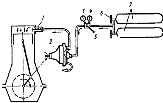
14.3-rasm. Siqilgan havo bilan ishga tushirish sxemasi.
