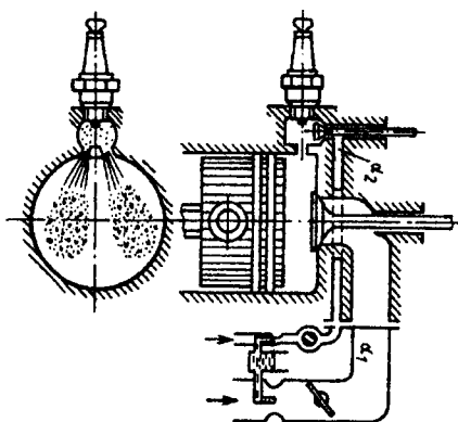
3.26-rasm. Forkamera-mash'alli o't oldiriladigan karbyuratorli dvigatelning sxemasi.
