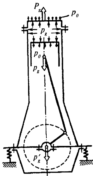
1.6-rasm. KSHM konstruksiya qismlariga gazlar kuchining ta'siri.
