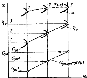
7.4-rasm. G_{yo} = \text{const} bo'lganda aralashmaning tarkibi bo'yicha rostlash tavsifi.
