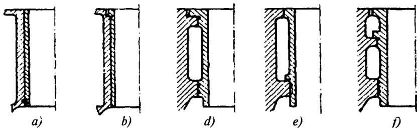
4.3-rasm. Silindrlar gilzalarining asosiy turlari:
