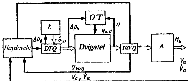
7.23-rasm. Uchqundan o't oldiriladigan dvigatelni avtomobilda boshqarish sxemasi.
