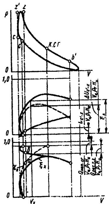
3.42-rasm. Dvigatelning ichki issiqlik balansi.
