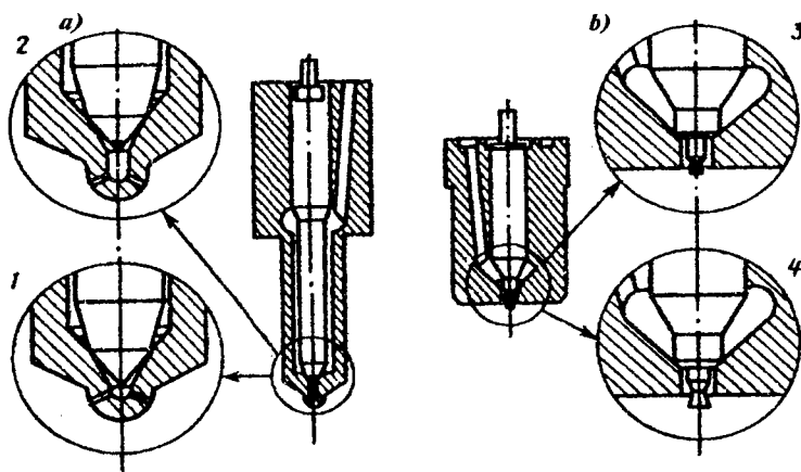
5.22-rasm. Berk forsunkalarning to'zitkichlari: a — ko'p oqimli; b — shtiftli.
