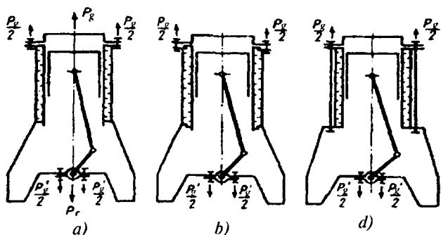
4.1-rasm. Suyuqlik bilan sovitiladigan IYOD kuch sxemalari: a – silindrlar bloki yuk ko'taruvchi; b – g'ilof yuk ko'taruvchi; d – kuch shpilka yuk ko'taruvchi.
