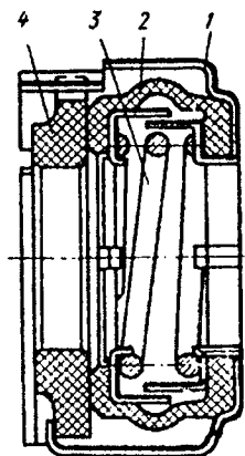
11.13-rasm. Suyuqlik nasosining zichlagichi.
