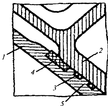
4.4-rasm. Gilzani quyi belbog'da zichlash:
