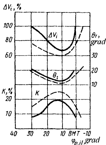
6.13-rasm. Yonish kamerasi porshenda joylashgan dizellarning IG ning tutab chiqishiga ( \varphi_{p,il} ) ni ta'siri:
