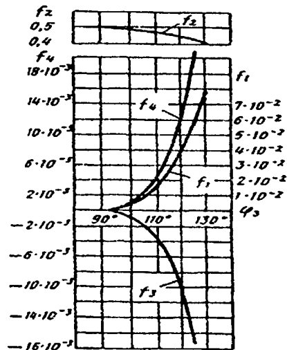
6.8-rasm. Eguvchi moment M va normal kuch N ning bekilish burchagiga bog'liqligini aniqlash uchun yordamchi diagramma.
