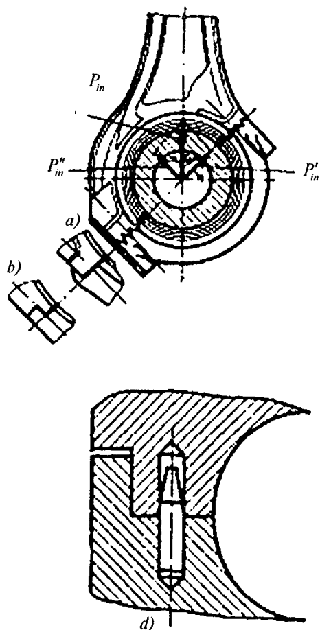
6.5-rasm. Uchburchak shlitsalar (a), bo'rtiqlar (b) ko'rinishidagi qiya ajratkichli va (d) shtift bilan qaydlanuvchi tekis tutash sathli shatunning krivoship kallagi.
