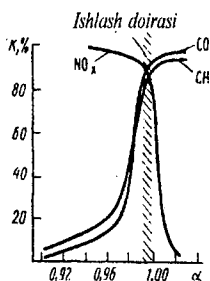
6.8-rasm. Uch tashkil etuvchili neytrallagichning samarali ishlash doirasi.
