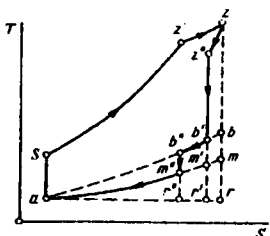
2.25-rasm. T—S koordinatalarda issiqlik aralash usulda beriladigan sikl.
