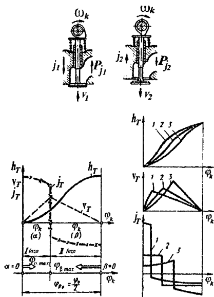
9.23-rasm. Qavariq (1), botiq (2) va tangensial (3) profilli turtkichlarning bir xil ko'tarilishida va burchak ta'sirida kinematik parametrlarini taqqoslash.
