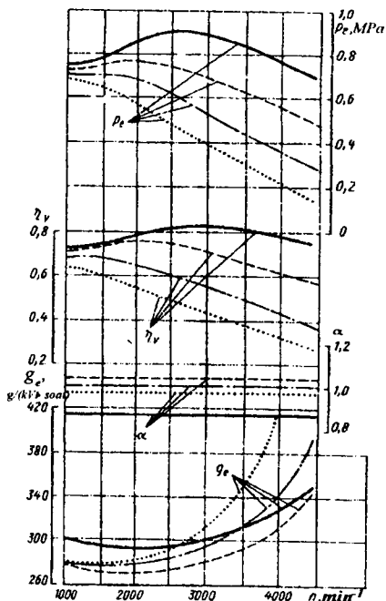
7.13-rasm. V8 karbyuratorli dvigatelning tashqi va qisman tezlik tavsiflari
