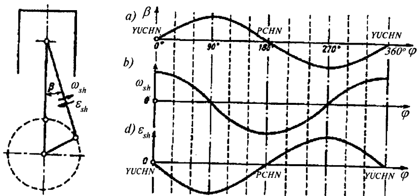
1.4-rasm. Shatunning kinematik parametrlari:
