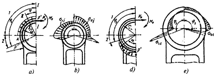
6.7-rasm. Porshen kallagida yuklamalarning taqsimlanishi va tashqi hamda ichki sathlarda kuchlanishlar epyuralari: a – cho‘zilishda yuklamaning taqsimlanish sxemasi; b – cho‘zilishda kuchlanishlar epyuri; d – siqishda yuklamaning taqsimlanish sxemasi; e – siqishda kuchlanishlar epyuri.
