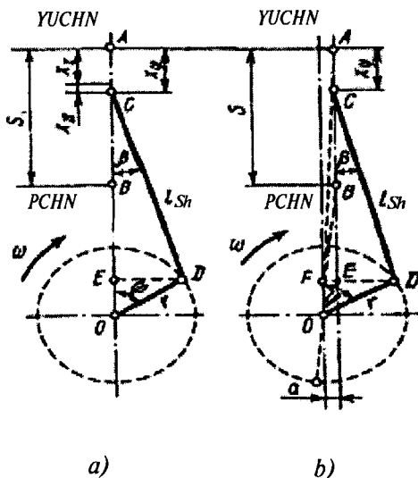
1.2-rasm. KSHM ni hisoblash sxemalari: a – markaziy; b – siljirilgan.
