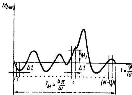
8.6-rasm. «Motor» massaga ta'sir qiluvchi burovchi momentning garmonik tahlili.
