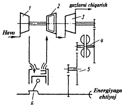
2.11-rasm. Kombinirlangan dvigatelning sxemasi:
