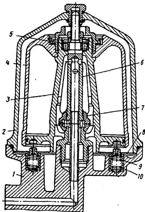
10.12-rasm. YAMZ-840 dvigateli sentrifugasining konstruksiyasi:
