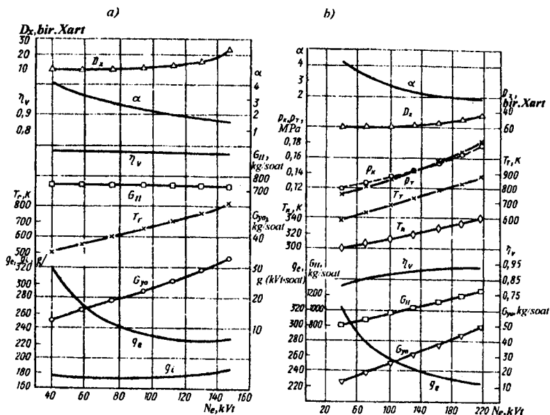
3.10-rasm. Dizelnin yuklama tavsifi:
