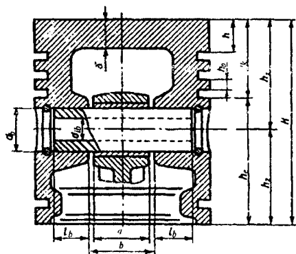
5.5-rasm. Porshen guruhi konstruktiv elementlari parametrlari.
