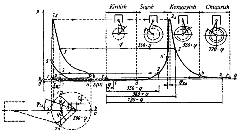
1.5-rasm. Indikator diagrammani p-V dan p-\varphi koordinatasida qayta qurish.
