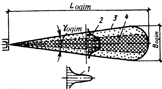
3.30-rasm. To'zitilgan yonilg'i oqimining sxemasi.
