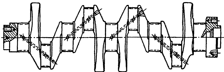
7.1-rasm. Po'latdan tayyorlangan tirsakli val.
