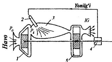
1.2-rasm. Bir valli gazyurtinalli dvigatelning sxemasi:
