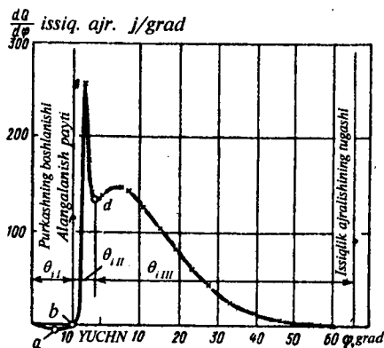
3.40-rasm. Dizelda issiqlik ajralib chiqish tezligining tavsifi.
