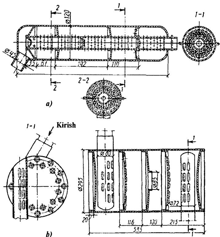
13.2-rasm. Yengil avtomobil (a) va avtobusning (b) chiqarish shovqinini so'ndirgichlar.
