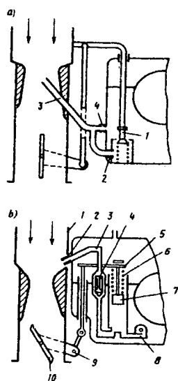
5.5.-rasm. Ekonomayzer (a) va tezlatish nasosining sxemasi (b).
