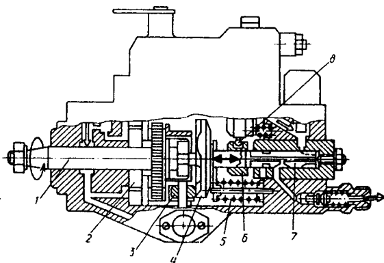
5.18-rasm. Bir plunjerli taqsimlash nasosi.
