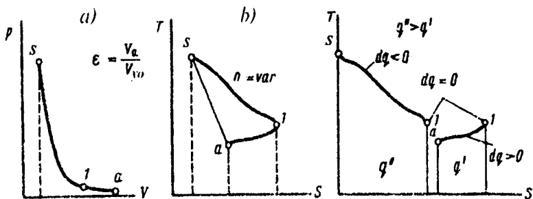
3.9-rasm. Siqish jarayoni:
