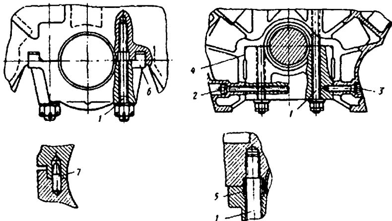
4.5-rasm. Tirsakli val o'zak podshipniklarining qopqoqlarini mahkamlash:
