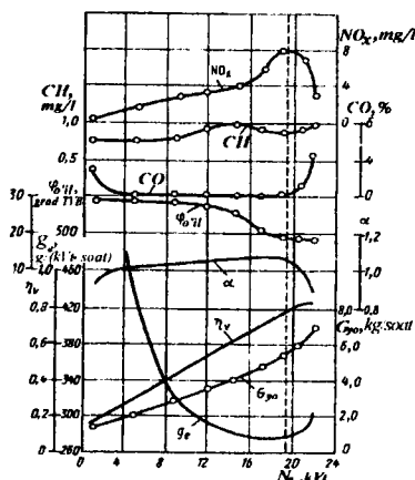
7.8.-rasm. Karbyuratorli dvigatelnining yuklama tavsifi:
