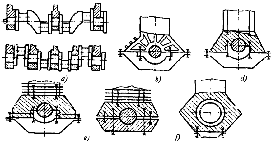
4.2-rasm. Blok-karterning bikrliligini oʻrtirish boʻyicha asosiy konstruktiv tadbirlar: a – toʻliqsiz tayanchli tirsakli valdan toʻliq tayanchlilikka oʻtish; b – oxirgi tayanch toʻsiqlarini va yon devorlarini qovurgʻalash; d – karter ajratkichi tekisligini pastga tushirish; e – tunnelli karter; f – oʻzak tayanch bilan birlashtirilgan ramali plita yoki moy togʻoraning qutisimon konstruksiyasi.
