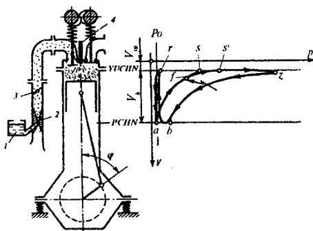
1.3-rasm. Karbyuratorli dvigatelning sxemasi va indikator diagrammasi:
