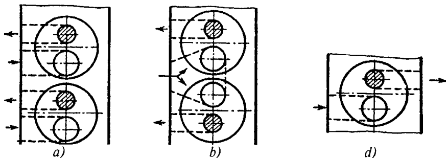
9.1-rasm. Bir silindrda ikki klapanli bir jinslilik qilib joylashtirish: a, d—kiritish va chiqarish klapanlari almashinadi; b—juft joylashishi.
