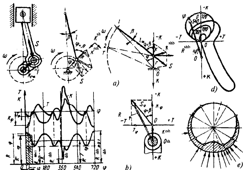
1.10-rasm. Shatun bo'ynini yuklantiradigan kuchlarni hisoblashga:
