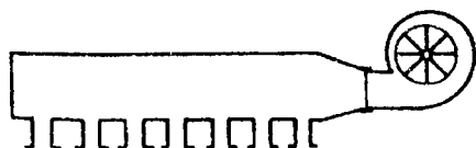
5.29-rasm. Bosim ostida kiritishning izobar tizimi.
