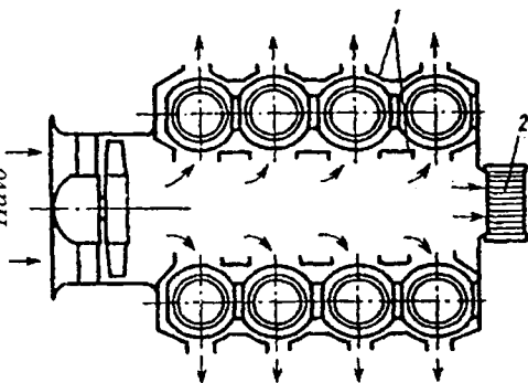
11.18-rasm. Havo bilan sovitiladigan dvigatelda havoning aylanma harakatini tashkil etish sxemasi: 1 – deflektorlar; 2 – moy radiatori.
