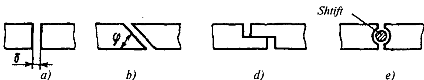
5.18-rasm. Halqalar qulflarining shakllari: a – toʻgʻri burchakli; b – qiya; d – pogʻonali; e – ikki taktili dvigatel uchun shtiftli.
