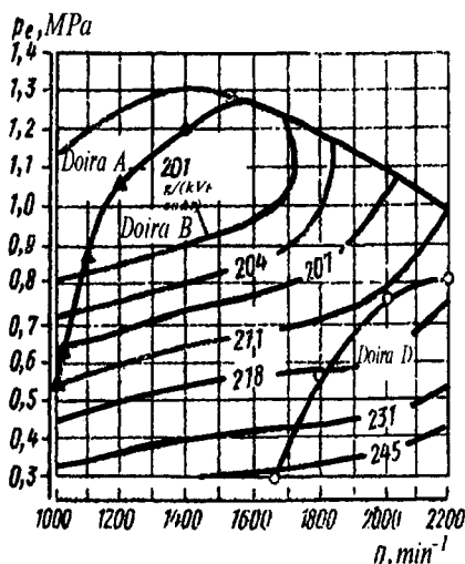
7.18-rasm. Kombinirlangan bosim ostida kiritish va turbinani chetlab gazlarni o'tkazib yuborish boshqariladigan dizelning ko'p parametrlil tavsifi: A doira-yurituvchi haydovchi ulangan; B doira-yurituvchi haydovchi uzib qo'yilgan; D doira-yurituvchi haydovchi uzib qo'yilgan va klapanlar ochiq.
