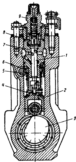
5.16-rasm. Yuqori bosimli ko'p plunjerli yonilg'i nasosi.
