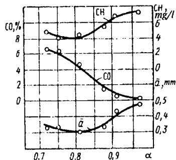
6.7-rasm. \alpha ga bog'liq holda IG tarkibini va osmada dvigatel titrash
