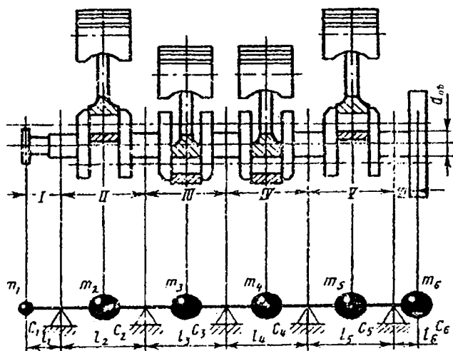
8.13-rasm. Tirsakli valning egilish tebranishlari- ning tahlili uchun ekvivalent sxema.
