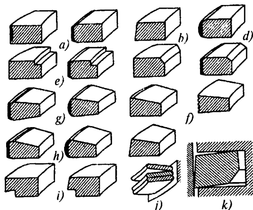
5.15-rasm. Birinchi kompression halqalarning asosiy konstruktiv yechimlari:
