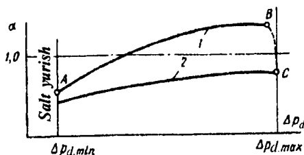
5.3-rasm. Aralashma tarkiblarida karbyuratorning eng qulay tavsifi: 1 — tejamkor; 2 — quvvatli.
