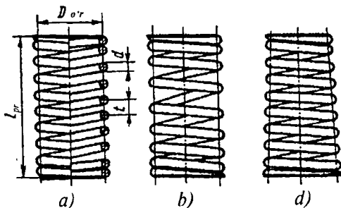
9.14-rasm. O'ramlar qadami doimiy (a) va o'zgaruvchan (b) bo'lgan klapan prujinalari; (d) konussimon prujina.
