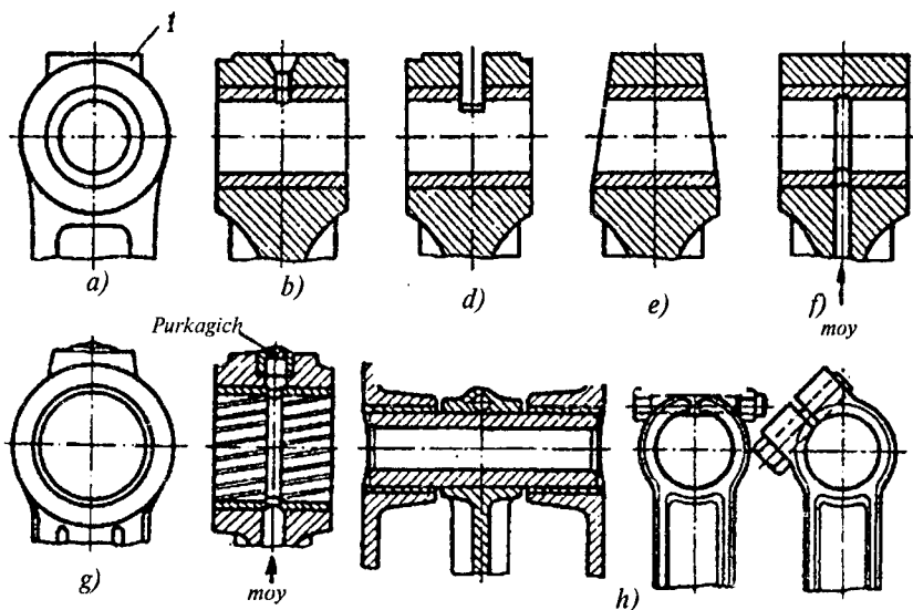
6.3-rasm. Shatunlarning porshen kallaklari:
