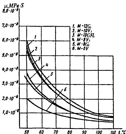
10.6-rasm. Motor moylari qovushqoqligining haroratga bog'liqlik grafigi.
