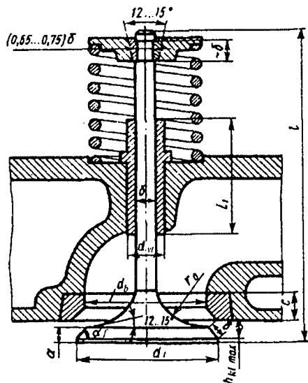
9.19-rasm. Klapan mexanizmining konstruktiv nisbatlari:
