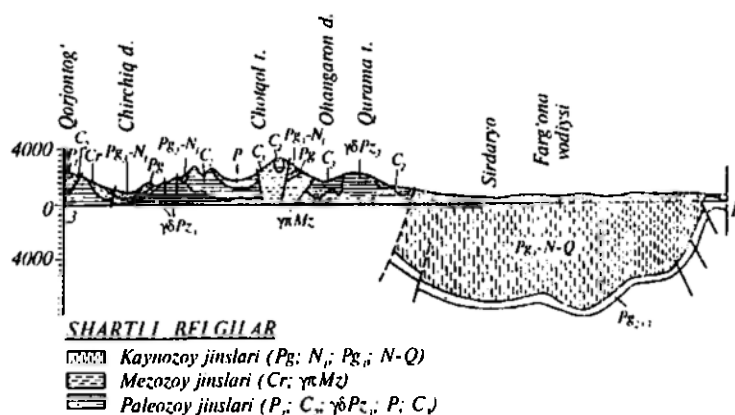
2-rasm. G'azalkent bilan Vodil orqali o'tkazilgan geologik profil.
