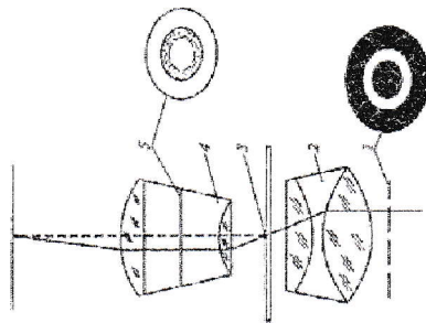
15-rasm. Fazo-kontrast moslama ishlatishda nurlarning o'tish sxemasi: 1-halqasimon diafragma; 2-kondensor; 3-obyekt; 4-obyektiv; 5-fazaviy plastinka.
