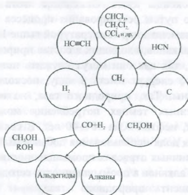
Рис. 3.2. Использование метана как сырья для химической промышленности
