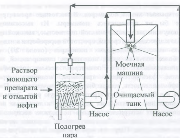
Рис. 6.2. Схема очистки нефтеналивных танков
