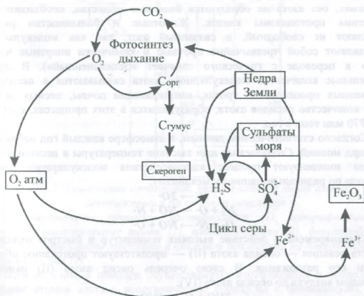
Рис. 2.1. Некоторые важнейшие элементы глобального цикла кислорода
