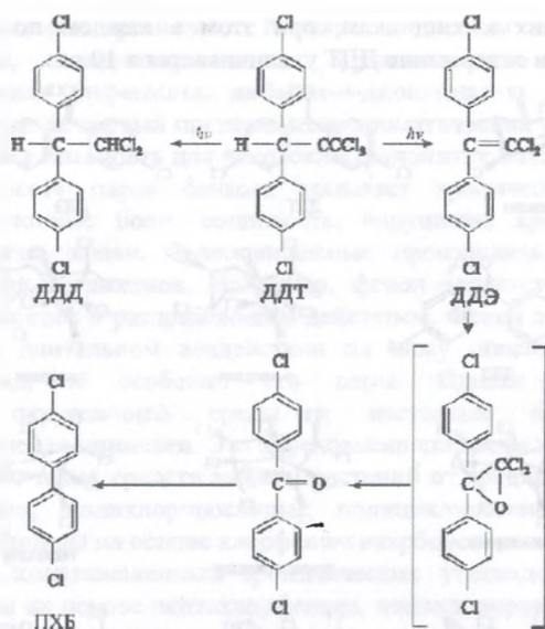
Рис.6.4. Превращения ДДТ под действием света
