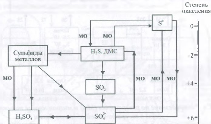
Рис.2.5. Химические соединения, участвующие в цикле серы МО — процессы, осуществляемые микроорганизмами, ДМС — диметилсульфид \text{CH}_3\text{SCH}_3
