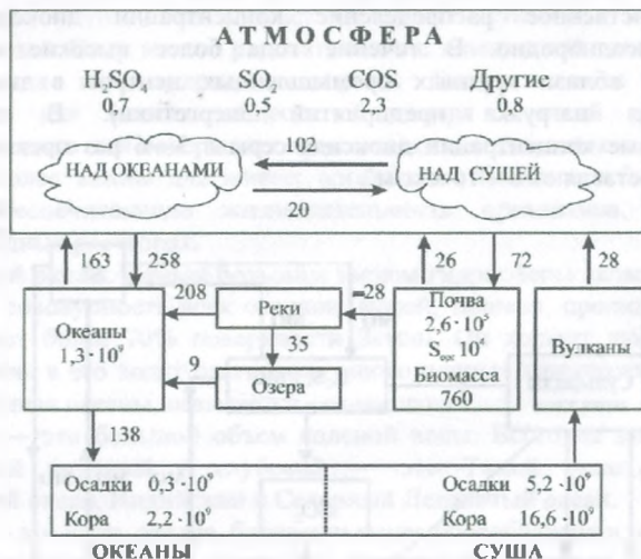
Рис. 2.4. Распределение по резервуарам (Мт) и миграционные потоки (Мт/год) серы в географической оболочке Земли
