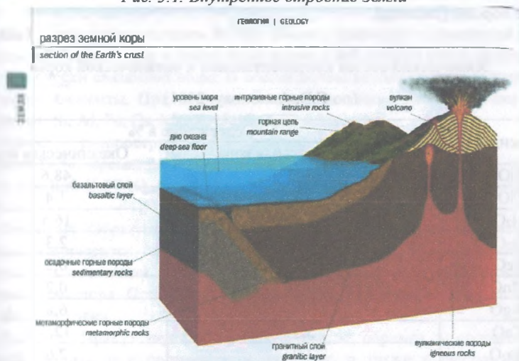
Рис. 5.2. Типы земной коры (по М.В. Муратову): 1- вода; 2 - осадочный слой; 3 - гранитный слой; 4 - базальтовый слой; 5 - мантия Земли; 6 - участки мантии,
