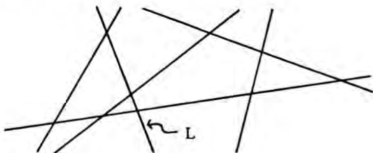
Рис. 3.6. Множество линий
