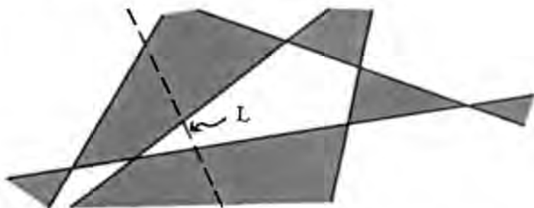
Рис. 3.7. Раскрашено в соответствии с наличием m линий
