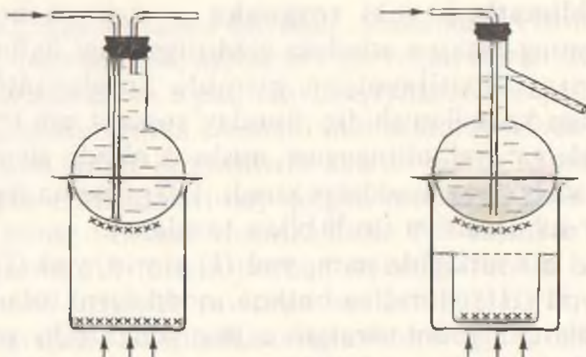
15-rasm. Moddalarni sublimatlash yo'li bilan tozalash.
