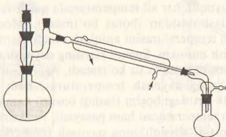
18-rasm. Vakuumdagi haydash asbobi.
