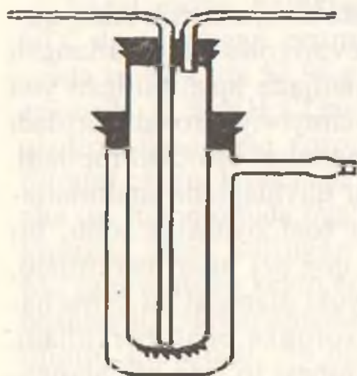
16-rasm. Vakuumda sublimatsiya qilish asbobi.
