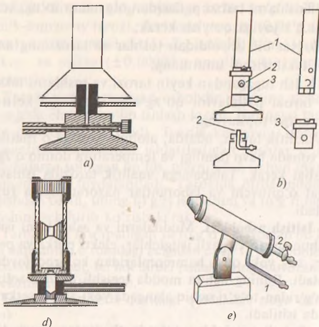
3-rasm. Gaz isitgichlari:
