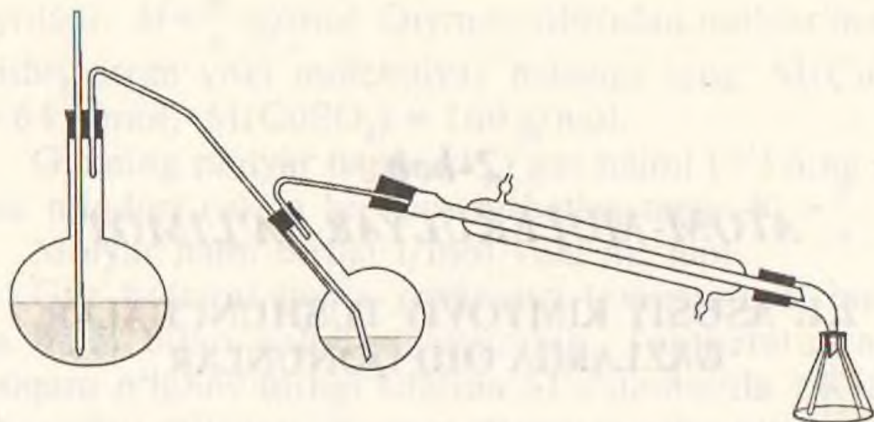
19-rasm. Suv bug'i bilan haydash asbobi.
