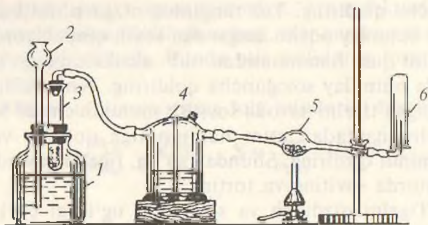
24-rasm. Oksid tarkibini aniqlash asbobi.
