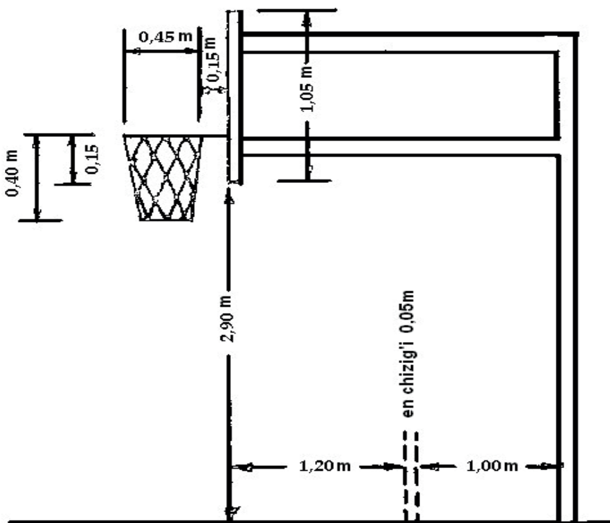
1-rasm. Halqa shit qurilmasi.
