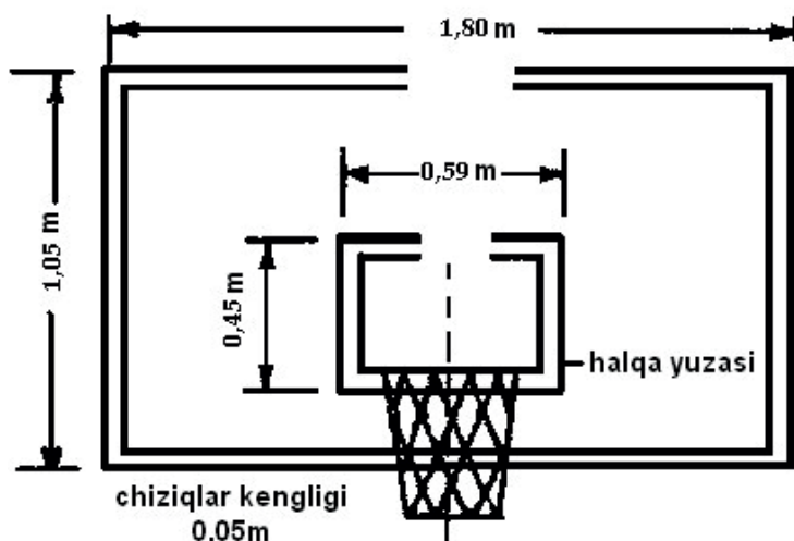
2-rasm. Shit. Uning o'lchovlari.
