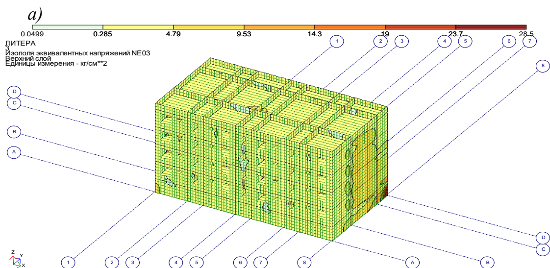
Рис.11. Изополя эквивалентных напряжений при упругом взаимодействии фундамента с грунтом основания и низкочастотных колебаниях: (a) в пространственном виде.
