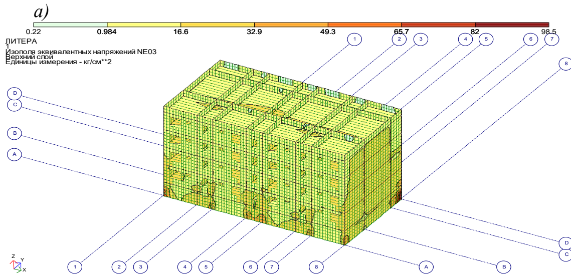
Рис.9. Изополю эквивалентных напряжений при жестком защемлении фундамента с грунтом основания и низкочастотных колебаниях: (a) в пространственном виде.
