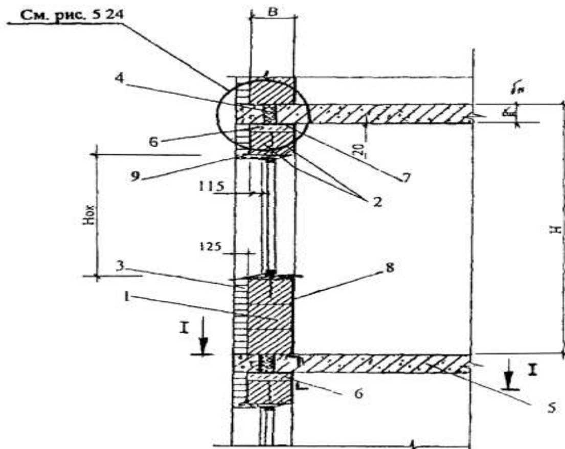
2-расм. Ғиштли, фасад облицовкали юк кўтаришга мўлжалланмаган деворнинг вертикал кесими.
