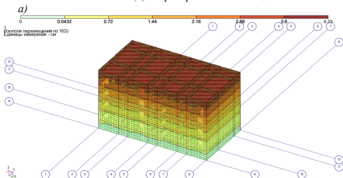
Рис.14. Изополю линейного перемещения по Y при жестком защемлении фундамента с грунтом основания и высокочастотных колебаниях: (a) в пространственном виде.
