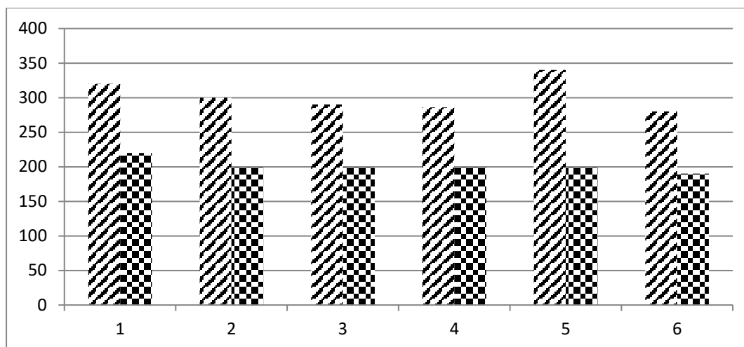
1-расм. Иккиламчи материал ресурслар миқдори турлича бўлган тўқималарнинг танда ва ароқоқ бўйича зичлигининг ўзгариши.
