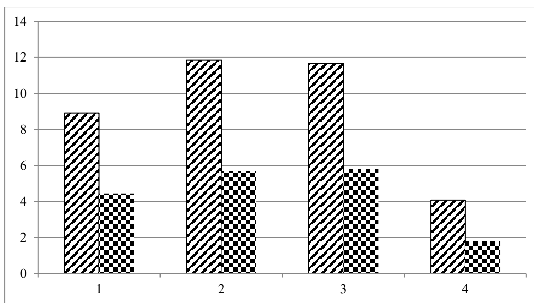
Аралашмали ип ▨ 1 m даги; ▣-10 m даги. 2-расм. Тола таркиби турлича бўлган ипларнинг 1 m ва 10 m даги вариация коэффициентининг ўзгариши.
