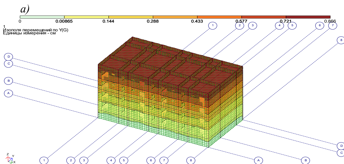
Рис.12. Изополя линейного перемещения по Y при вязкоупругом взаимодействии фундамента с грунтом основания и низкочастотных колебаниях: (a) в пространственном виде.
