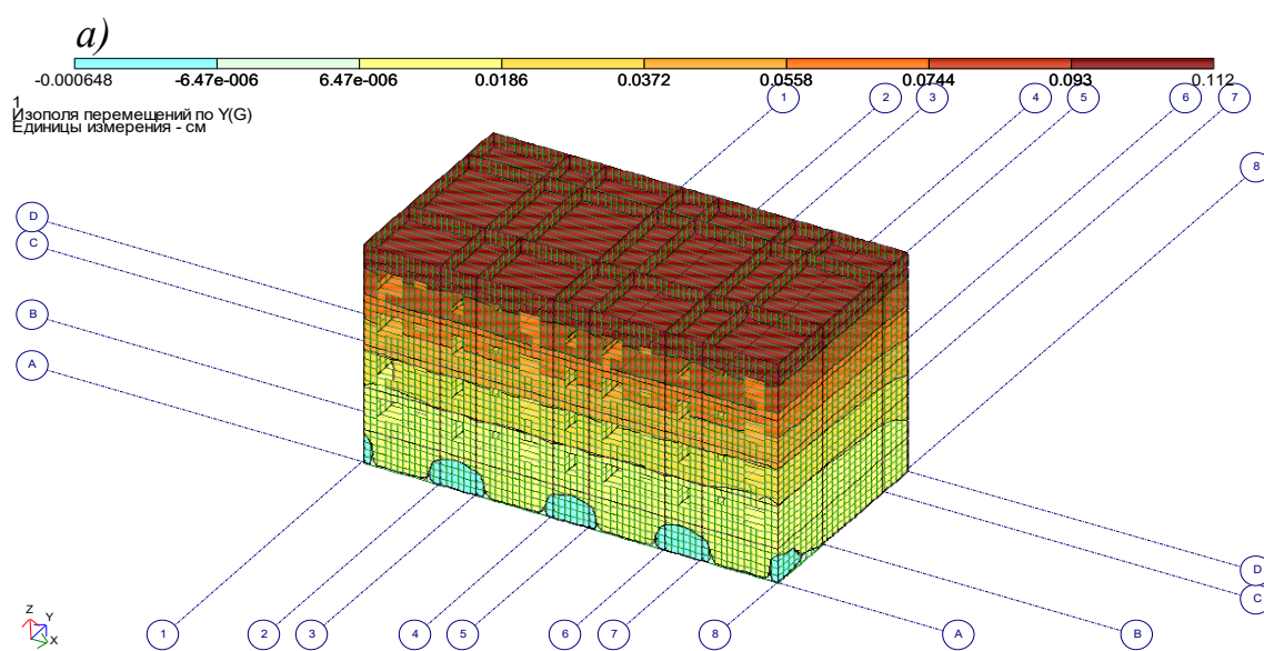
Рис.16. Изополю линейного перемещения по Y при упругом взаимодействии фундамента с грунтом основания и высокочастотных колебаниях: (a) в пространственном виде.
