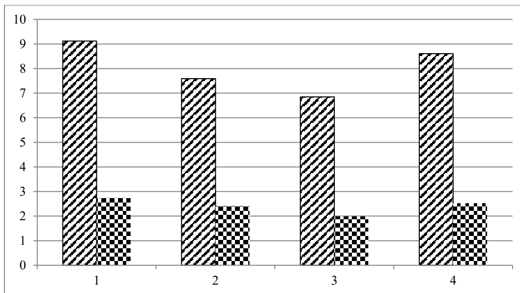
3-расм. Тола таркиби турлича бўлган ипларнинг тукдорлиги ва тукдорлиги бўйича квадратик нотекислигининг ўзгариши.
