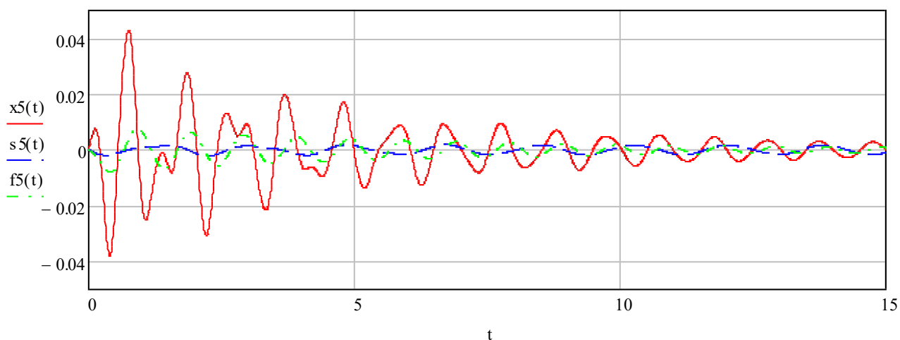
Рис.3. Перемещение последнего этажа здания при высокочастотных колебаниях: жесткое защемление фундамента x5(t) , упругое взаимодействие фундамента с грунтом s5(t) и вязкоупругое взаимодействие f5(t) , м
