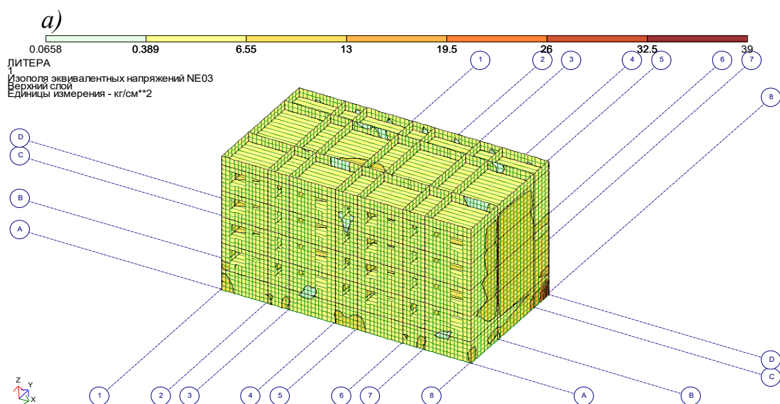
Рис.13. Изополю эквивалентных напряжений при вязкоупругом взаимодействии фундамента с грунтом основания и низкочастотных колебаниях: (a) в пространственном виде.
