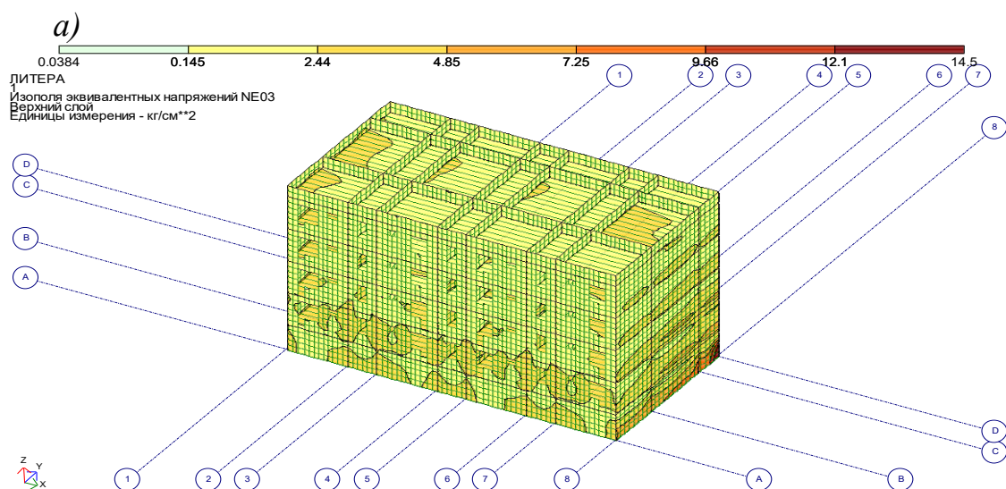
Рис.17. Изополю эквивалентных напряжений при упругом взаимодействии фундамента с грунтом основания и высокочастотных колебаниях: (a) в пространственном виде
