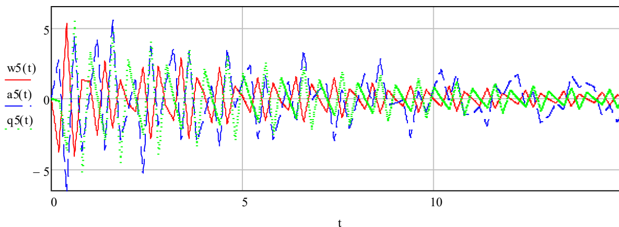
Рис.3. Ускорение последнего этажа здания при низкочастотных колебаниях: жесткое защемление фундамента w_5(t) , упругое взаимодействие фундамента с грунтом a_5(t) и вязкоупругое взаимодействие q_5(t) , \text{м/с}^2
