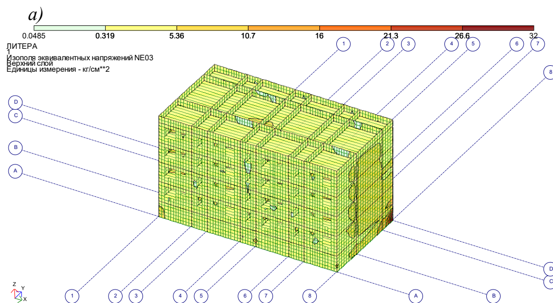
Рис.19. Изополю эквивалентных напряжений при вязкоупругом взаимодействии фундамента с грунтом основания и высокочастотных колебаниях: (а) в пространственном виде.
