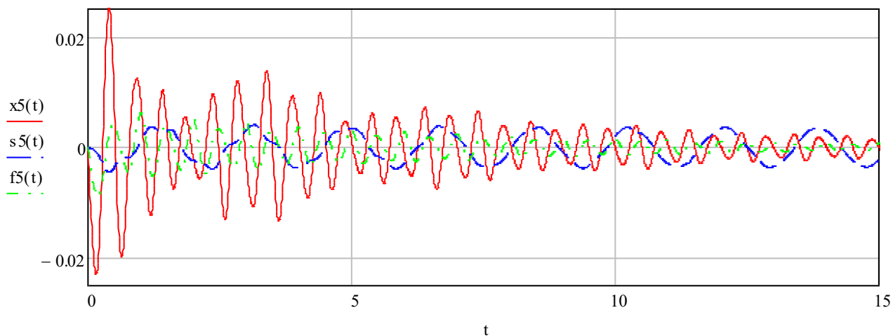
Рис.2. Перемещение последнего этажа здания при низкочастотных колебаниях: жесткое защемление фундамента x5(t) , упругое взаимодействие фундамента с грунтом s5(t) и вязкоупругое взаимодействие f5(t) , м
