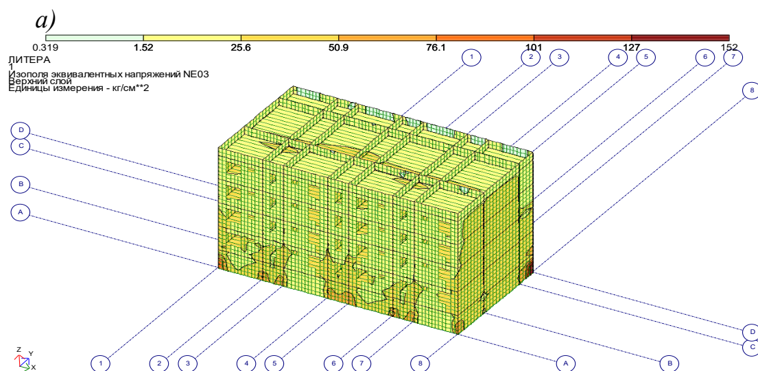
Рис.15. Изополю эквивалентных напряжений при жестком закреплении фундамента с грунтом основания и высокочастотных колебаниях: (a) в пространственном виде.
