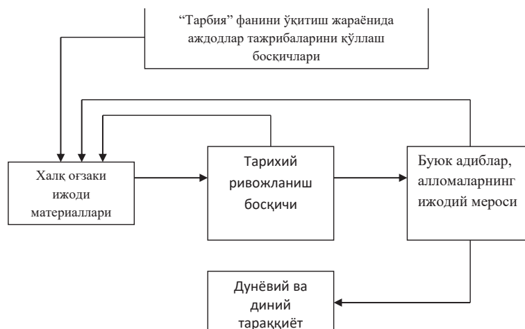
1.2-расм. “Тарбия” фанини ўқитиш жараёнида аждодлар тажрибаларини босқичлари
