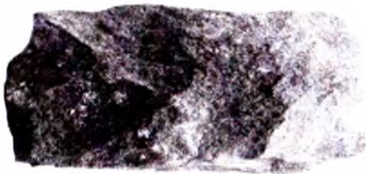
59- rasm. Kvarsit.
