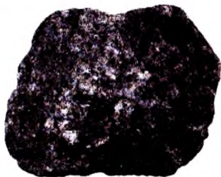
33- rasm. Granodiorit.
