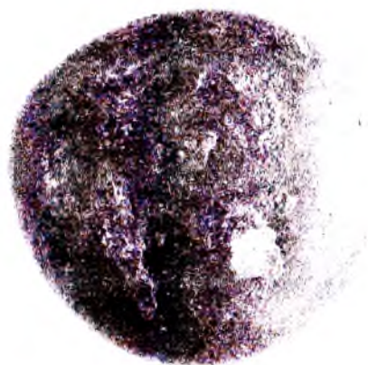
53- rasm. Fosforit.
