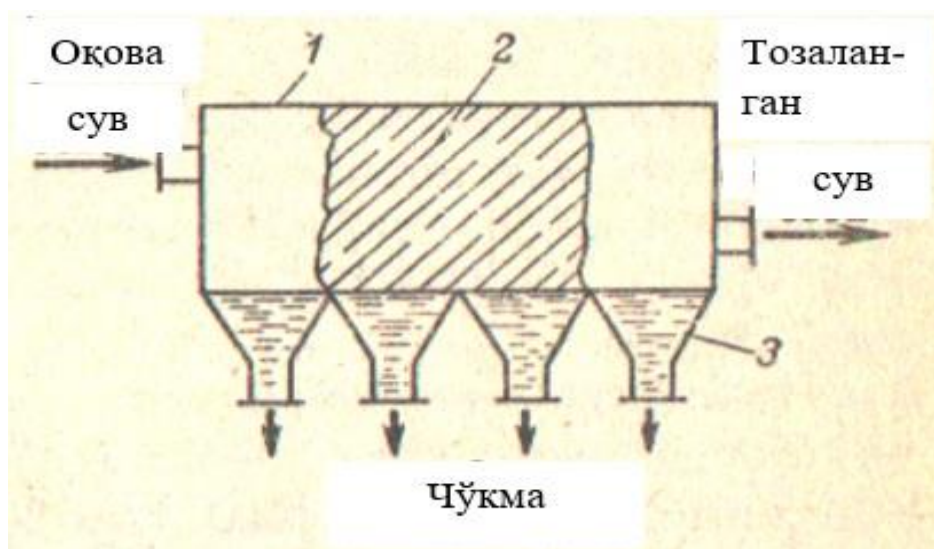
9.5-рasm. Пластиналари қия ўрнатилган тиндиргич: 1-корпус; 2-қия ўрнатилган пластиналар; 3-чўкмайиғичлар.
