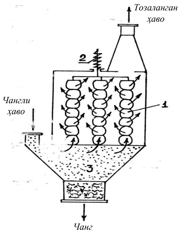
5.12-расм. Бир секцияли енгли филтрнинг кўриниши: 1- тўқимали (енгли) филтр; 2- енгларни силкитувчи мослама; 3- чанг йиғувчи бункер.
