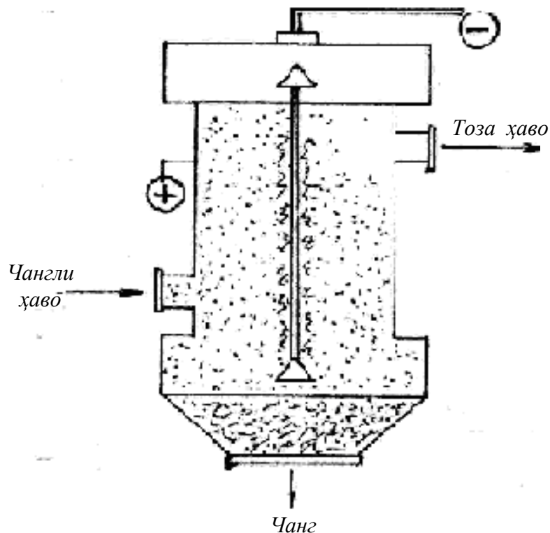
5.14-расм. Электр филтри.
