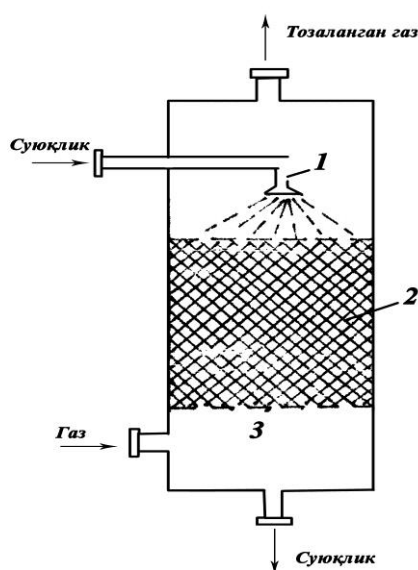
5.18- расм. Абсорбернинг кўриниши: 1- сувни пуркаб берувчи форсунка; 2- сув қатлами; 3- ўтказма.
