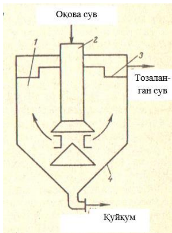
9.2-расм. Тик (вертикал) тиндиргич: 1-цилиндр қисми; 2-марказий қувур; 3-желоб; 4-конуссимон қисм.
