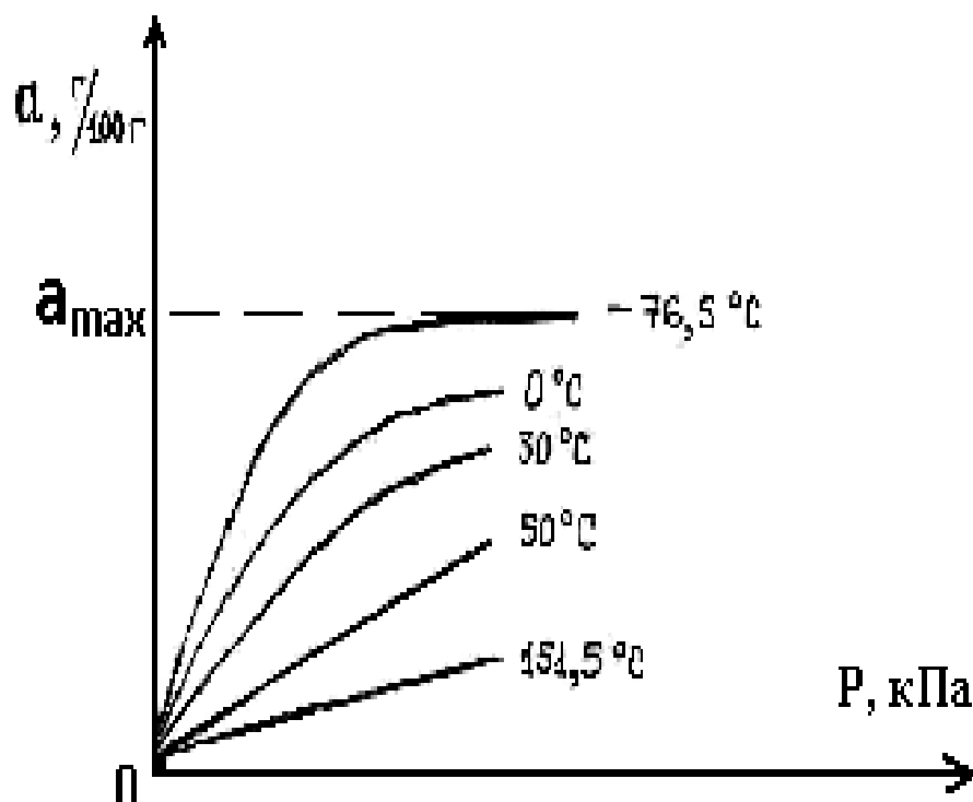
5.17 - расм. Фаоллаштирилган кўмирга углерод кўш оксидининг адсорбцияланиш изотермалари.
