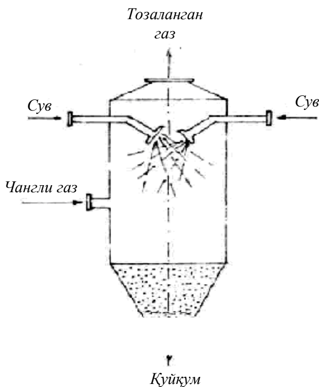
5.8-расм. Форсункали скруббер.
