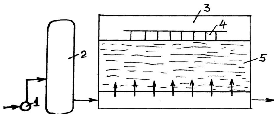
9.7 - расм. Флотацион қурилманинг кўриниши: 1-насос; 2-босимли бак; 3- кўпик йиғувчи механизм; 4 – кўпик йиғгич; 5-флотацион камера.
