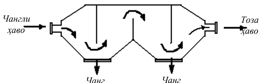
5.3-расм. Тўсиқли чанг чўктириш камераси.
